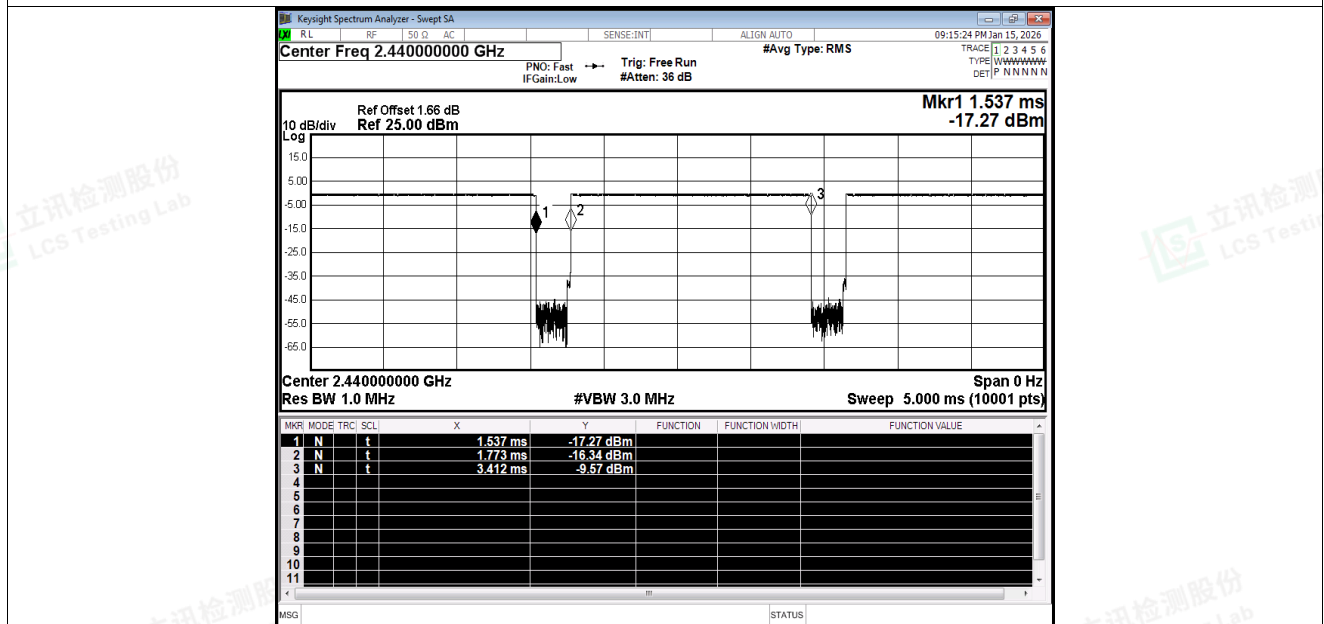
Duty Cycle NVNT BLE 1M 2440MHz Ant1
