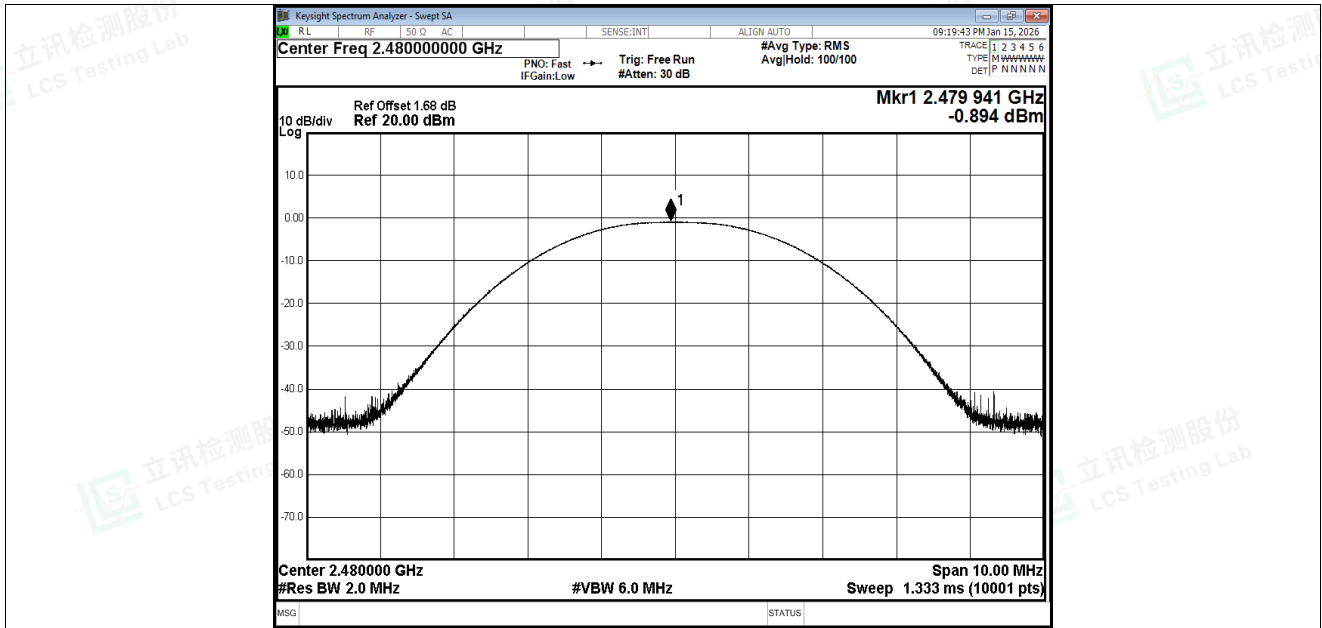
Peak Power NVNT BLE 1M 2480MHz Ant1
