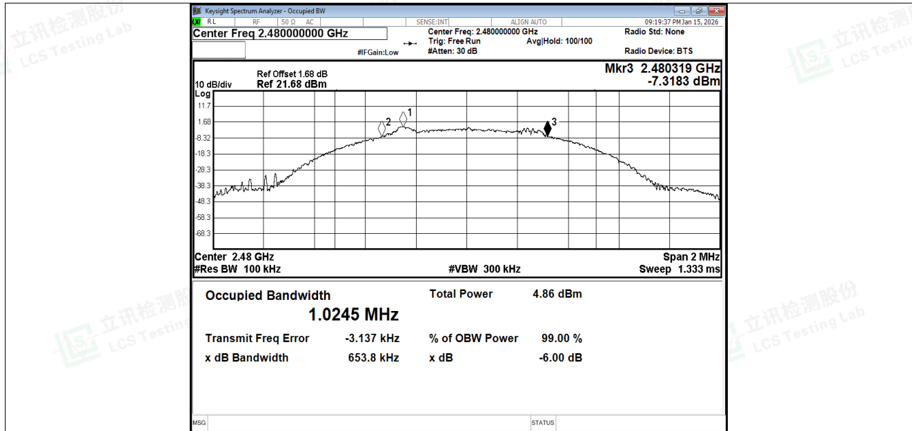
-6dB Bandwidth NVNT BLE 1M 2480MHz Ant1
