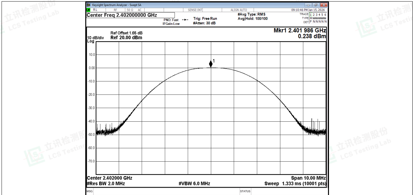
Peak Power NVNT BLE 1M 2402MHz Ant1
