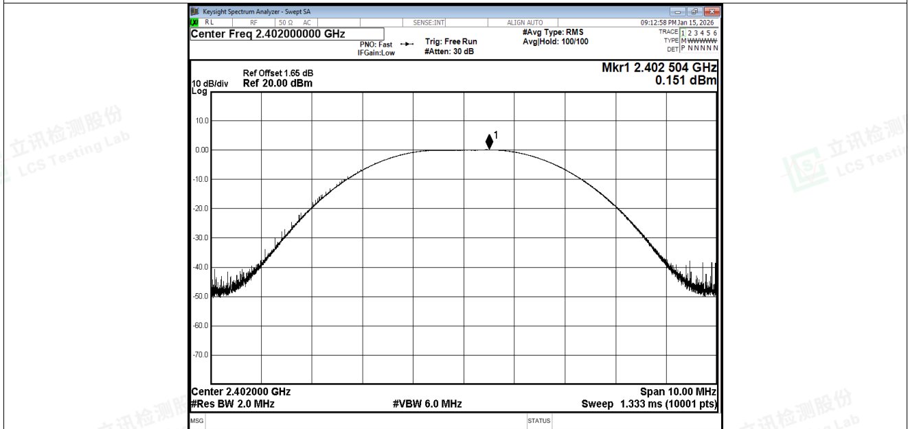
Peak Power NVNT BLE 2M 2402MHz Ant1
