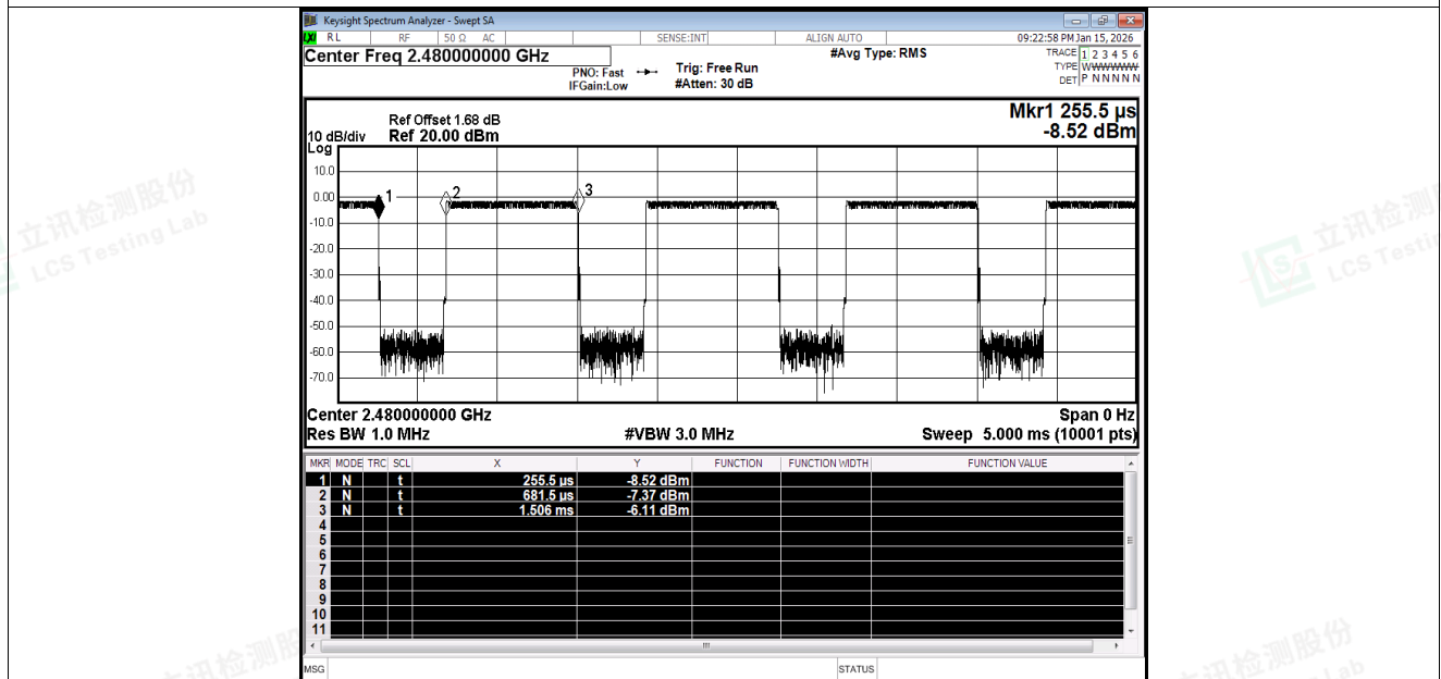
Duty Cycle NVNT BLE 2M 2480MHz Ant1
