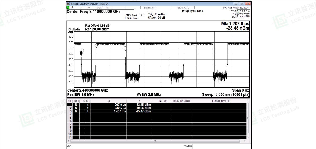
Duty Cycle NVNT BLE 2M 2440MHz Ant1
