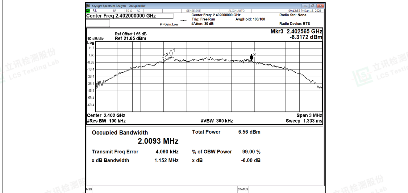
-6dB Bandwidth NVNT BLE 2M 2402MHz Ant1
