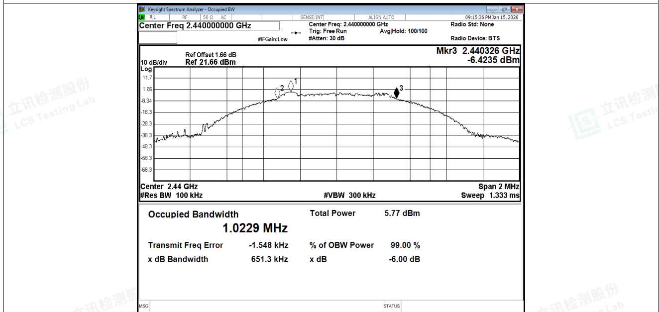
-6dB Bandwidth NVNT BLE 1M 2440MHz Ant1
