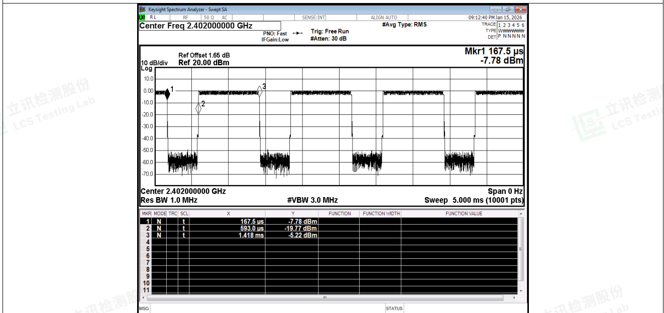
Duty Cycle NVNT BLE 2M 2402MHz Ant1
