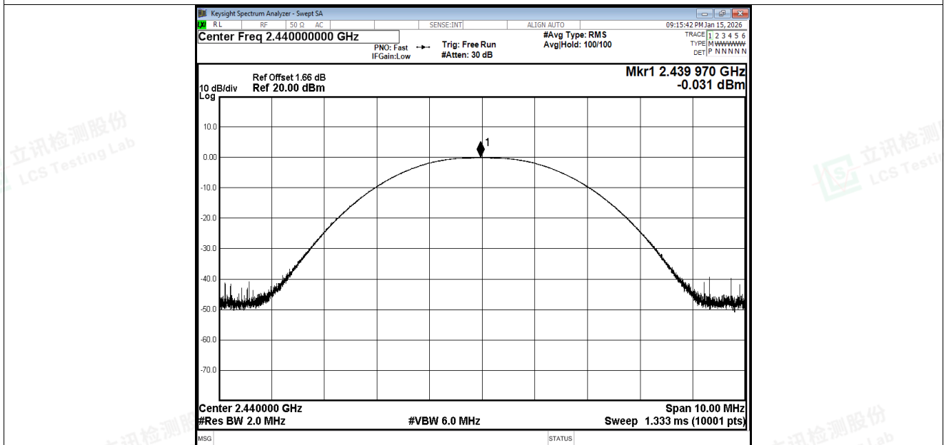
Peak Power NVNT BLE 1M 2440MHz Ant1
