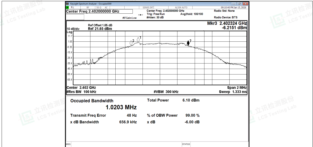
-6dB Bandwidth NVNT BLE 1M 2402MHz Ant1
