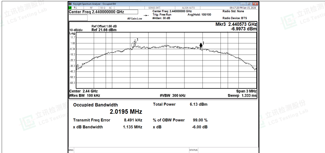
-6dB Bandwidth NVNT BLE 2M 2440MHz Ant1
