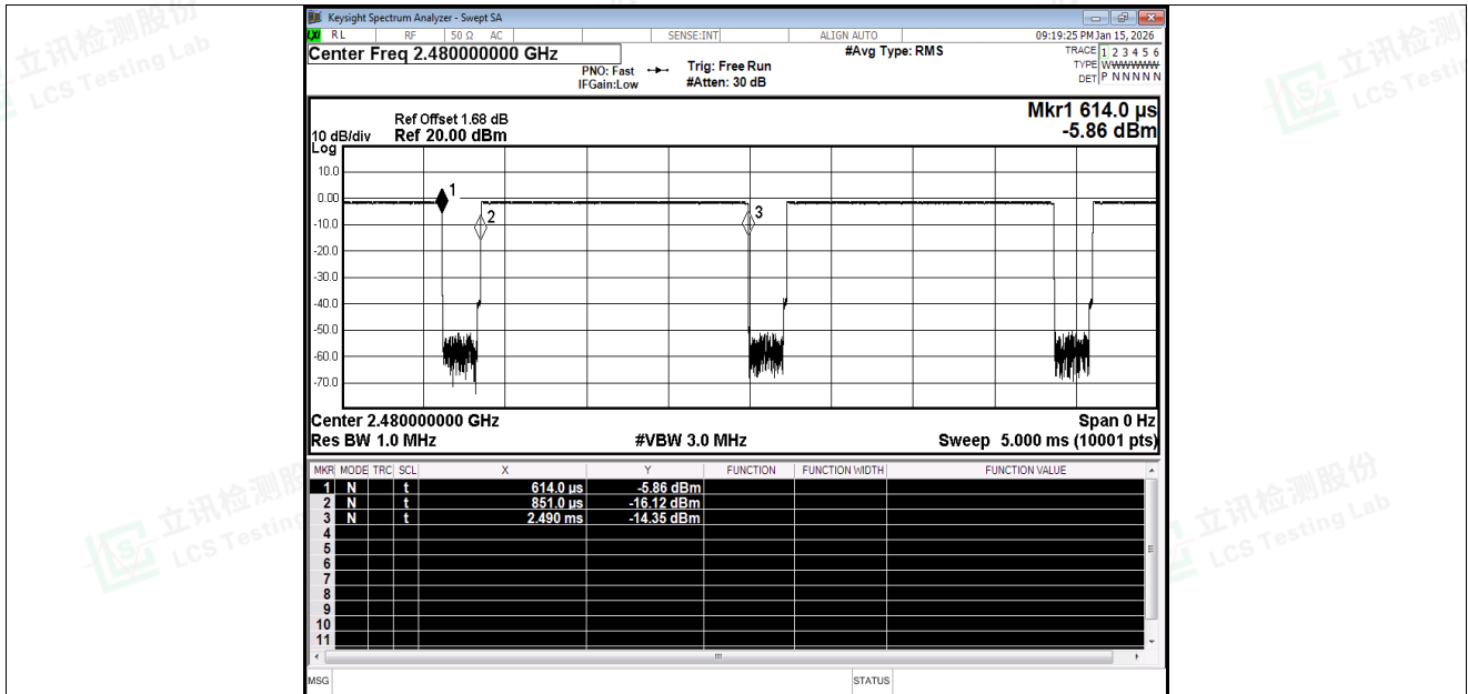
Duty Cycle NVNT BLE 1M 2480MHz Ant1
