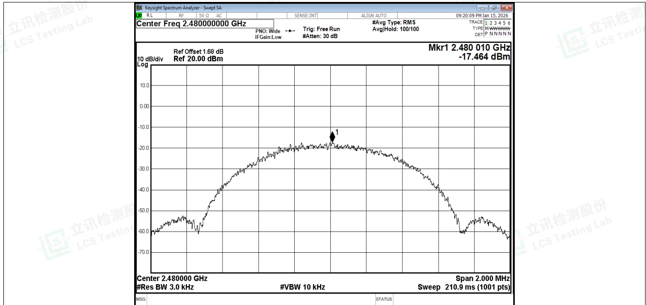
PSD NVNT BLE 1M 2480MHz Ant1
