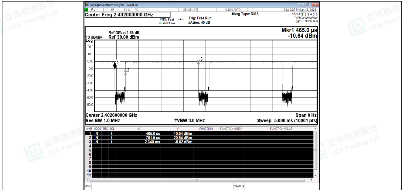
Duty Cycle NVNT BLE 1M 2402MHz Ant1
