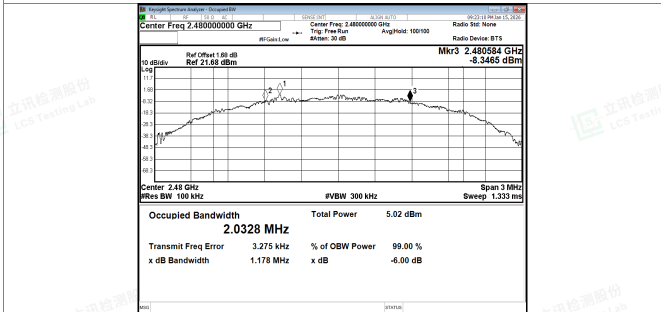
-6dB Bandwidth NVNT BLE 2M 2480MHz Ant1
