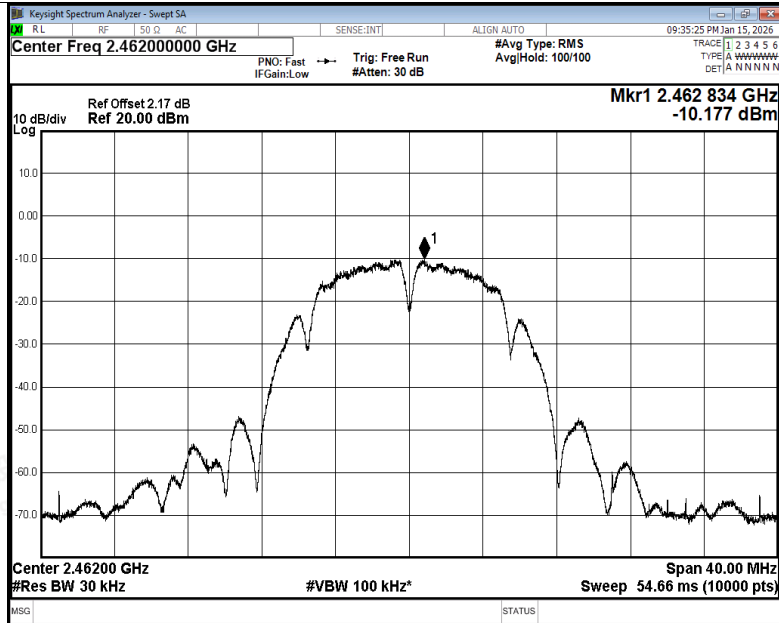
PSD NVNT b 2462MHz Ant1
