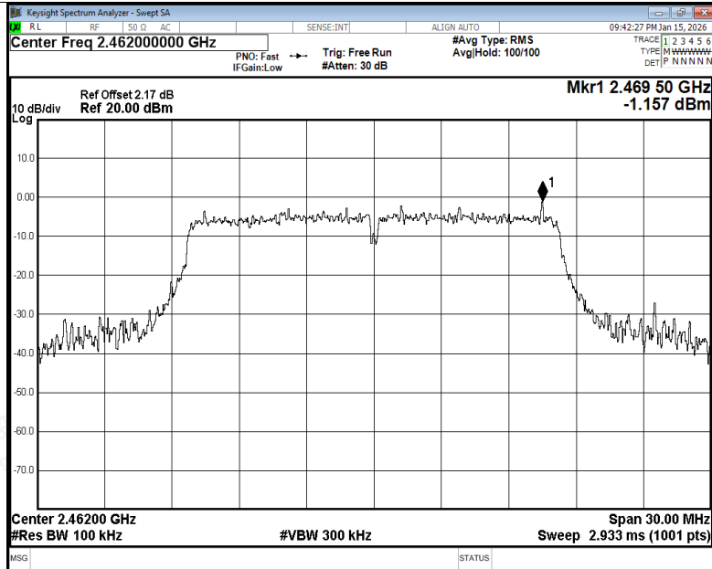
Band Edge NVNT g 2462MHz Ant1 Ref
