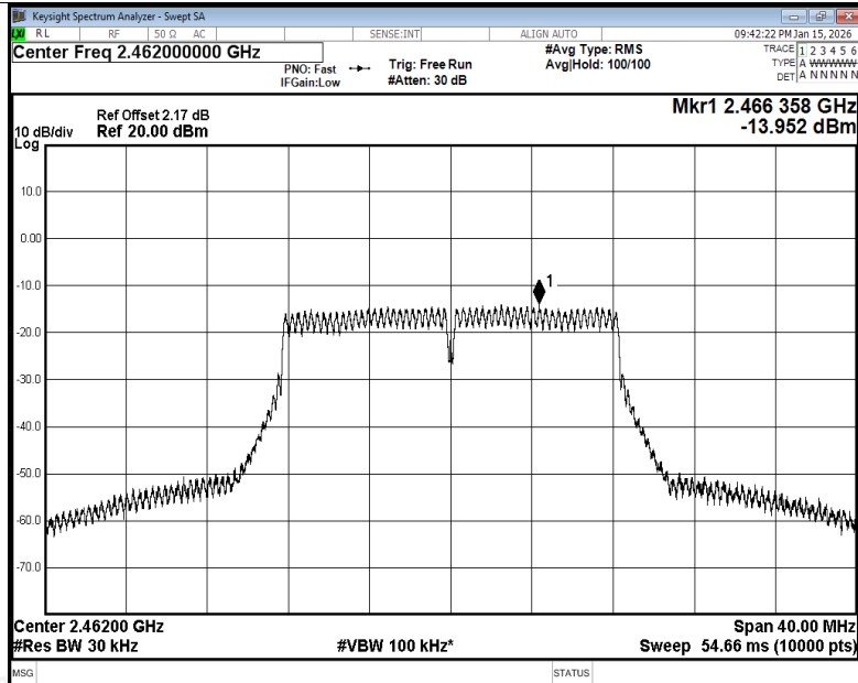
PSD NVNT g 2462MHz Ant1
