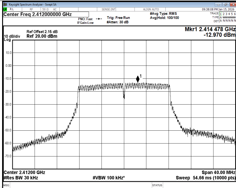
PSD NVNT g 2412MHz Ant1
