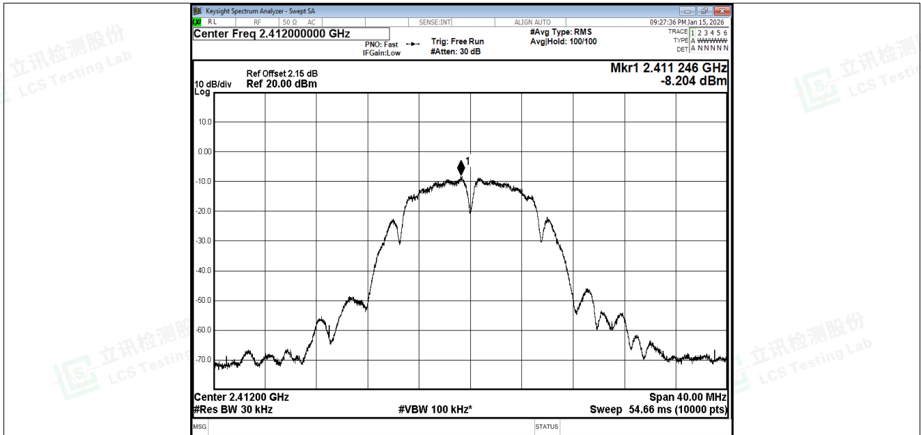
PSD NVNT b 2412MHz Ant1
