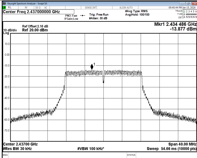
PSD NVNT g 2437MHz Ant1
