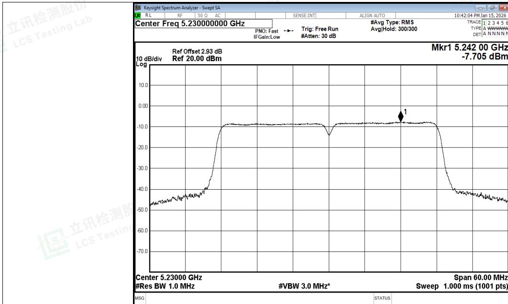
PSD NVNT ac40 5230MHz Ant1
