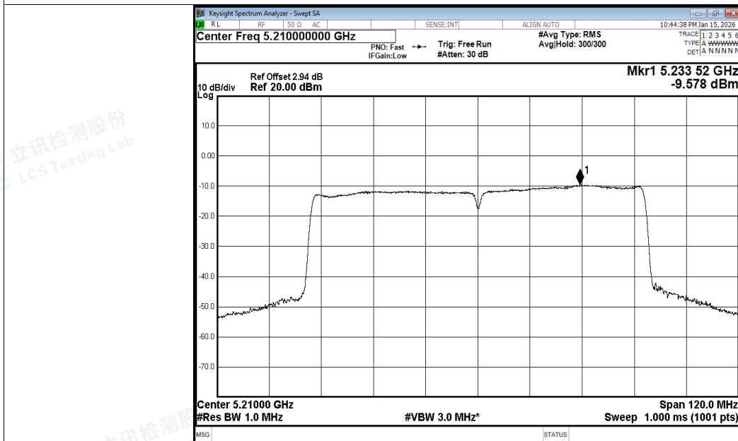
PSD NVNT ac80 5210MHz Ant1
