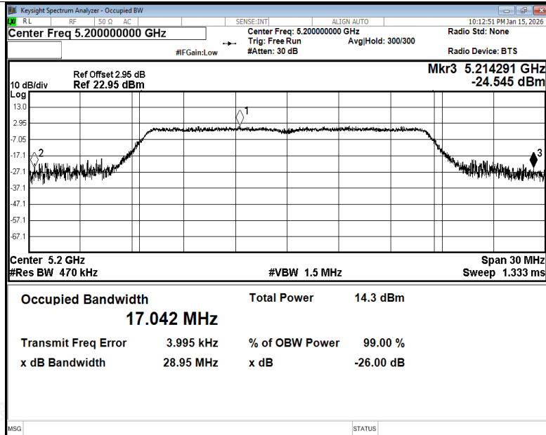
-26dB Bandwidth NVNT a 5200MHz Ant1
