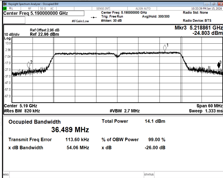
-26dB Bandwidth NVNT n40 5190MHz Ant1
