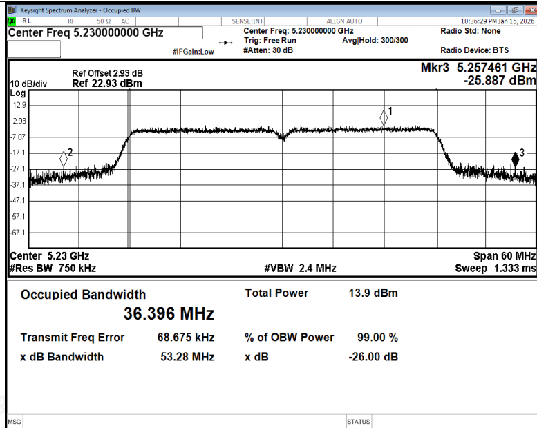
-26dB Bandwidth NVNT n40 5230MHz Ant1
