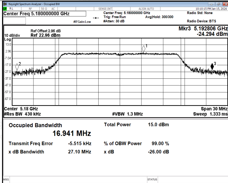
-26dB Bandwidth NVNT a 5180MHz Ant1
