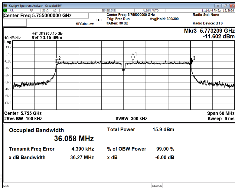
-6dB Bandwidth NVNT ac40 5755MHz Ant1
