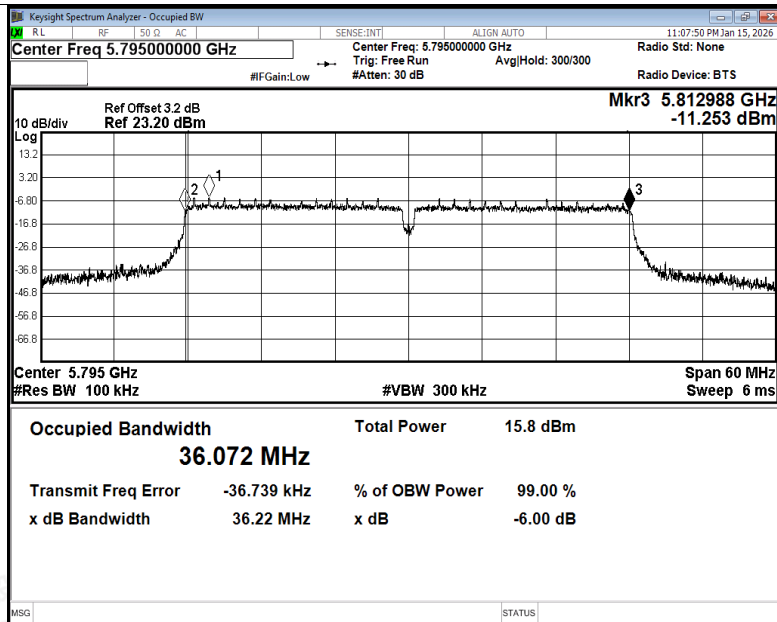
-6dB Bandwidth NVNT n40 5795MHz Ant1
