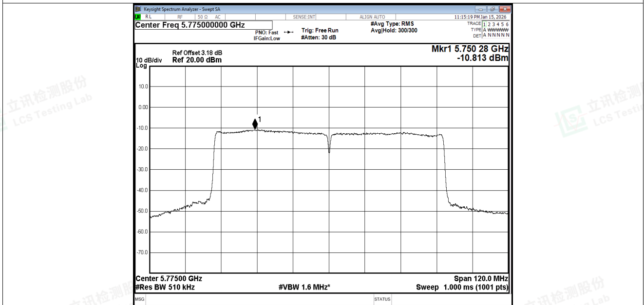
PSD NVNT ac80 5775MHz Ant1
