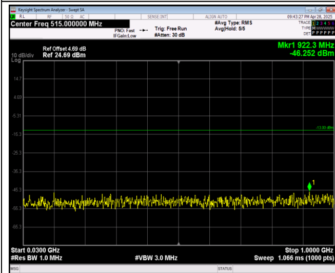
Band4-20MHz-QPSK-20175-1RB#0-Range1:30~100 0MHz
