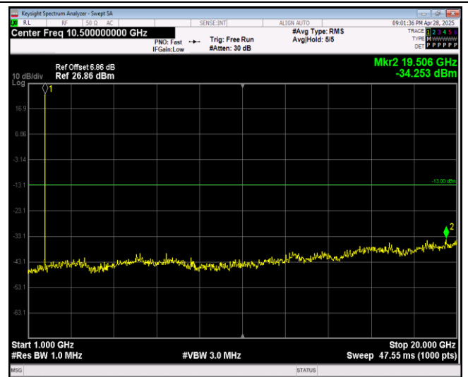
Band4-20MHz-QPSK-20050-1RB#0-Range2:1000~2 0000MHz
