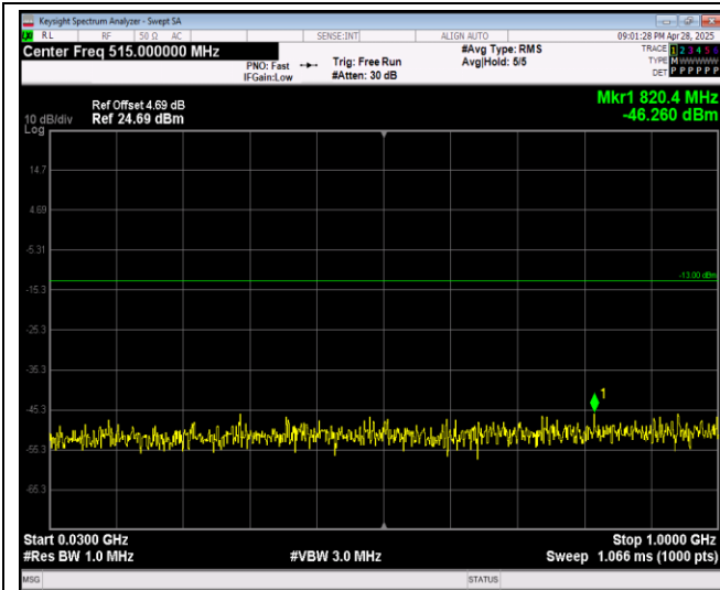
Band4-20MHz-QPSK-20050-1RB#0-Range1:30~100 0MHz
