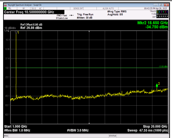
Band4-20MHz-QPSK-20175-1RB#0-Range2:1000~2 0000MHz
