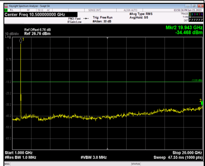
Band2-20MHz-QPSK-18900-1RB#0-Range2:1000~ 20000MHz
