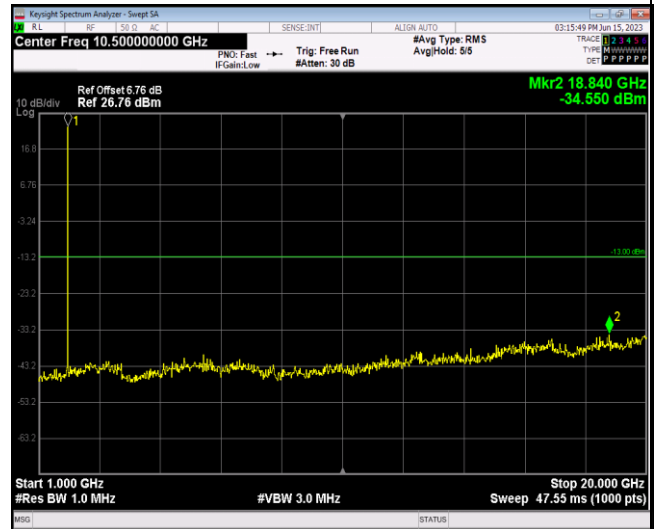
Band2-20MHz-QPSK-18700-1RB#0-Range2:1000~ 20000MHz
