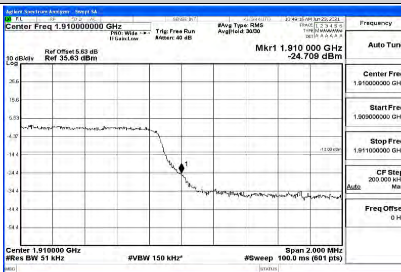
Band2-5MHz-QPSK-18625-25RB#0
