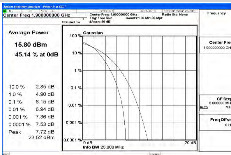
Band2-20MHz-16QAM-19100-100RB#0
