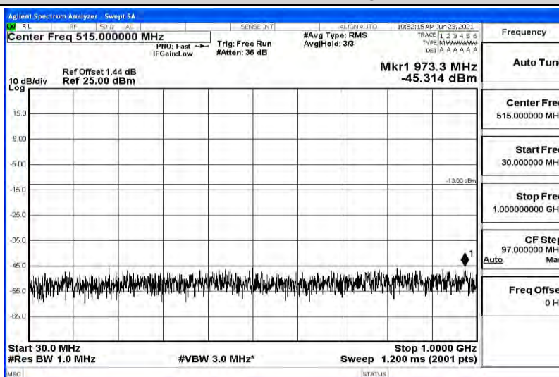
Band2-3MHz-QPSK-18900-1RB#0-Range4:1000~10000MHz
