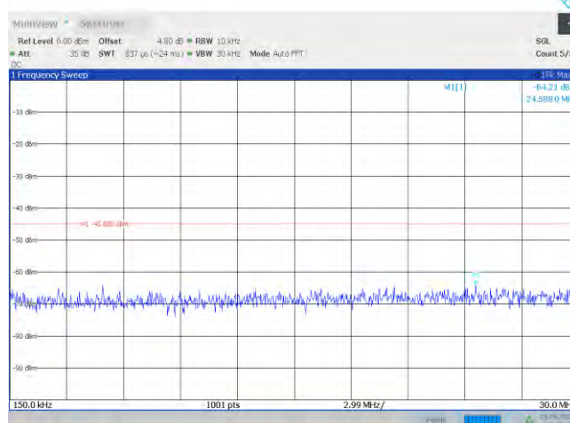
Band41-20MHz-QPSK-39750-1RB#0-Range2:0.15~30MHz
