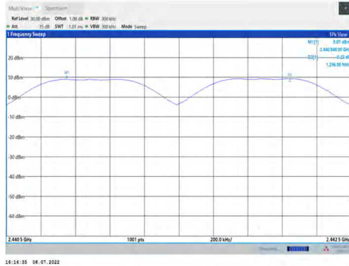
2DH5_Ant7_Hop
