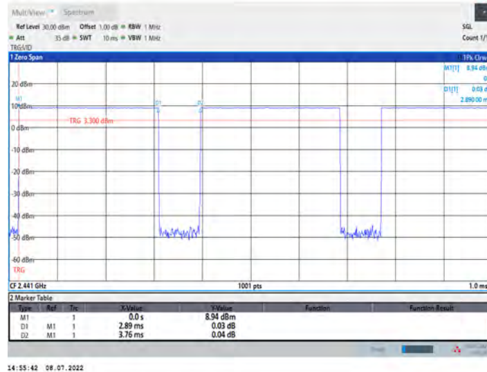
DH5_Ant7_2441
