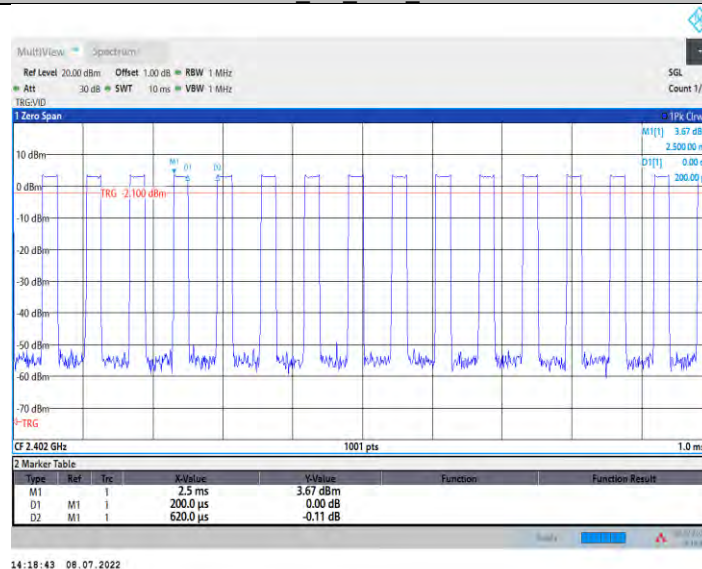
BLE_2M_Ant7_2402
