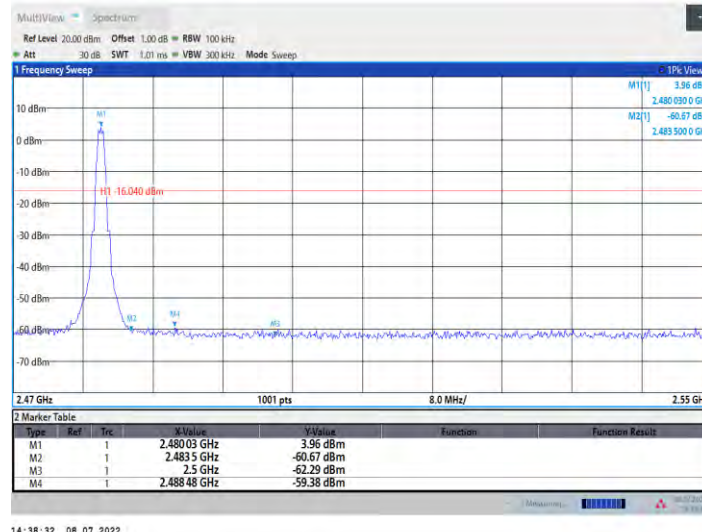
BLE 1M Ant7 High 2480
