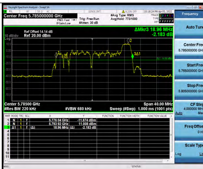
11AX20MIMO_Ant0_5785_242Tone_RU61
