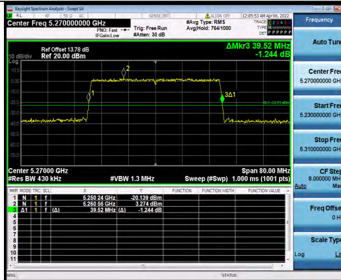
11AX40MIMO_Ant1_5270_26Tone_RU0
