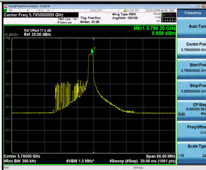
11AX40MIMO_Ant1_5795_26Tone_RU17
