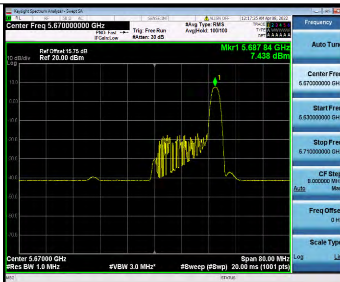
11AX40MIMO_Ant1_5670_484Tone_RU65
