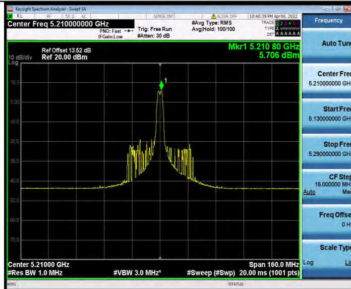
11AX80MIMO_Ant0_5210_26Tone_RU36
