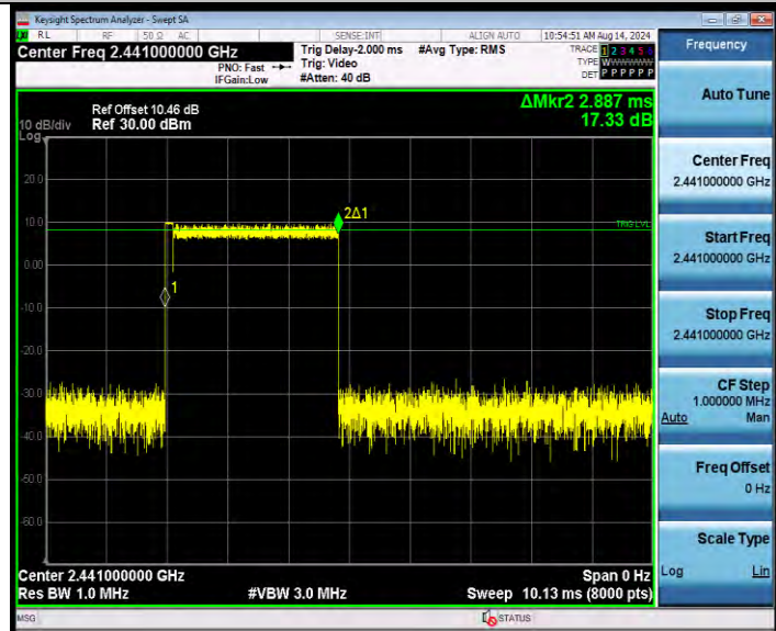
3DH5_Ant1_Hop
