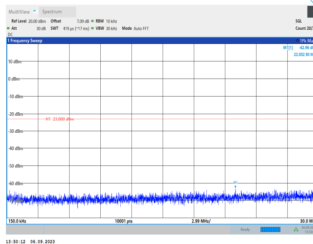
GSM850-128-0.15~30MHz
