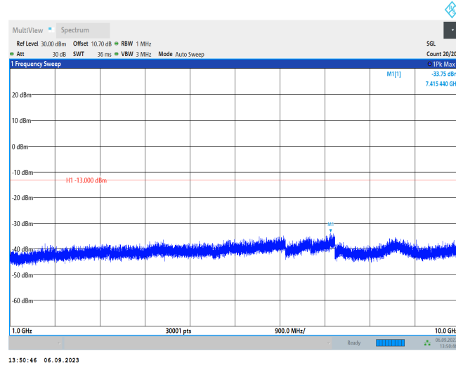
GSM850-190-1000~10000MHz
