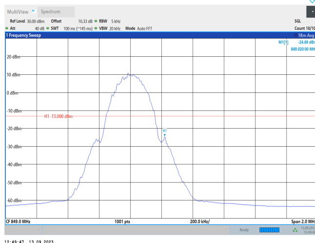
GSM850-251
