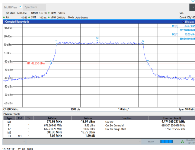
Band71-5MHz-QPSK-133297-25RB#0
