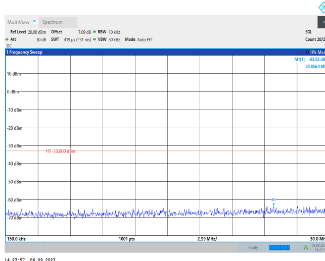
BandII-9262-0.15~30MHz
