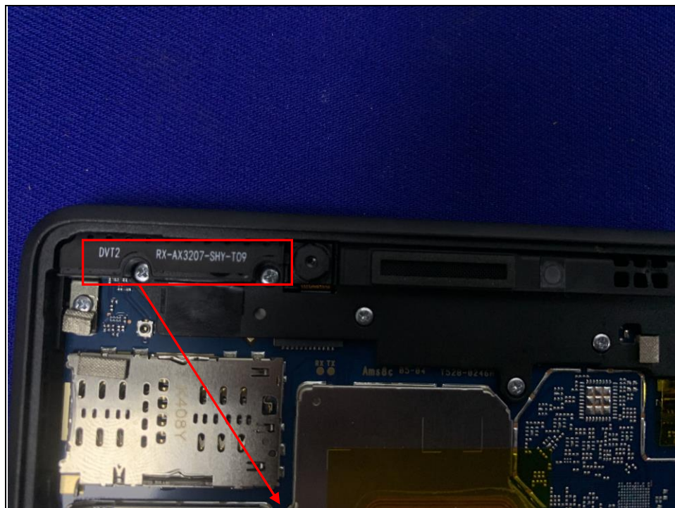
BT/WIFI Antenna
