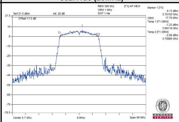
802.11ac (20MHz)
