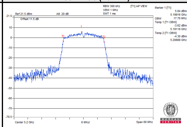
802.11ac (20MHz)
