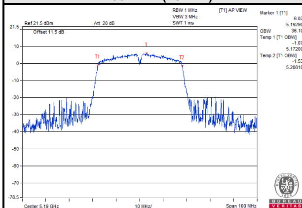
802.11n (40MHz)
