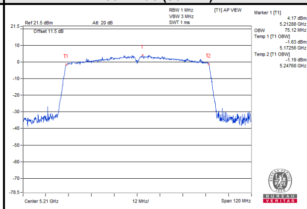
802.11ac (80MHz)
