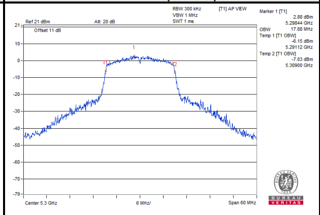
802.11ac (20MHz)
