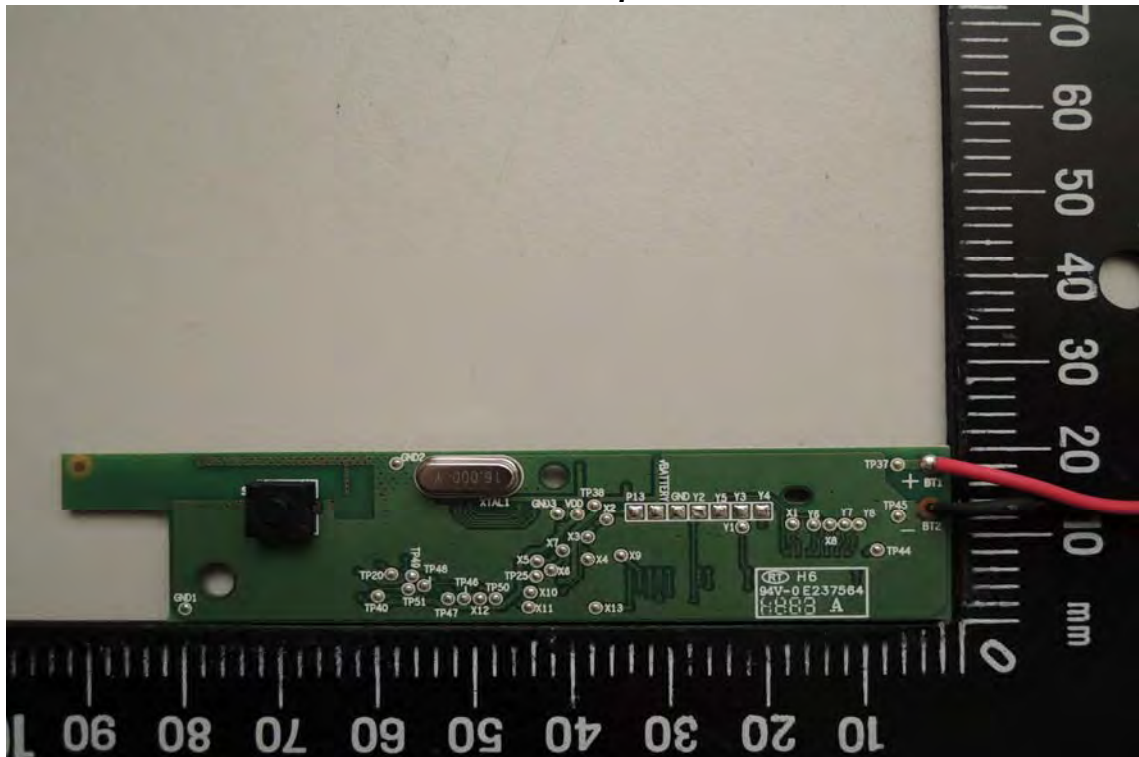
2.4G Antenna
