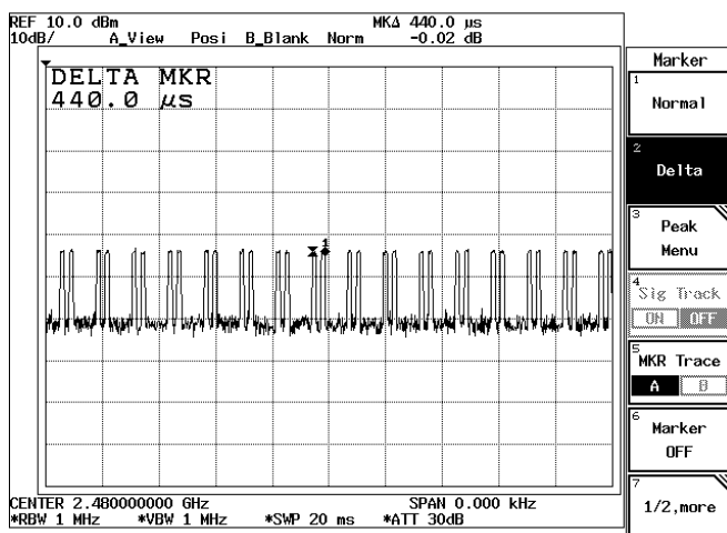
CH 78 2480MHz
