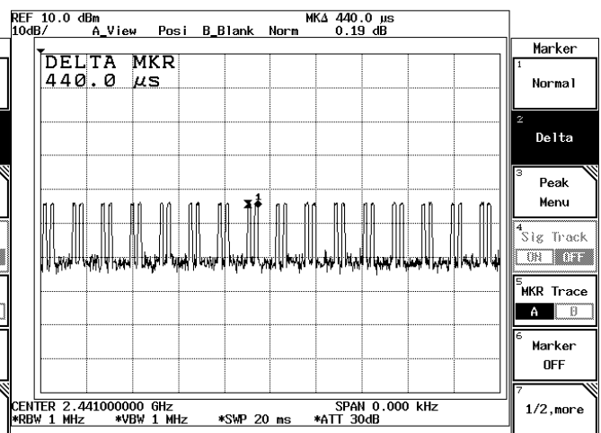
CH 39 2441MHz
