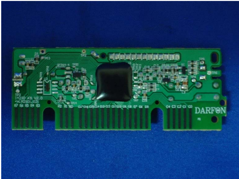
(5) EUT Photo-M/N:IM230
