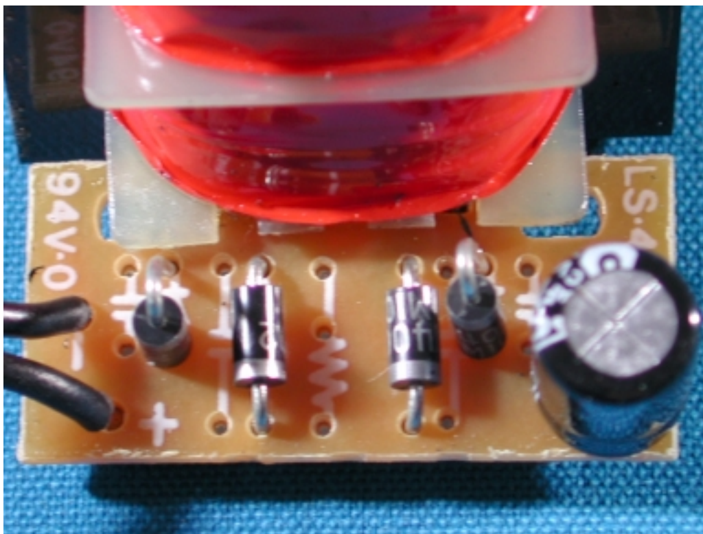
(18) EUT Photo
