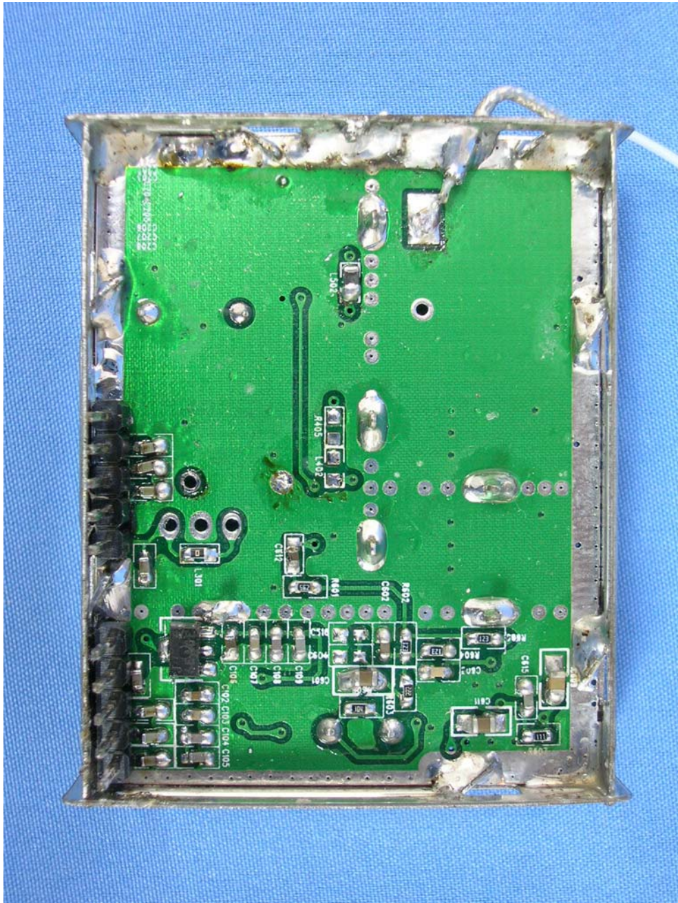
(18) EUT Photo
