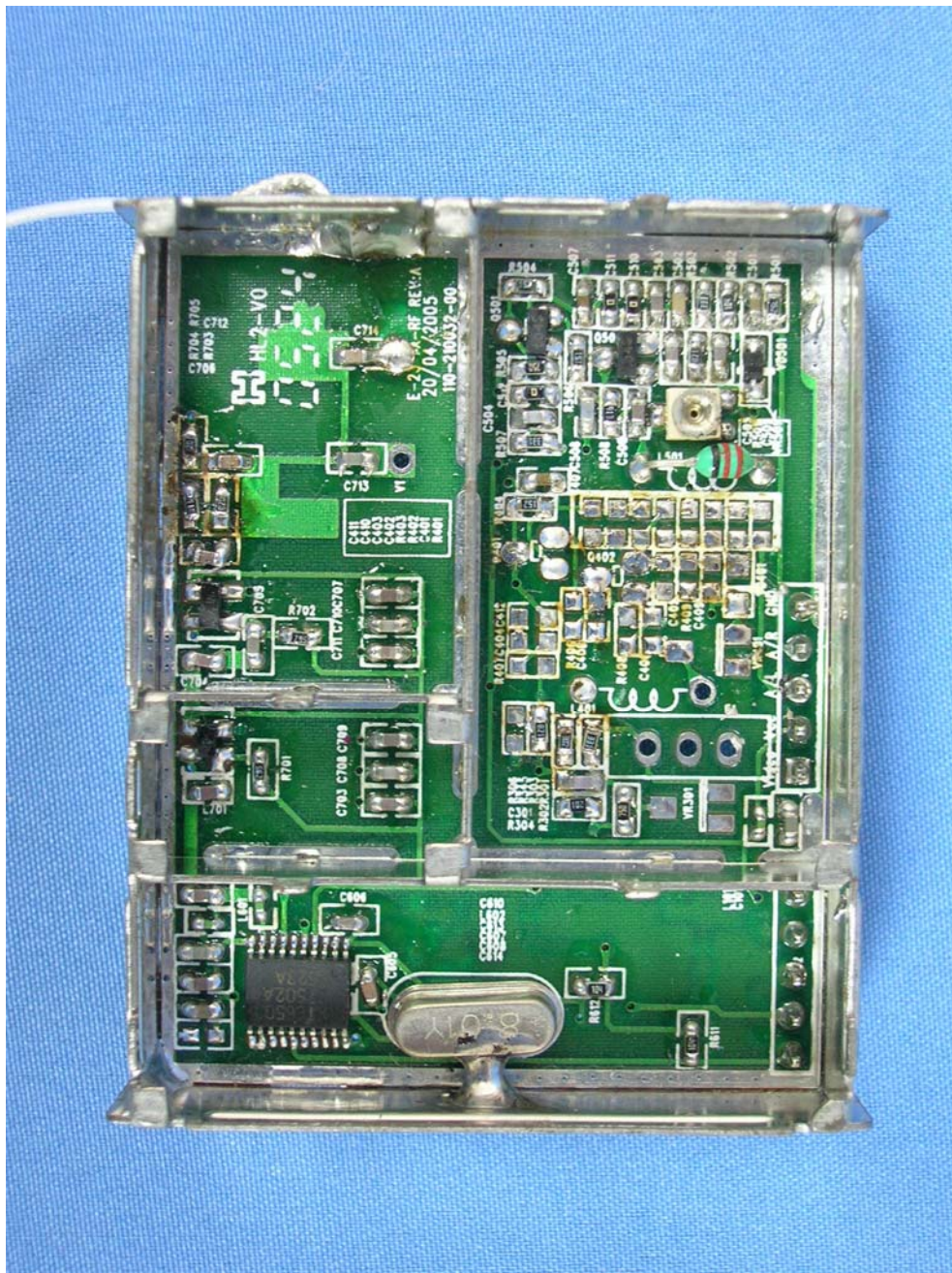
(17) EUT Photo
