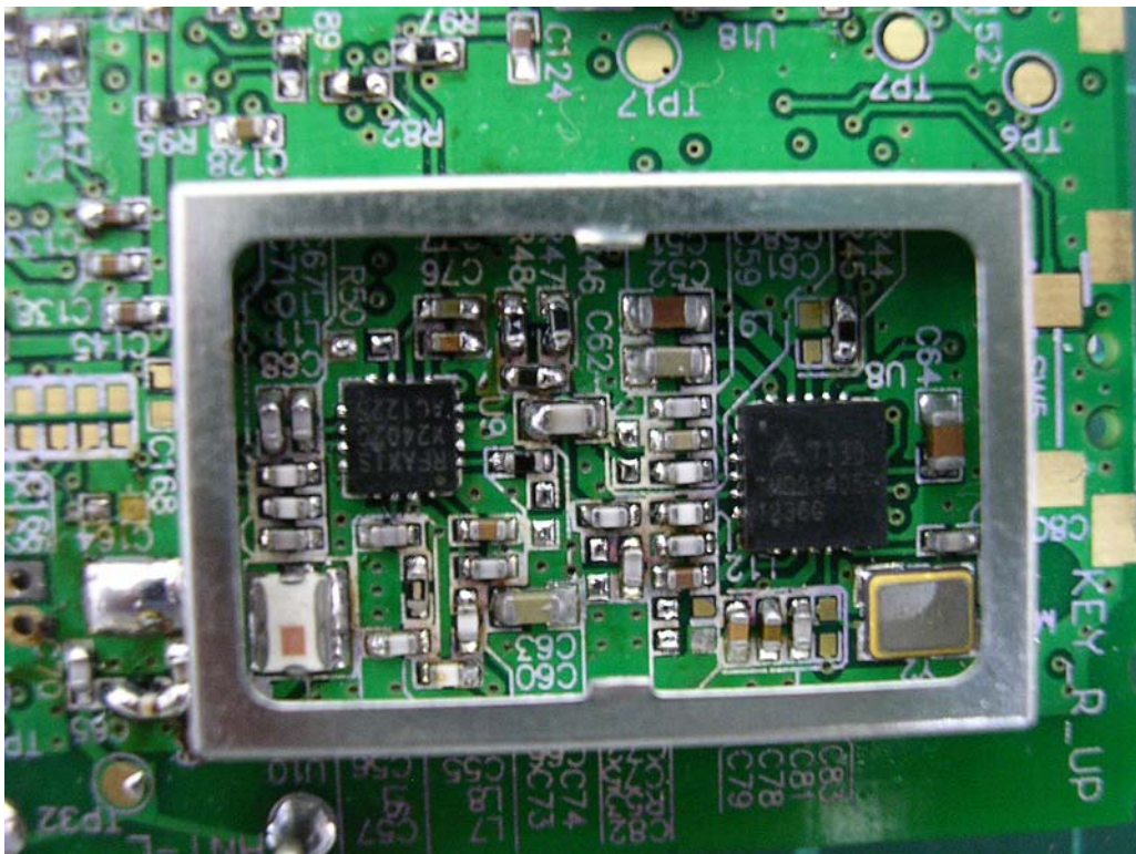
RF module
