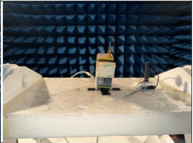
Axis XY
