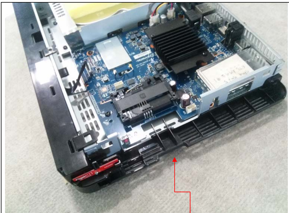
2 GHz, 5 GHz : ANT 2
