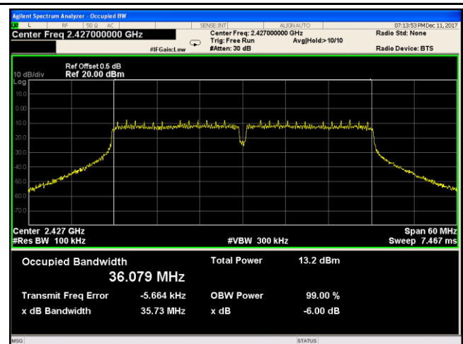
802.11n40 6dB Bandwidth - 4 CH 2427
