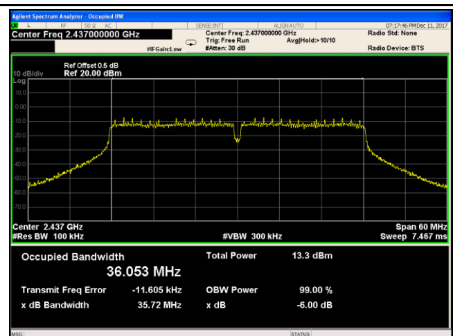
802.11n40 6dB Bandwidth - 6 CH 2437
