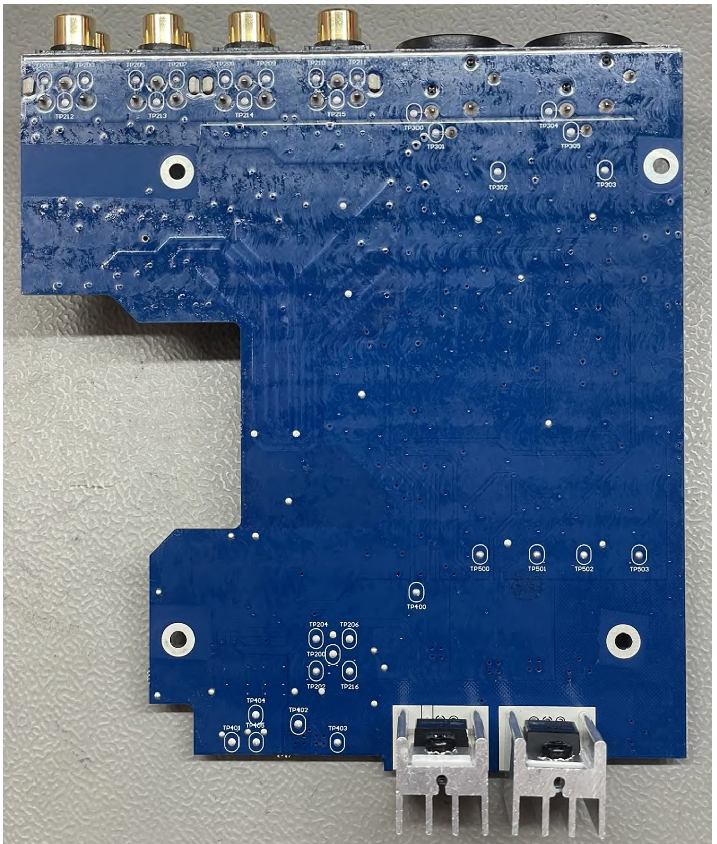
ZCAS4GPREPCB - Caspian 4G PRE-RIAA Assembly BOTTOM.JPG
