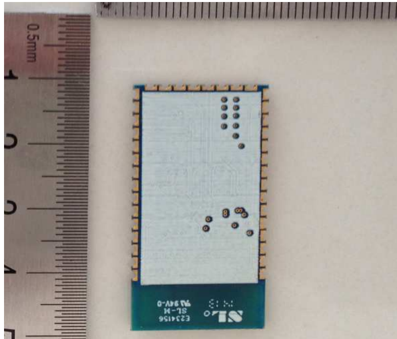
WIFI Module
