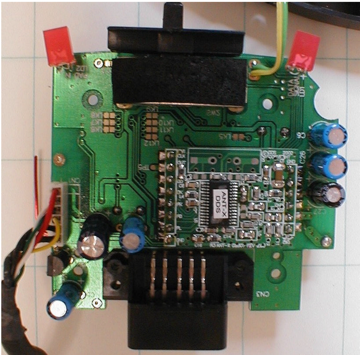
PCB Bottom
