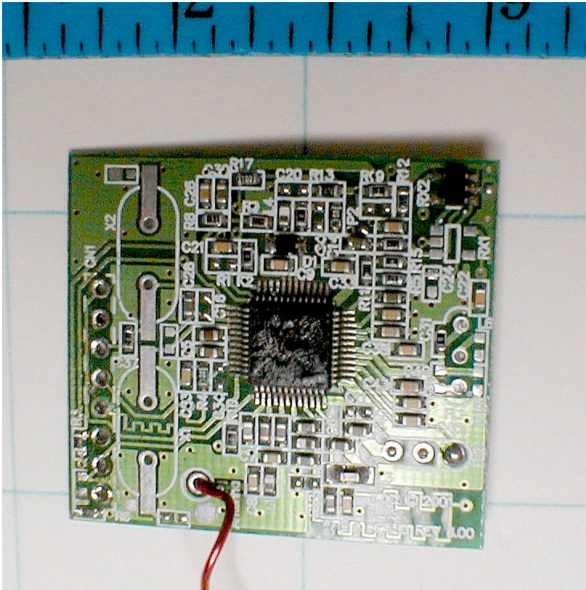
Radio Module Top
