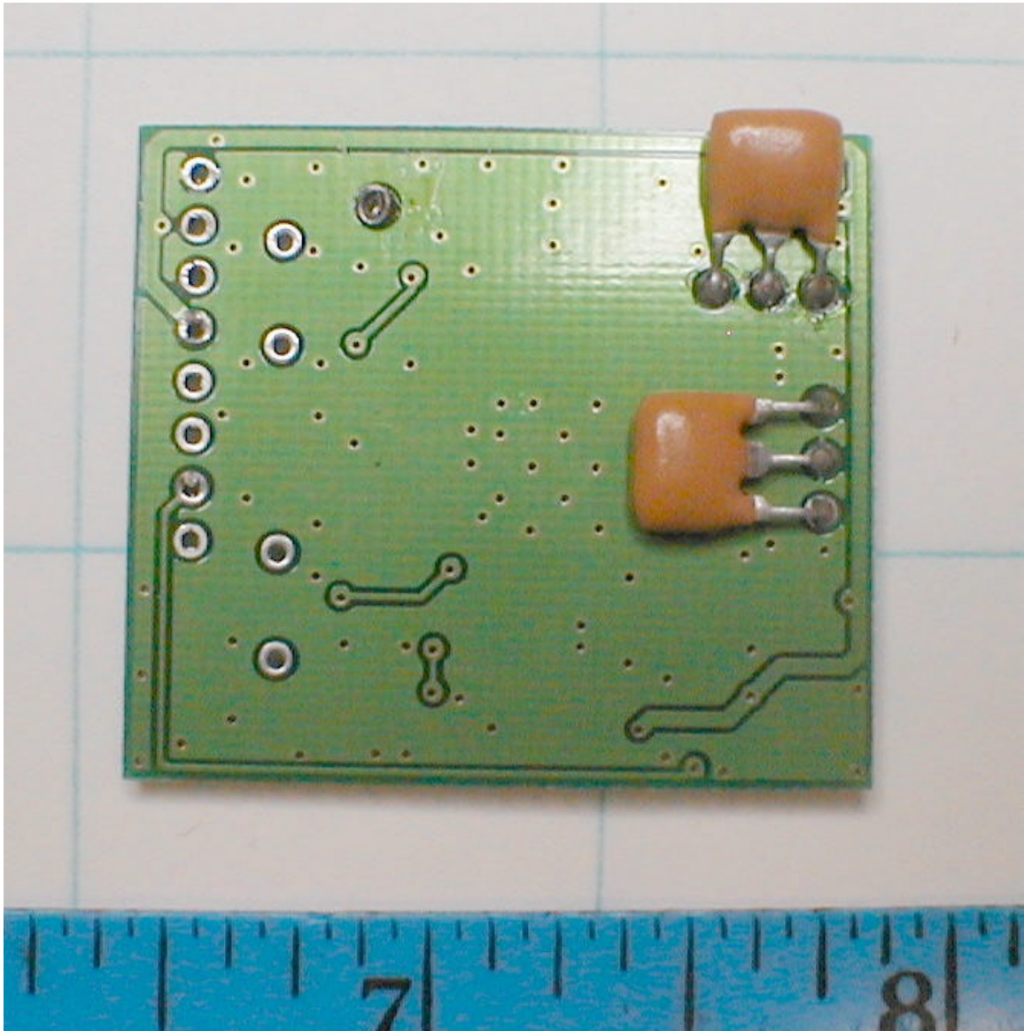
Radio Module Bottom
