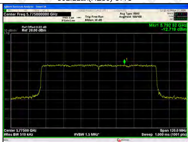
802.11ax(HE80)-5775
