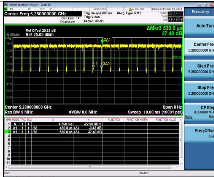
11AX20MIMO_Ant2_5280
