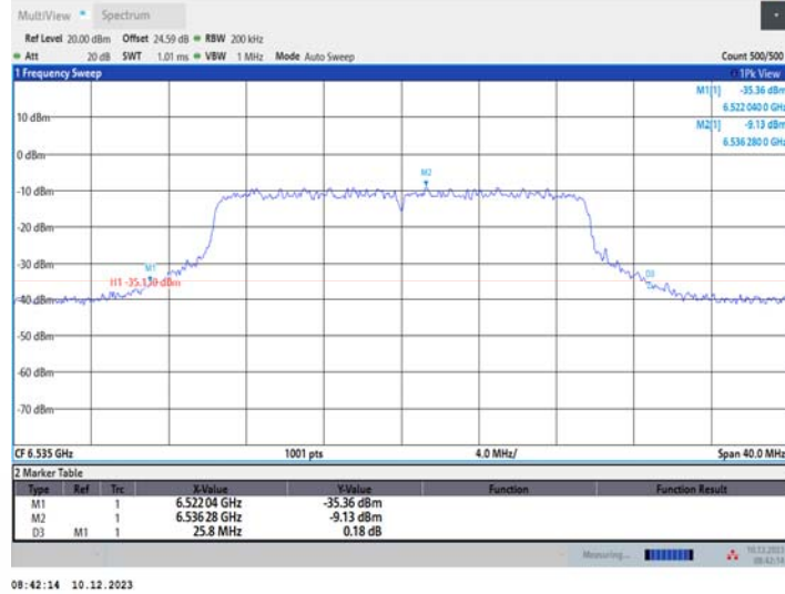
11AX20MIMO_Ant1_6535
