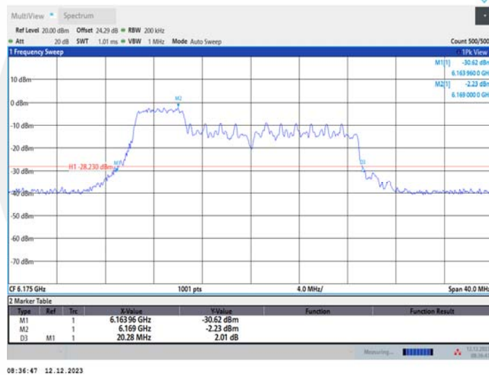
11AX20MIMO_Ant2_6175_106Tone_RU53
