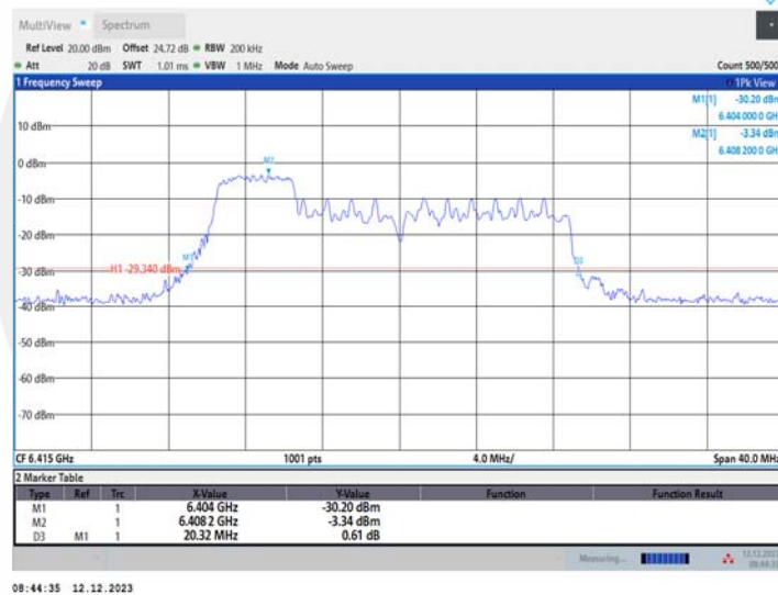
11AX20MIMO_Ant2_6415_106Tone_RU53
