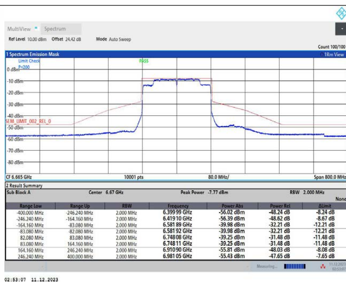
11AX160MIMO_Ant1_6665
