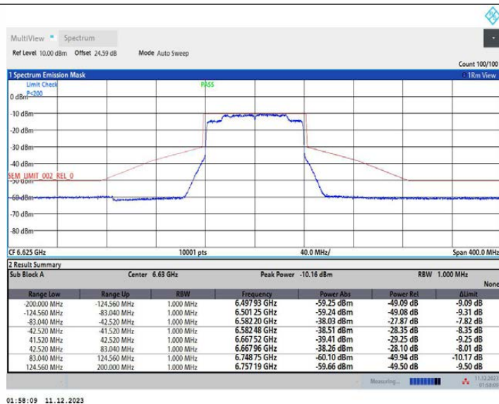
11AX80MIMO_Ant1_6625
