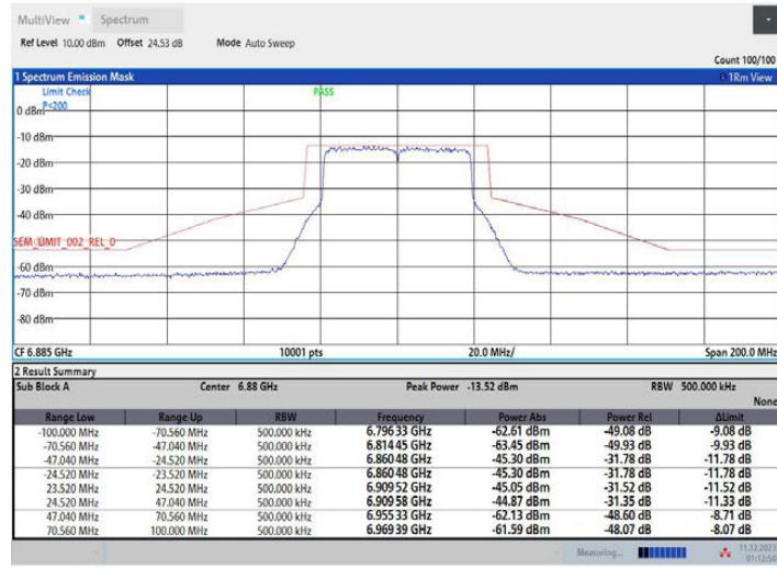
11AX40MIMO_Ant1_6885
