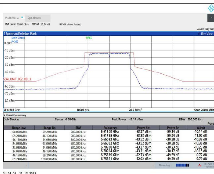
11AX40MIMO_Ant1_6685
