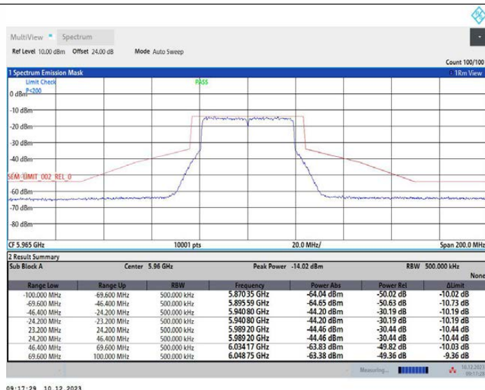
11AX40MIMO_Ant1_5965
