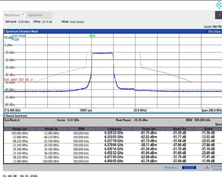
11AX40MIMO_Ant1_6405_26Tone_RU0
