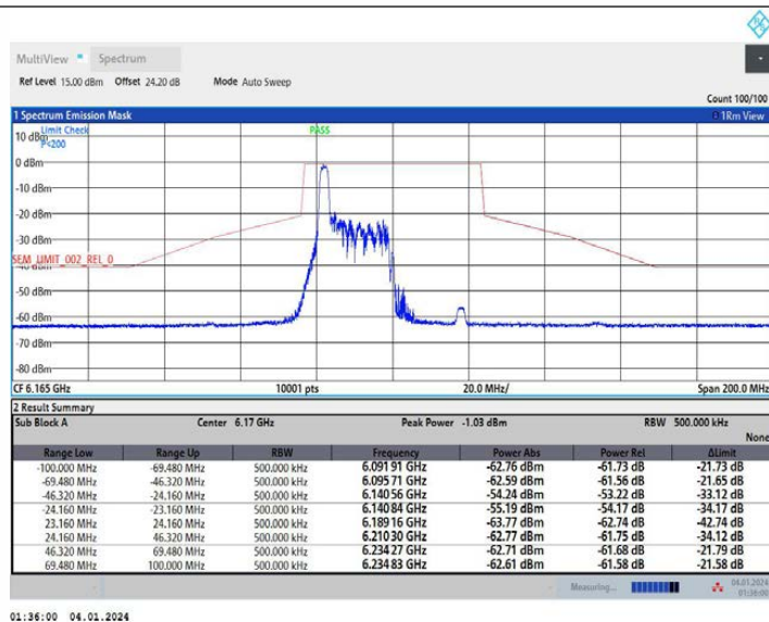
11AX40MIMO Ant1 6165 52Tone RU37
