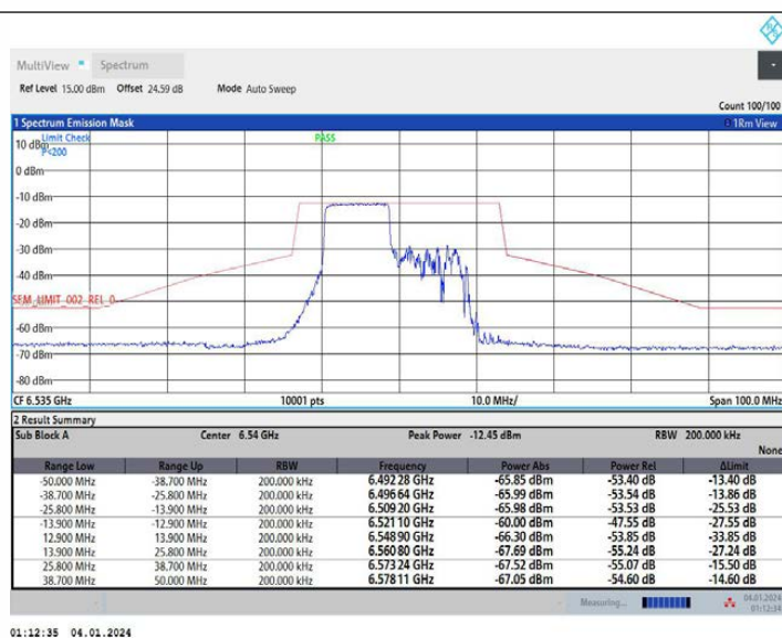
11AX20MIMO Ant1 6535 26Tone RU0
