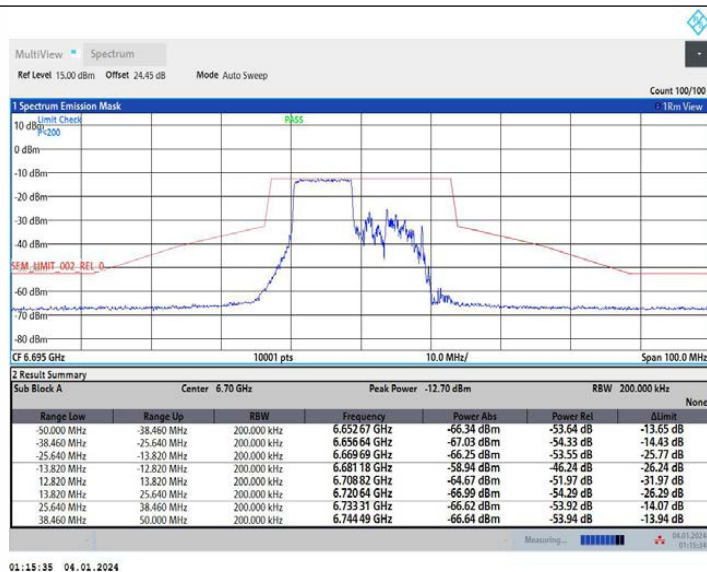
11AX20MIMO Ant1 6695 26Tone RU0
