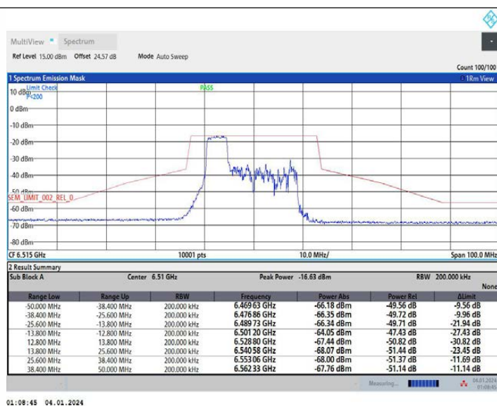
11AX20MIMO_Ant1_6515_106Tone_RU53
