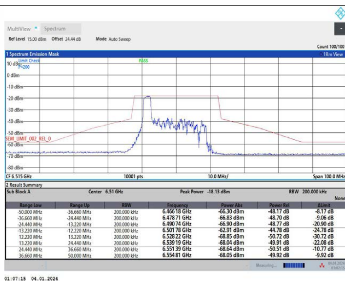
11AX20MIMO_Ant2_6515_52Tone_RU37
