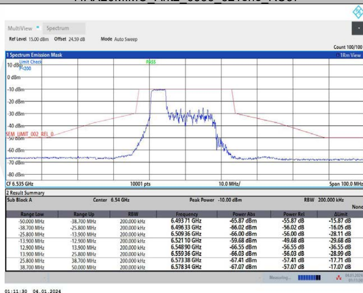
11AX20MIMO Ant2 6535 106Tone RU53
