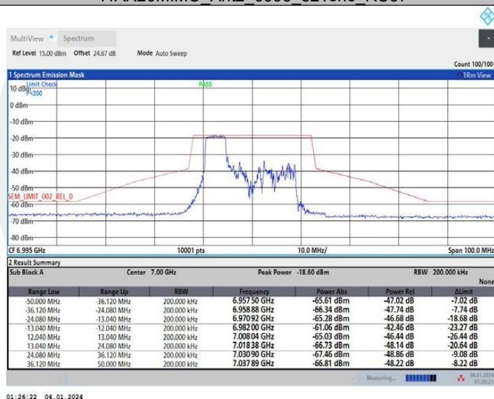
11AX20MIMO_Ant2_6995_106Tone_RU53
