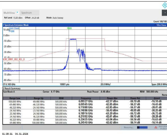
11AX40MIMO_Ant1_6165_242Tone_RU61
