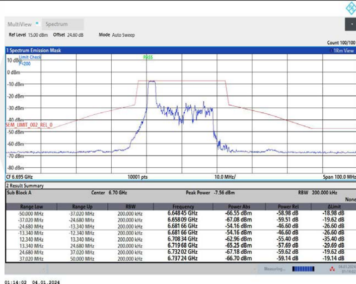
11AX20MIMO Ant1 6695 52Tone RU37
