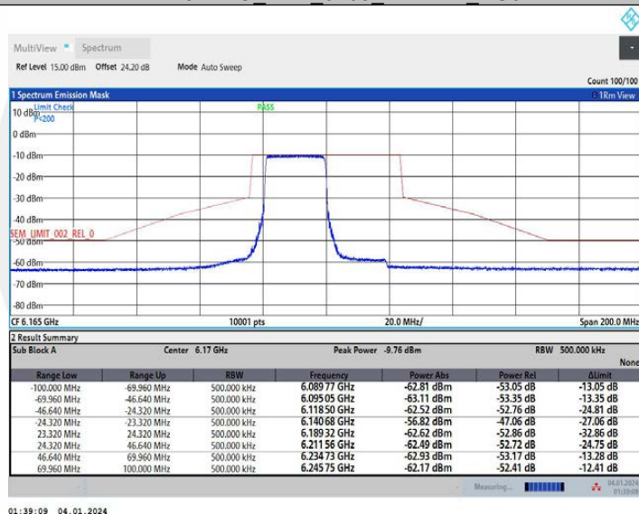
11AX40MIMO_Ant1_6165_26Tone_RU0
