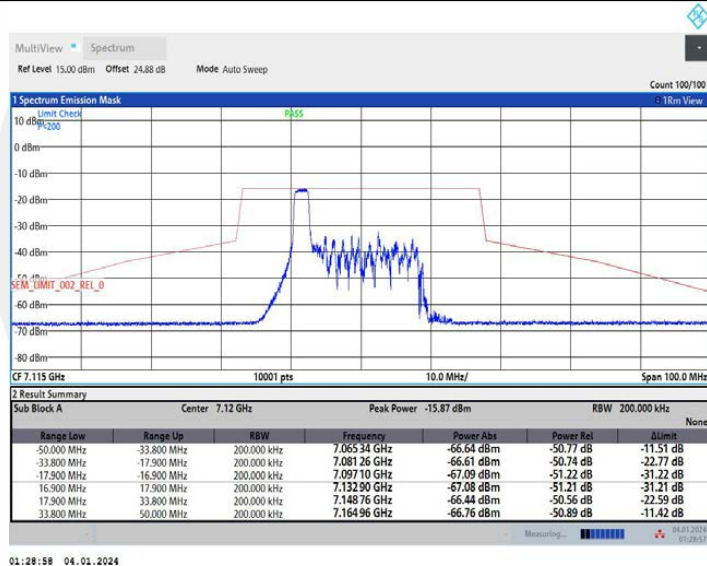
11AX20MIMO Ant1 7115 52Tone RU37
