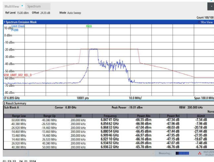
11AX20MIMO_Ant1_6895_106Tone_RU53
