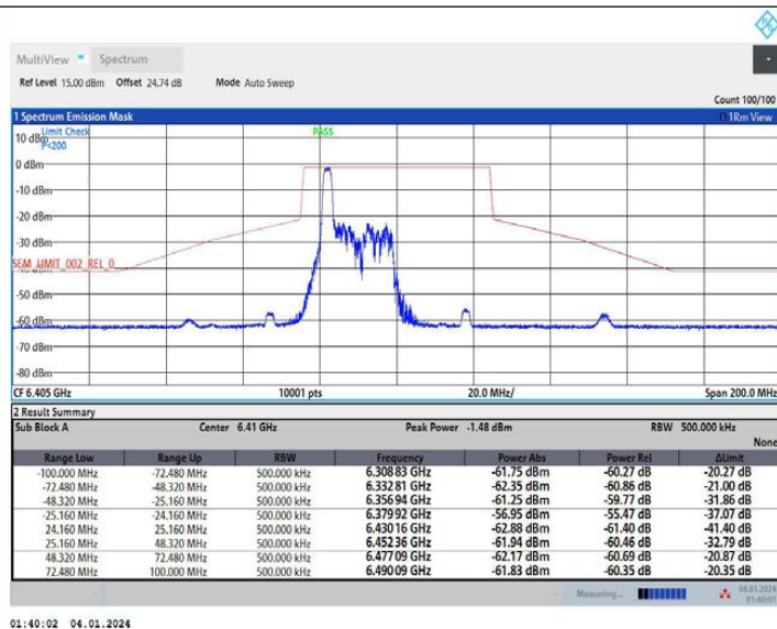
11AX40MIMO_Ant2_6405_52Tone_RU37
