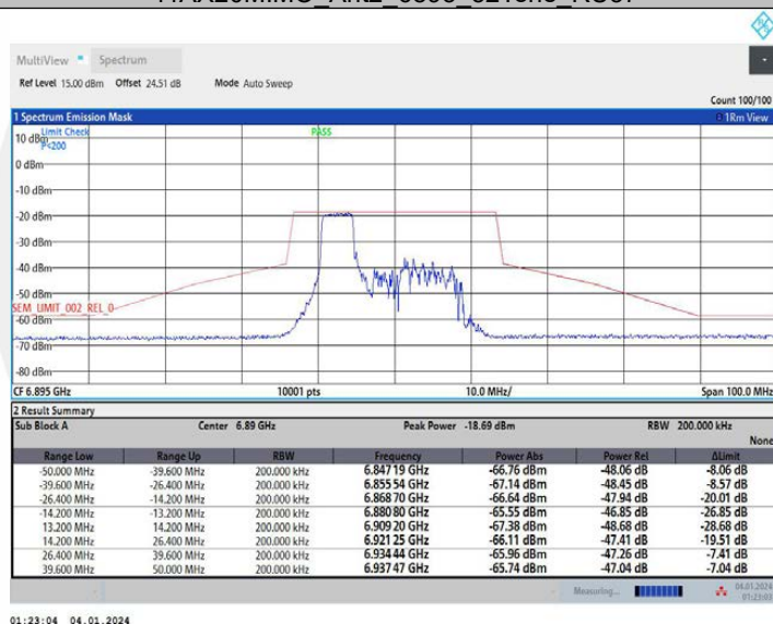
11AX20MIMO_Ant2_6895_106Tone_RU53
