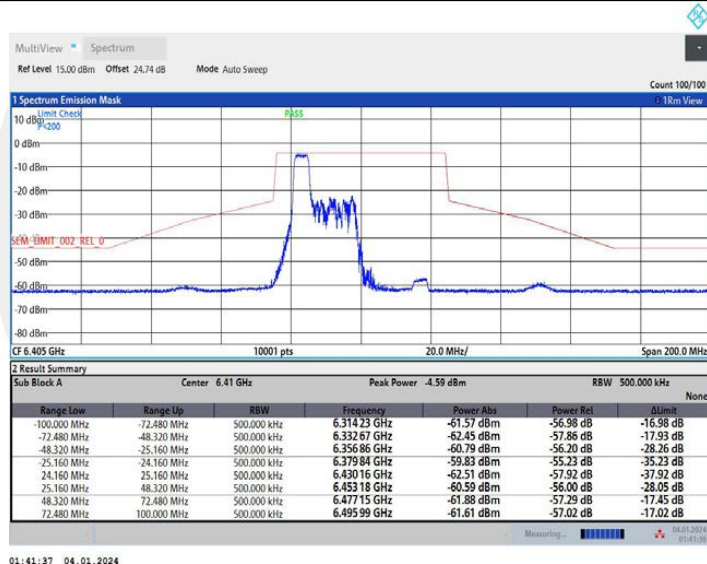
11AX40MIMO_Ant2_6405_106Tone_RU53
