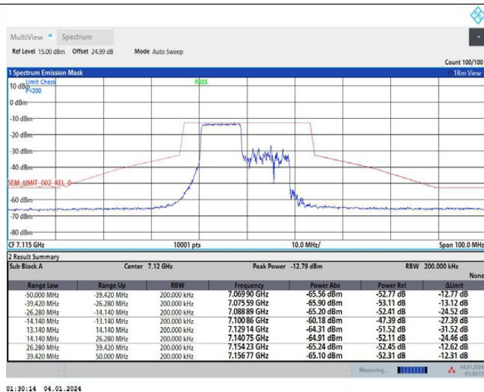
11AX20MIMO Ant1 7115 26Tone RU0
