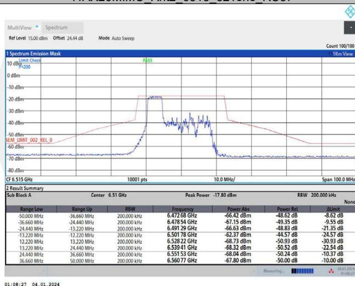
11AX20MIMO_Ant2_6515_106Tone_RU53
