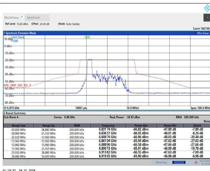
11AX20MIMO_Ant2_6875_52Tone_RU37
