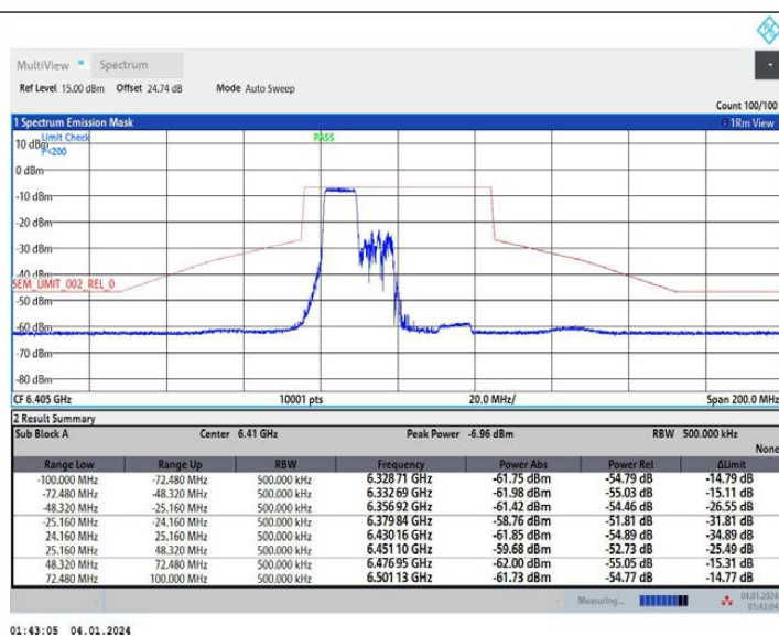
11AX40MIMO_Ant2_6405_242Tone_RU61
