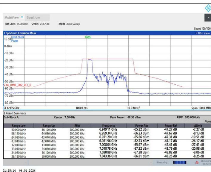
11AX20MIMO_Ant2_6995_52Tone_RU37
