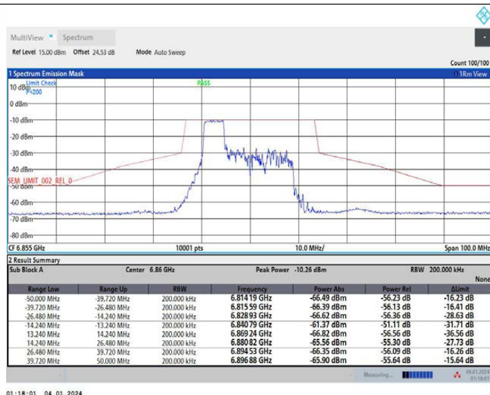
11AX20MIMO_Ant1_6855_106Tone_RU53
