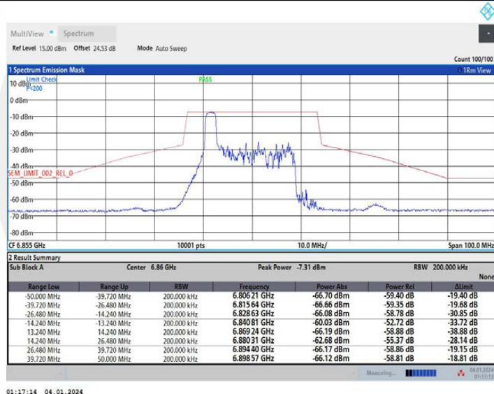
11AX20MIMO Ant1 6855_52Tone RU37
