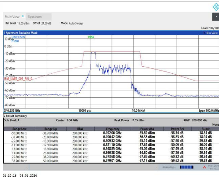
11AX20MIMO Ant2 6535 52Tone RU37
