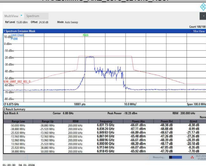
11AX20MIMO_Ant2_6875_106Tone_RU53
