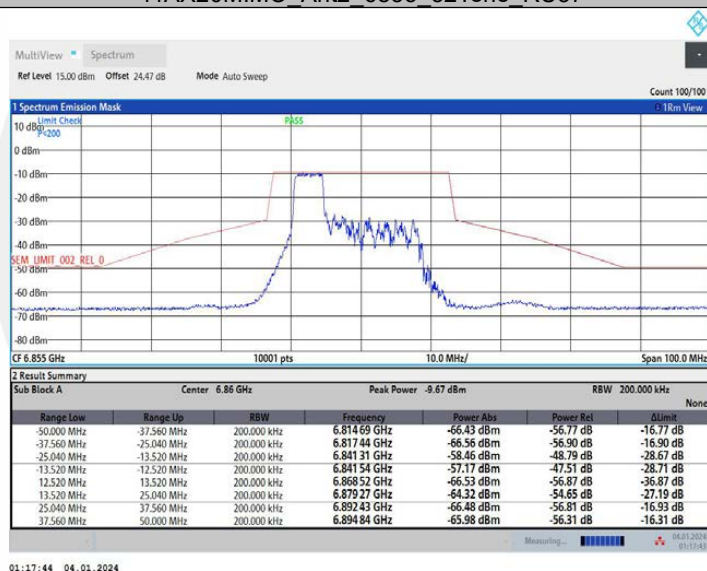
11AX20MIMO_Ant2_6855_106Tone_RU53
