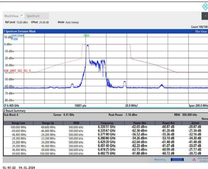
11AX40MIMO Ant1 6405 52Tone RU37
