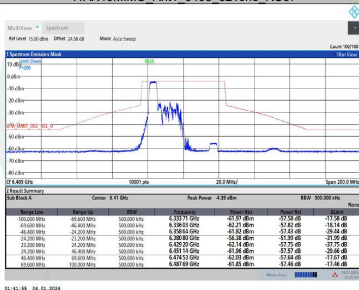
11AX40MIMO Ant1 6405 106Tone RU53
