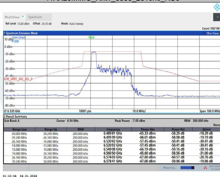
11AX20MIMO Ant1 6535 52Tone RU37
