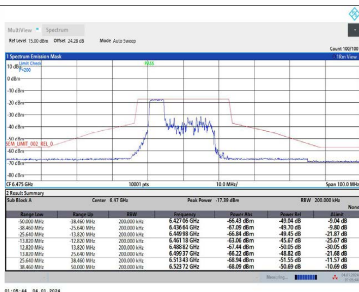
11AX20MIMO_Ant1_6475_106Tone_RU53
