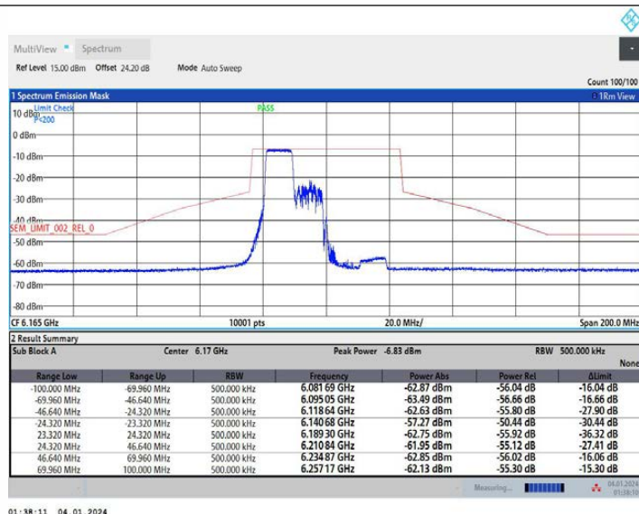
11AX40MIMO_Ant2_6165_242Tone_RU61
