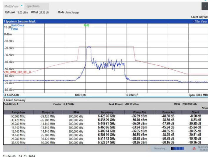
11AX20MIMO_Ant2_6475_52Tone_RU37
