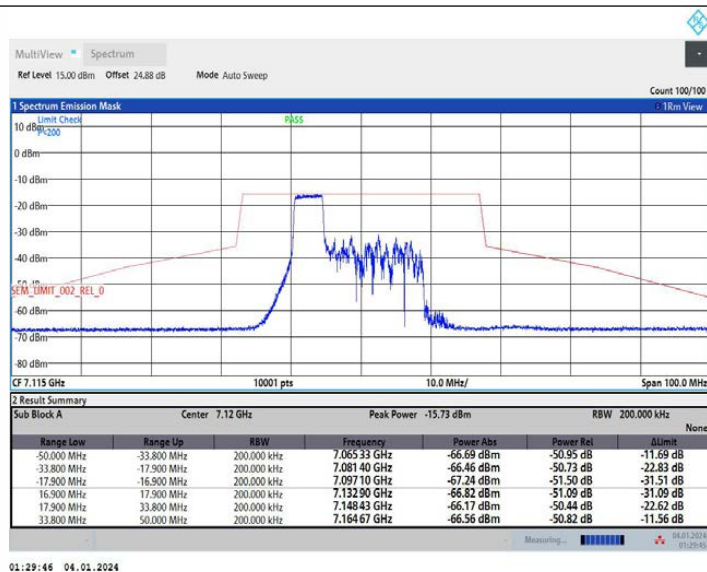
11AX20MIMO_Ant1_7115_106Tone_RU53
