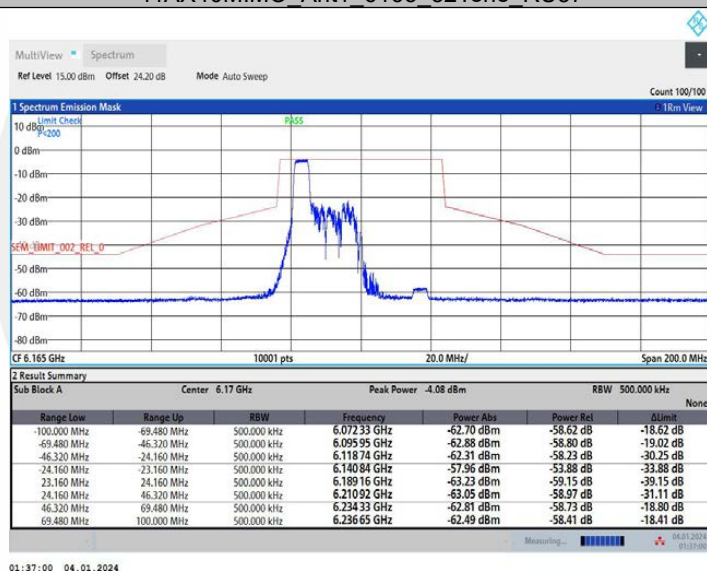
11AX40MIMO Ant1 6165 106Tone RU53
