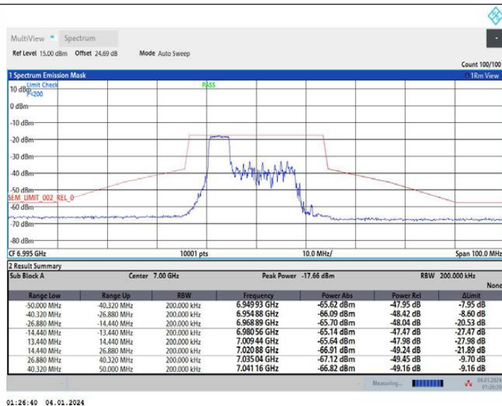
11AX20MIMO_Ant1_6995_106Tone_RU53
