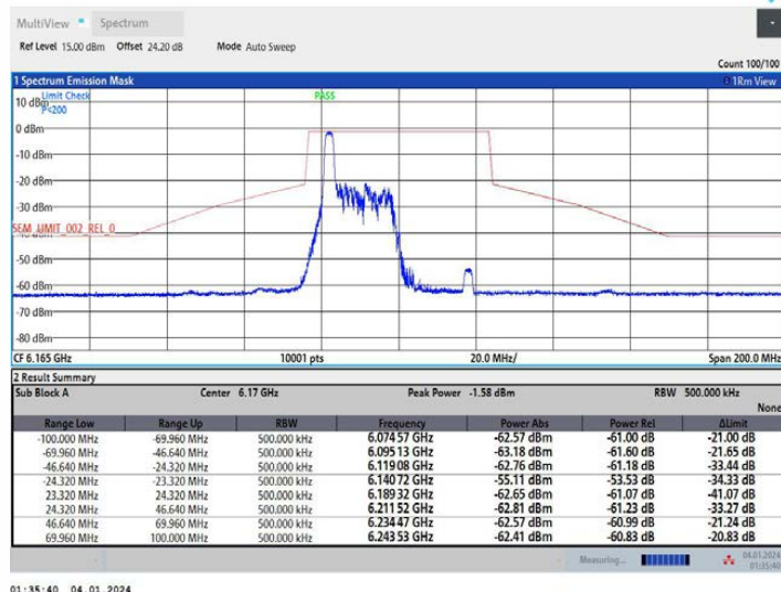
11AX40MIMO_Ant2_6165_52Tone_RU37
