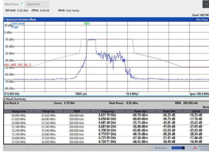
11AX20MIMO_Ant1_6695_106Tone_RU53
