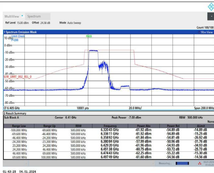
11AX40MIMO_Ant1_6405_242Tone_RU61
