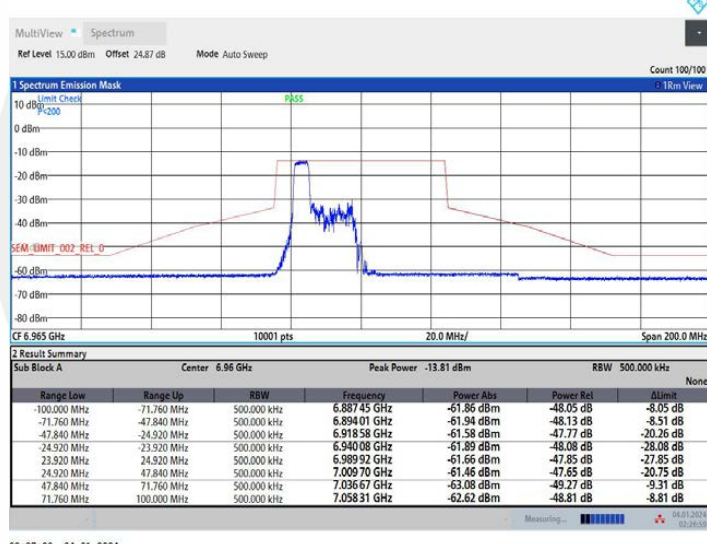
11AX40MIMO Ant1 6965 106Tone RU53
