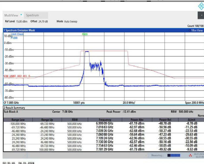
11AX40MIMO Ant1 7085 106Tone RU53
