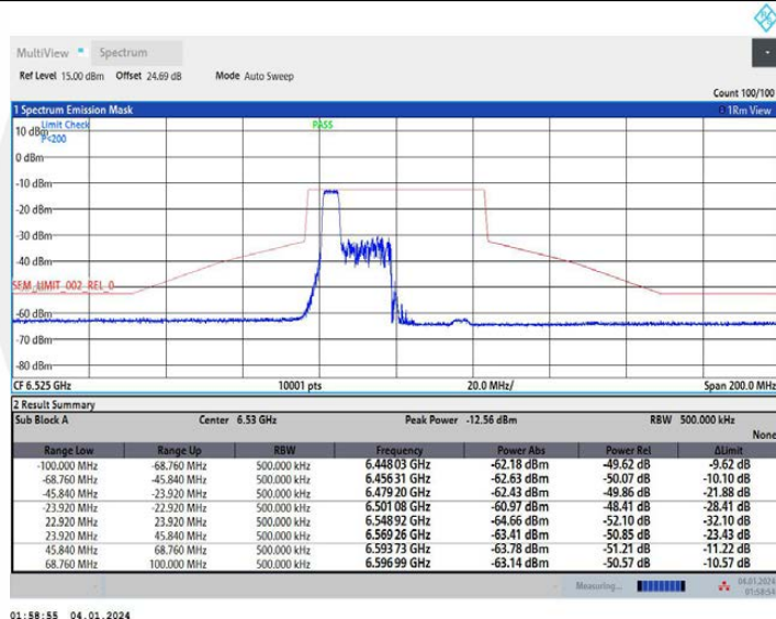
11AX40MIMO Ant1 6525 106Tone RU53
