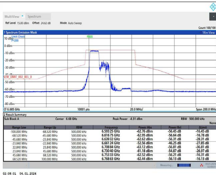
11AX40MIMO Ant1 6685 242Tone RU61
