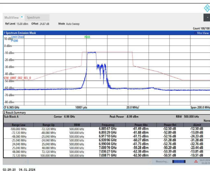
11AX40MIMO_Ant2_6965_242Tone_RU61
