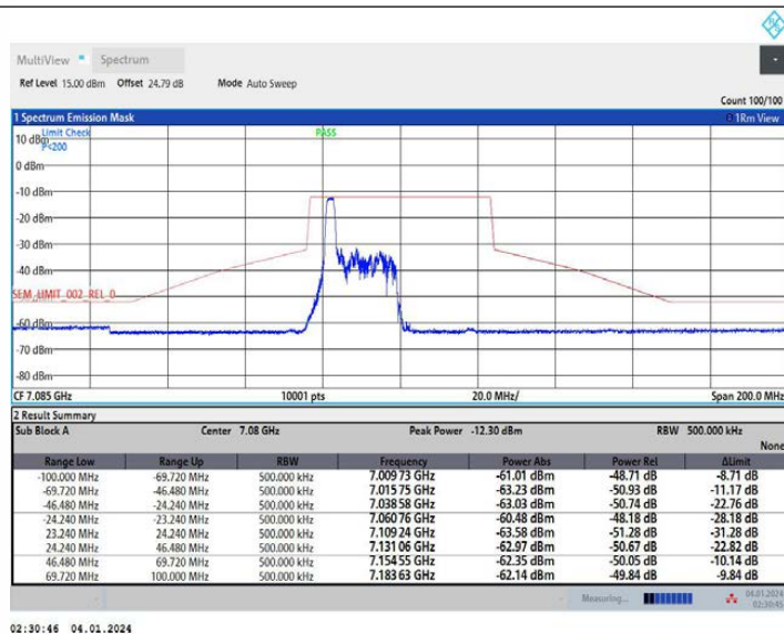
11AX40MIMO Ant1 7085 52Tone RU37
