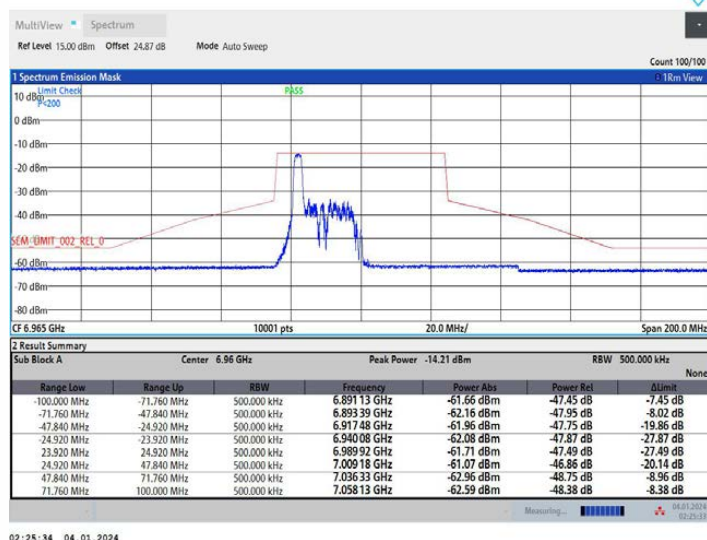
11AX40MIMO Ant1 6965 52Tone RU37
