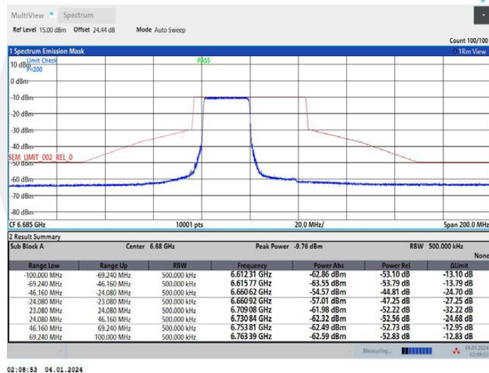
11AX40MIMO_Ant1_6685_26Tone_RU0
