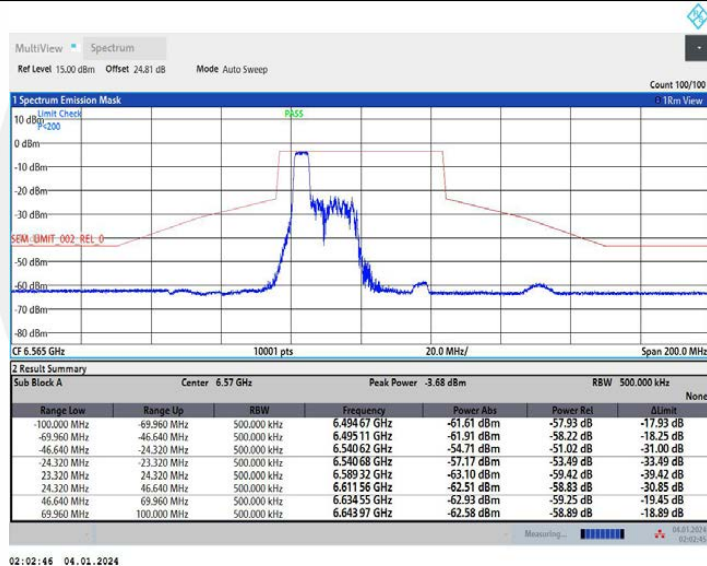
11AX40MIMO_Ant2_6565_106Tone_RU53
