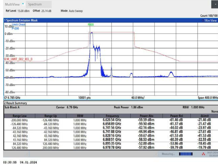
11AX80MIMO_Ant1_6785_106Tone_RU53
