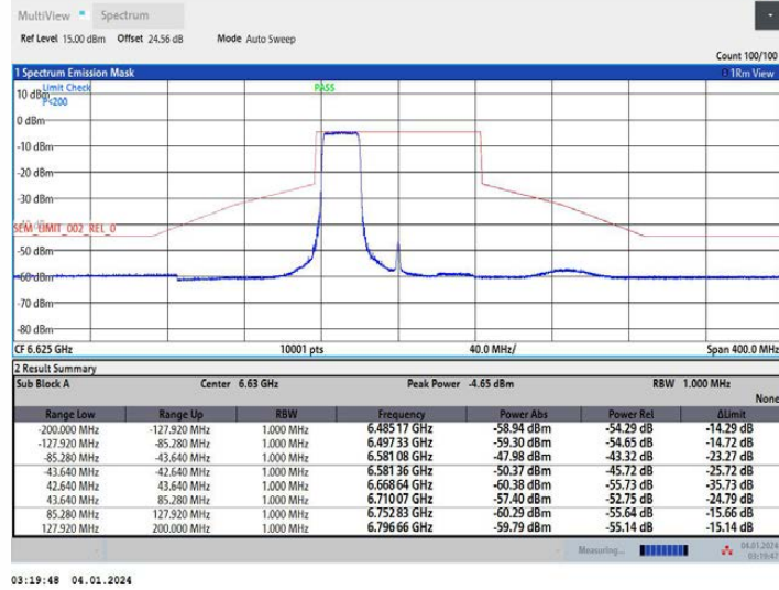
11AX80MIMO_Ant1_6625_484Tone_RU65
