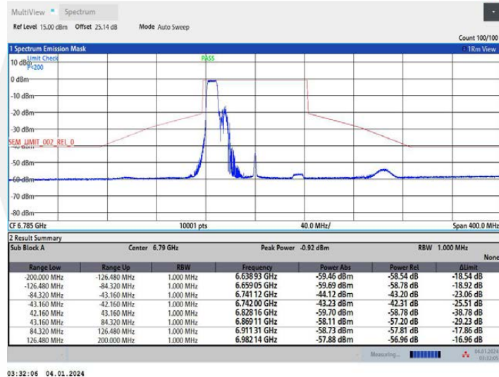
11AX80MIMO_Ant1_6785_242Tone_RU61
