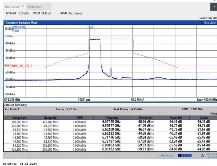
11AX80MIMO_Ant2_6705_484Tone_RU65
