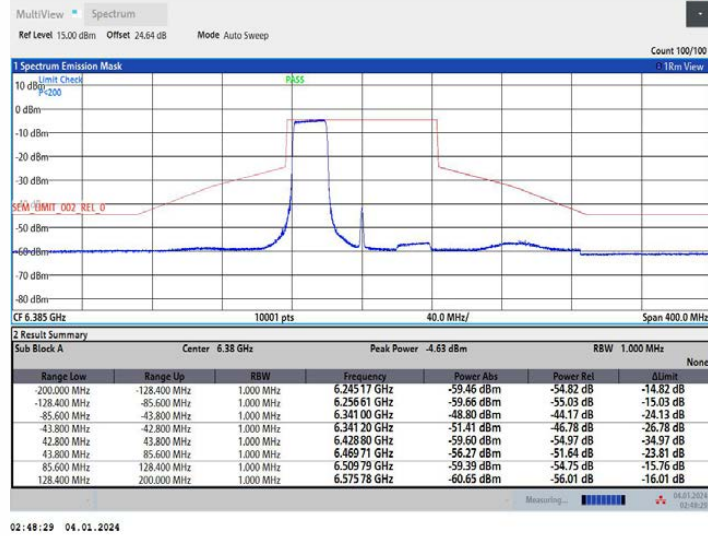
11AX80MIMO_Ant1_6385_484Tone_RU65
