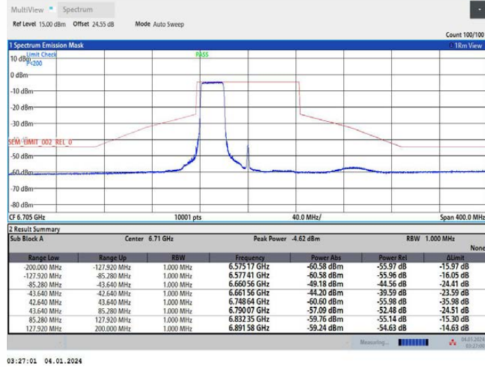
11AX80MIMO_Ant1_6705_484Tone_RU65
