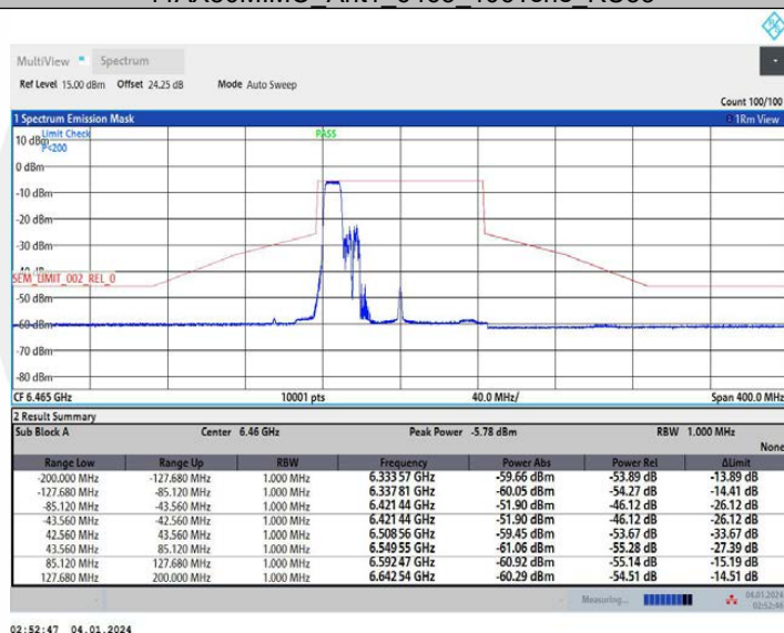
11AX80MIMO_Ant1_6465_242Tone_RU61
