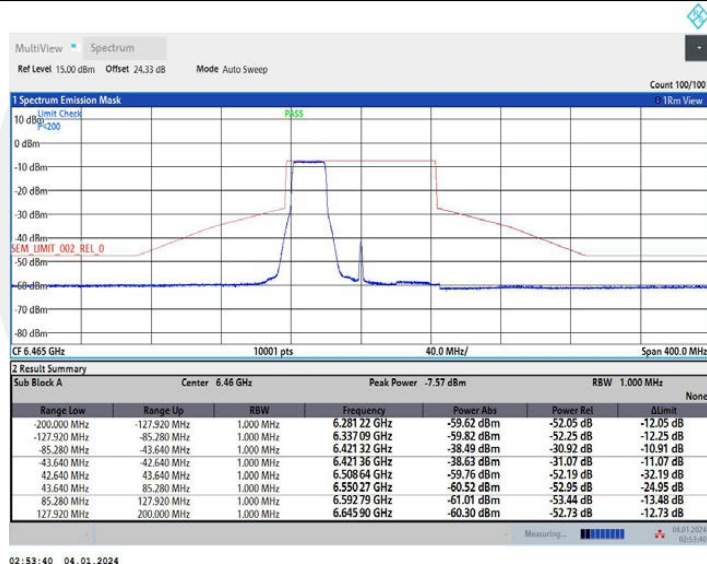
11AX80MIMO_Ant2_6465_484Tone_RU65
