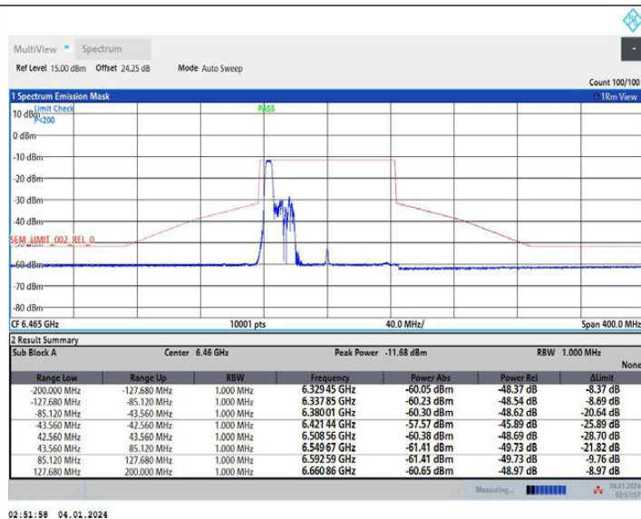
11AX80MIMO_Ant1_6465_106Tone_RU53
