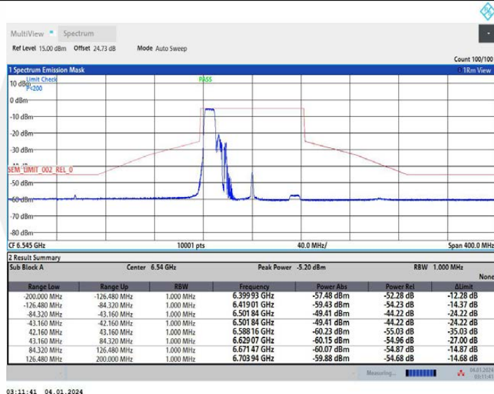
11AX80MIMO_Ant1_6545_242Tone_RU61
