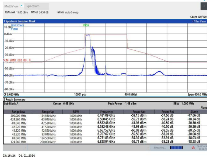
11AX80MIMO_Ant2_6625_242Tone_RU61
