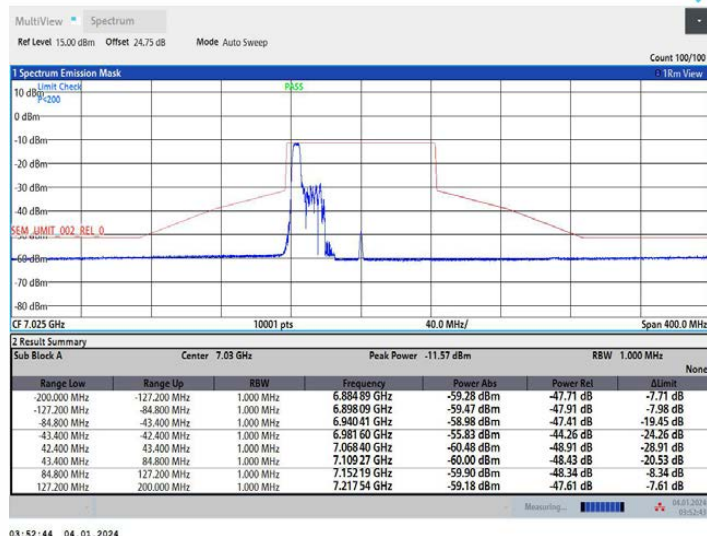
11AX80MIMO_Ant1_7025_106Tone_RU53
