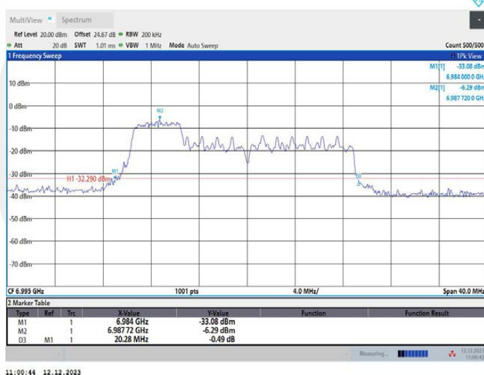
11AX20MIMO_Ant2_6995_106Tone_RU53
