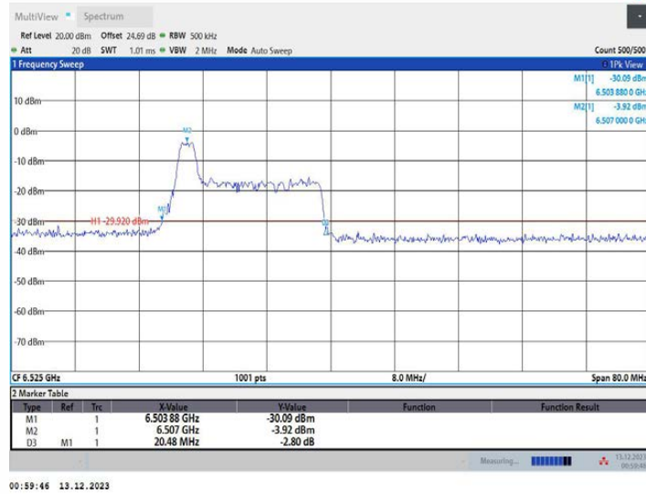
11AX40MIMO_Ant1_6525_52Tone_RU37
