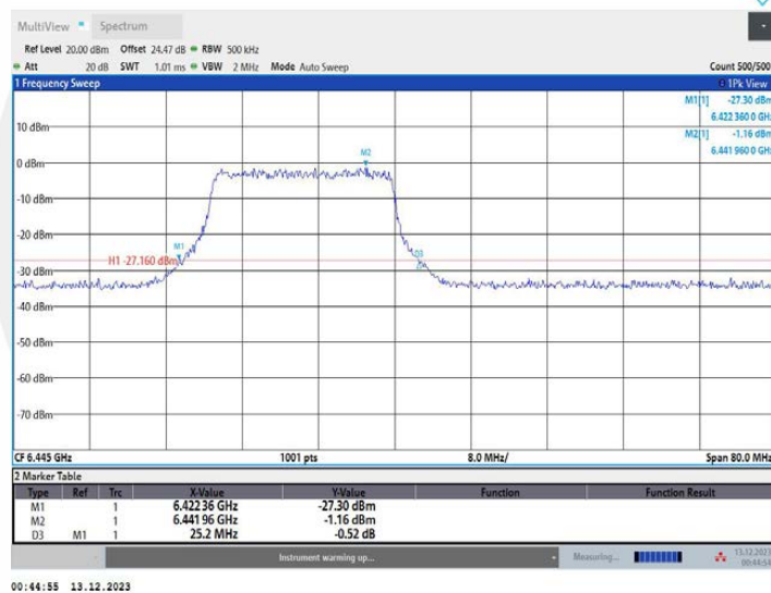
11AX40MIMO_Ant1_6445_26Tone_RU0
