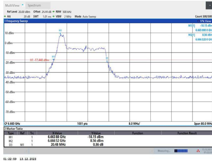
11AX40MIMO_Ant2_6685_52Tone_RU37
