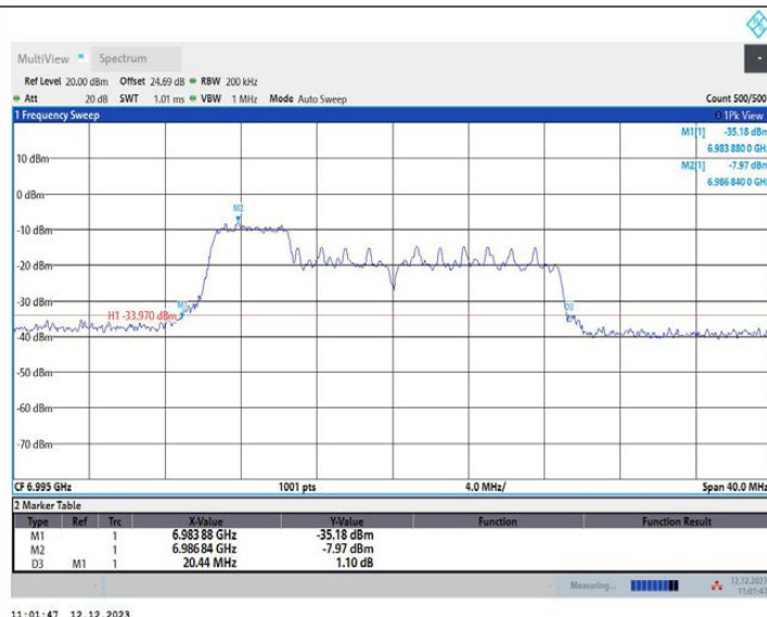
11AX20MIMO_Ant1_6995_106Tone_RU53
