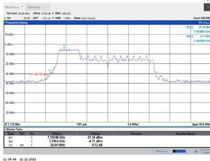
11AX20MIMO_Ant2_7115_106Tone_RU53
