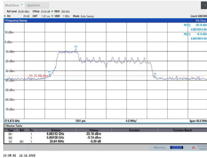
11AX20MIMO_Ant1_6875_106Tone_RU53
