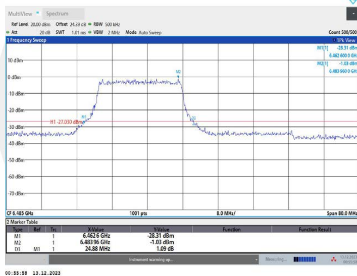
11AX40MIMO_Ant1_6485_26Tone_RU0
