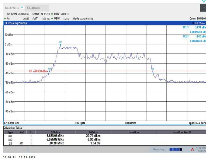
11AX20MIMO_Ant2_6695_106Tone_RU53
