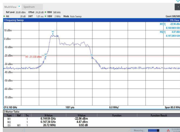
11AX40MIMO_Ant1_6165_106Tone_RU53
