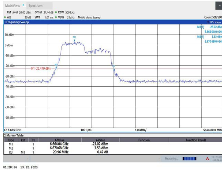
11AX40MIMO_Ant2_6685_242Tone_RU61
