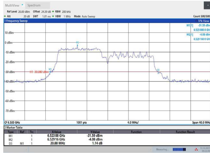
11AX20MIMO_Ant1_6535_26Tone_RU0
