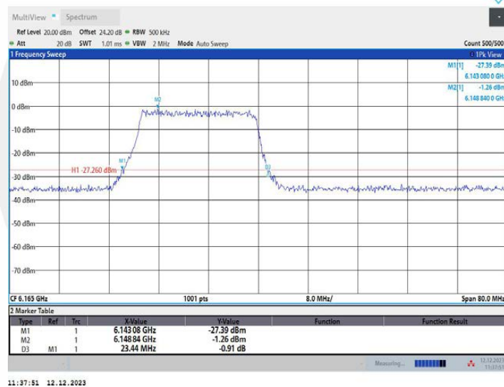
11AX40MIMO_Ant1_6165_26Tone_RU0
