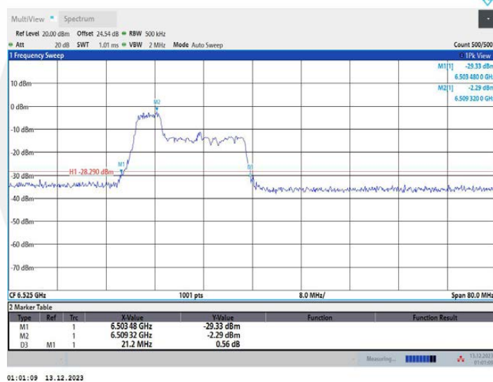
11AX40MIMO_Ant2_6525_106Tone_RU53
