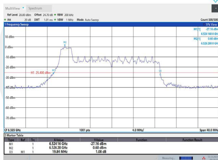
11AX20MIMO_Ant1_6535_52Tone_RU37
