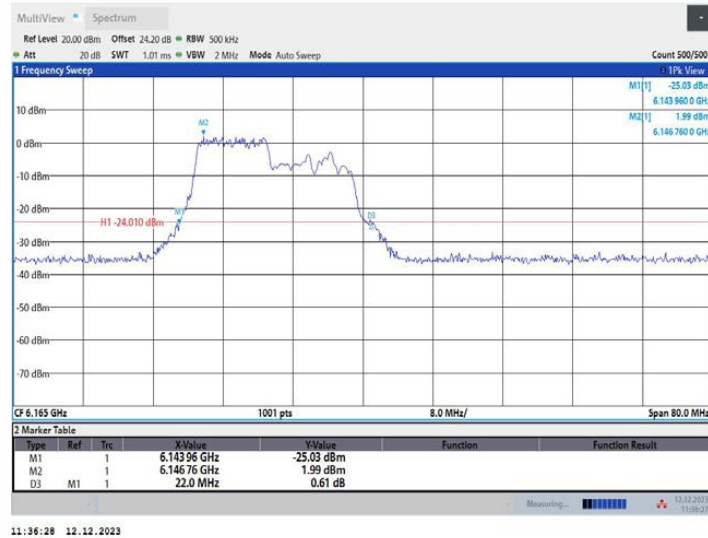
11AX40MIMO_Ant1_6165_242Tone_RU61
