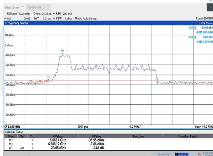
11AX20MIMO_Ant1_6895_52Tone_RU37
