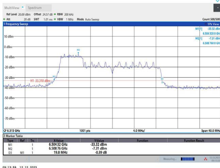
11AX20MIMO_Ant1_6515_106Tone_RU53
