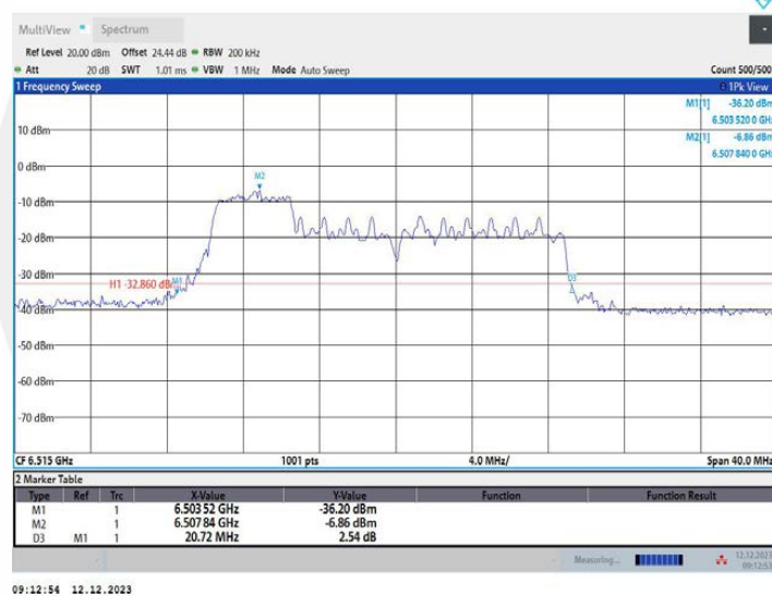
11AX20MIMO_Ant2_6515_106Tone_RU53
