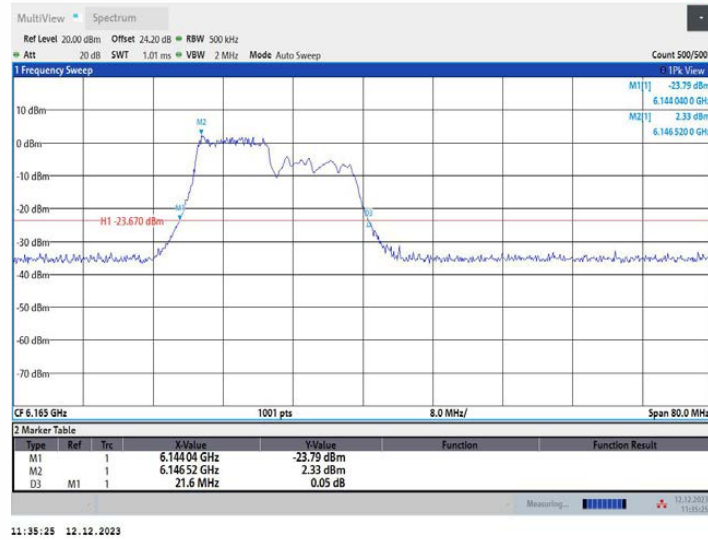
11AX40MIMO_Ant2_6165_242Tone_RU61
