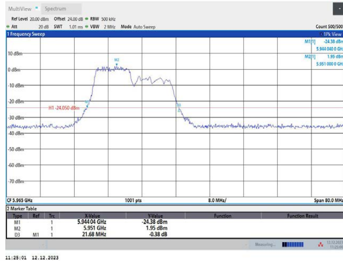
11AX40MIMO_Ant2_5965_242Tone_RU61
