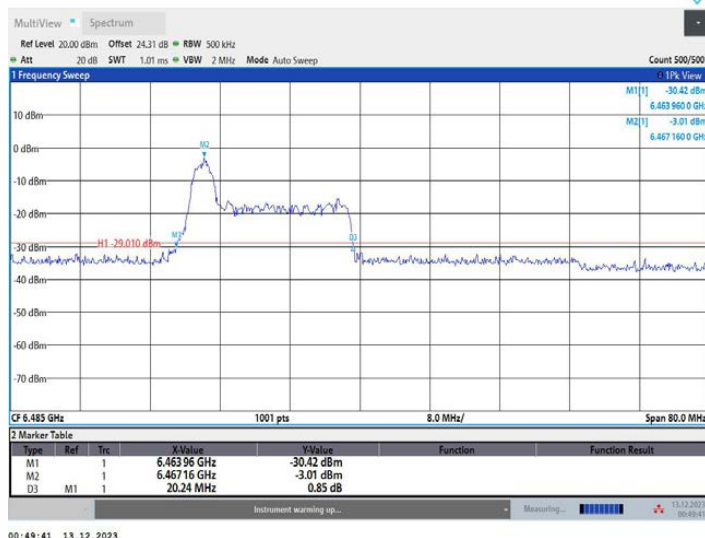
11AX40MIMO_Ant1_6485_52Tone_RU37
