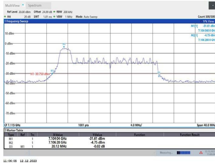
11AX20MIMO_Ant2_7115_52Tone_RU37
