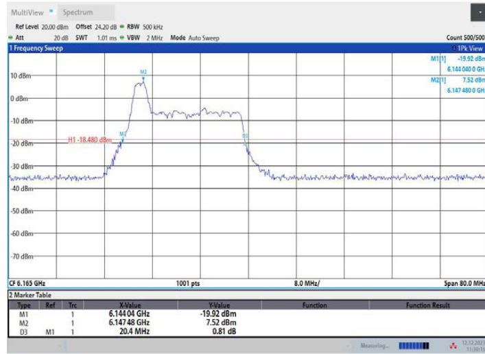
11AX40MIMO_Ant2_6165_52Tone_RU37
