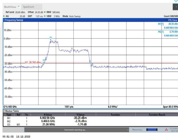
11AX40MIMO_Ant2_6485_106Tone_RU53
