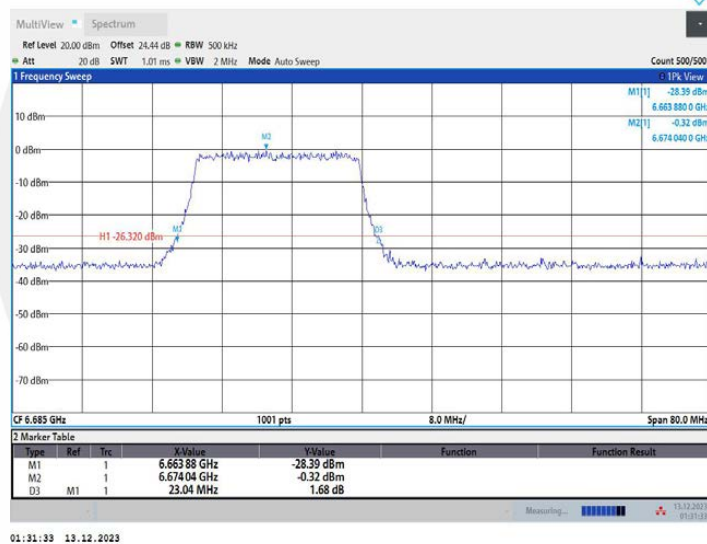
11AX40MIMO_Ant1_6685_26Tone_RU0
