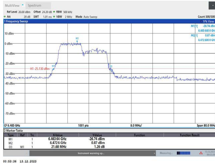
11AX40MIMO_Ant2_6485_242Tone_RU61
