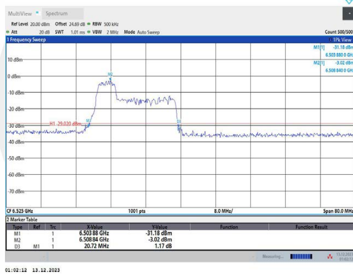
11AX40MIMO_Ant1_6525_106Tone_RU53
