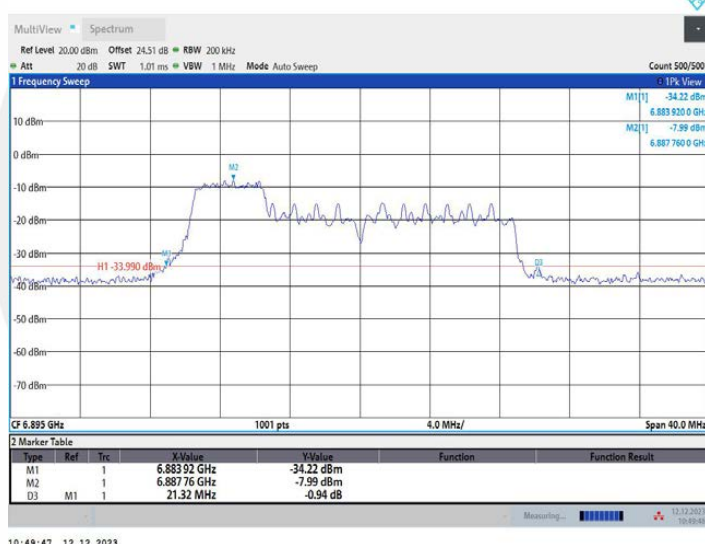
11AX20MIMO_Ant2_6895_106Tone_RU53
