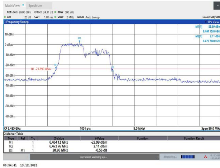
11AX40MIMO_Ant1_6485_242Tone_RU61
