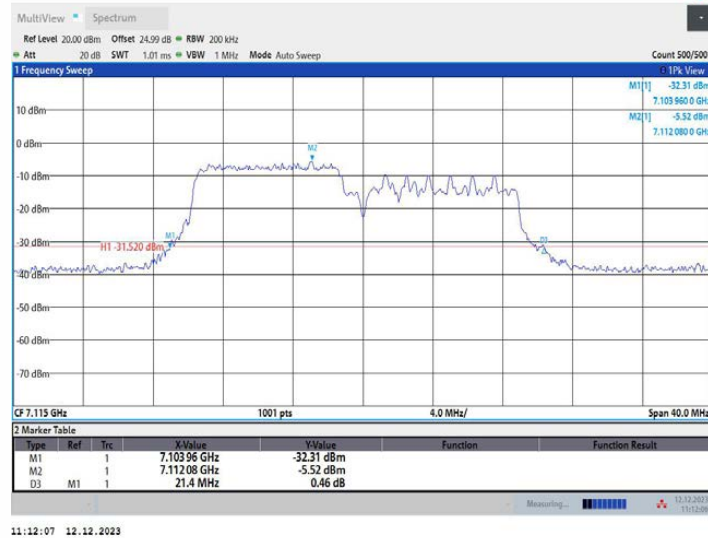
11AX20MIMO_Ant1_7115_26Tone_RU0
