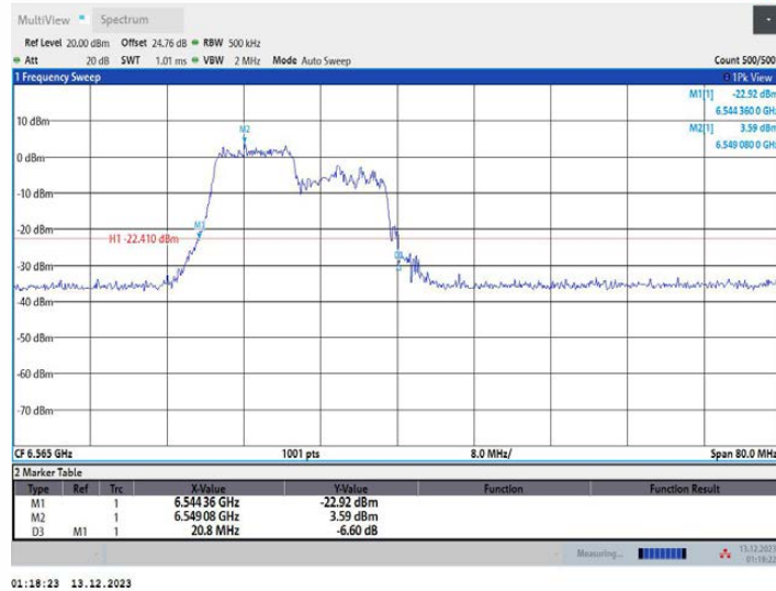
11AX40MIMO_Ant1_6565_242Tone_RU61
