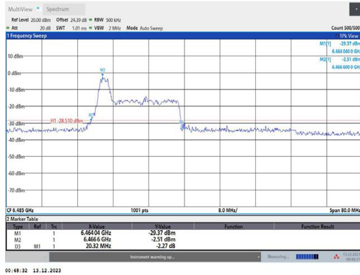
11AX40MIMO_Ant2_6485_52Tone_RU37
