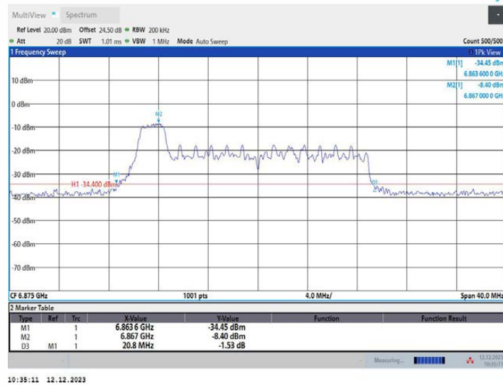
11AX20MIMO_Ant2_6875_52Tone_RU37
