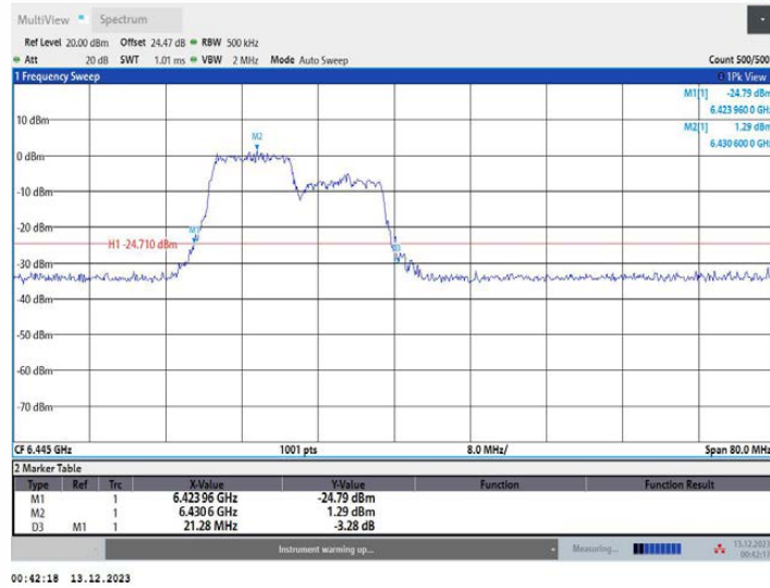
11AX40MIMO_Ant2_6445_242Tone_RU61
