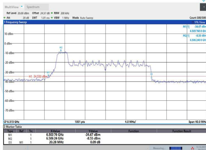
11AX20MIMO_Ant1_6515_52Tone_RU37
