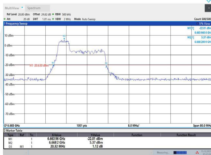
11AX40MIMO_Ant1_6685_106Tone_RU53
