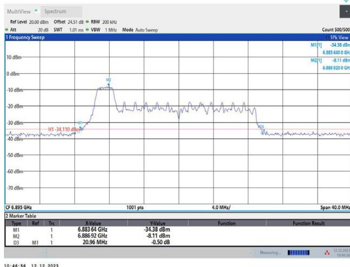
11AX20MIMO_Ant2_6895_52Tone_RU37
