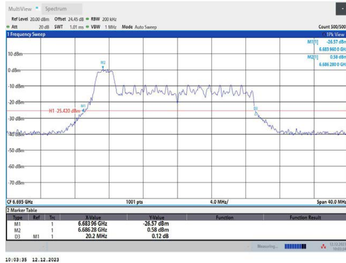
11AX20MIMO_Ant2_6695_52Tone_RU37
