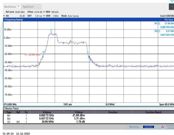
11AX40MIMO_Ant2_6685_106Tone_RU53
