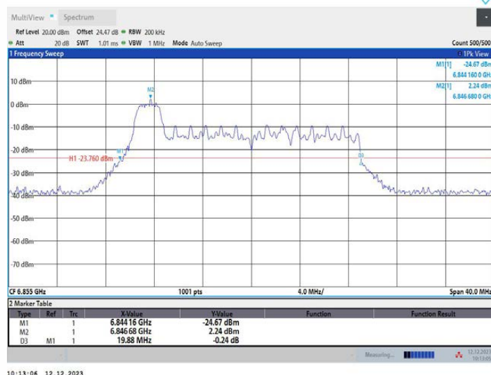
11AX20MIMO_Ant2_6855_52Tone_RU37
