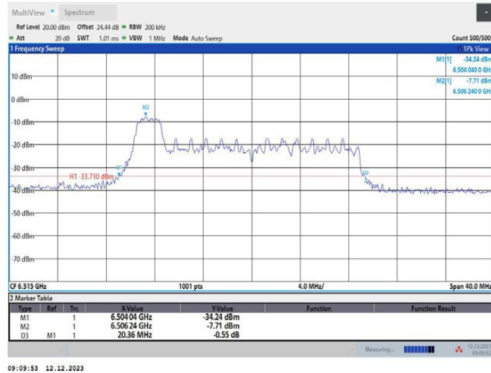
11AX20MIMO_Ant2_6515_52Tone_RU37
