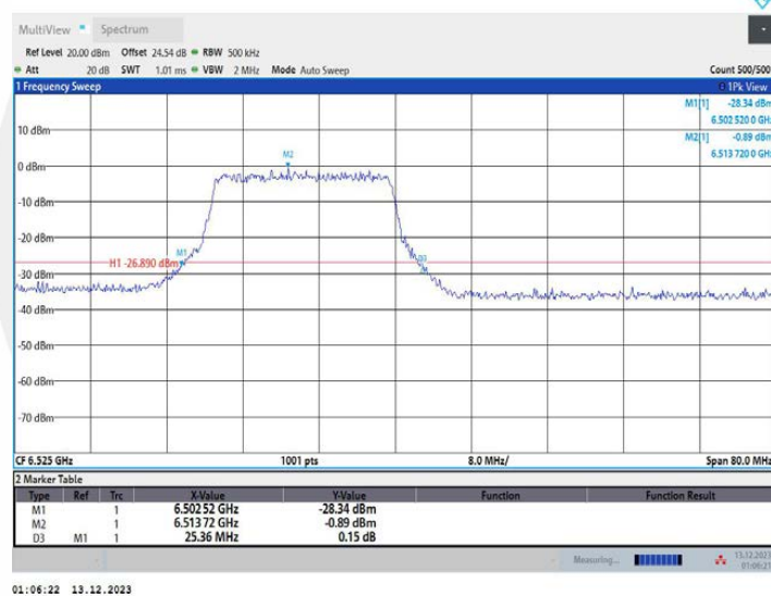
11AX40MIMO_Ant1_6525_26Tone_RU0
