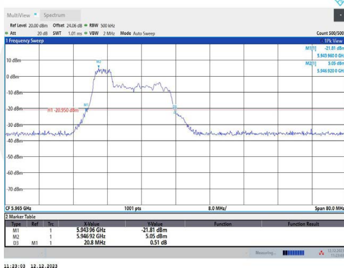
11AX40MIMO_Ant1_5965_106Tone_RU53
