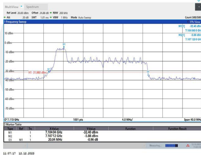
11AX20MIMO_Ant1_7115_52Tone_RU37
