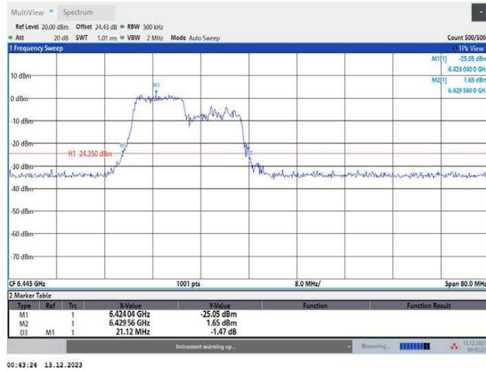
11AX40MIMO_Ant1_6445_242Tone_RU61
