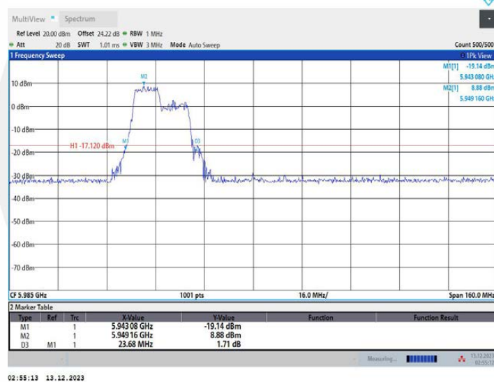
11AX80MIMO_Ant1_5985_242Tone_RU61
