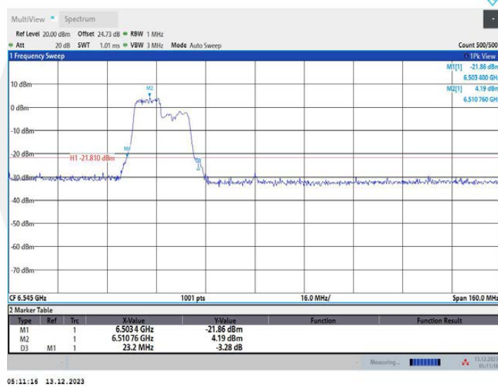
11AX80MIMO_Ant1_6545_242Tone_RU61
