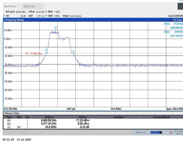
11AX80MIMO_Ant1_6705_242Tone_RU61
