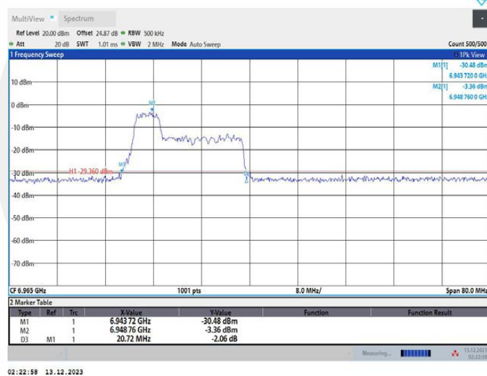
11AX40MIMO_Ant1_6965_106Tone_RU53
