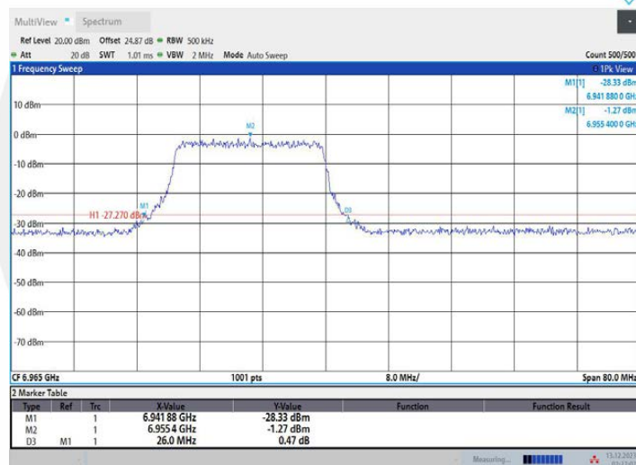
11AX40MIMO_Ant1_6965_26Tone_RU0
