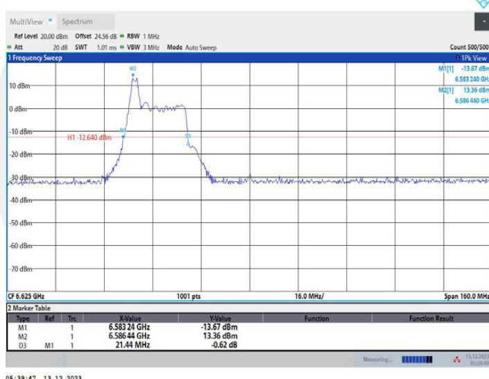
11AX80MIMO_Ant1_6625_52Tone_RU37
