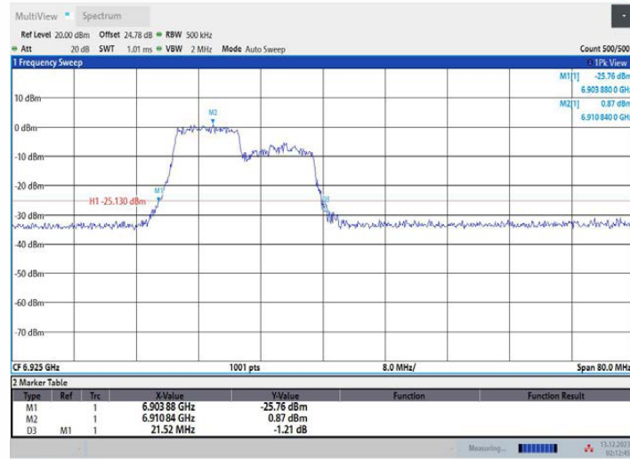
11AX40MIMO_Ant2_6925_242Tone_RU61
