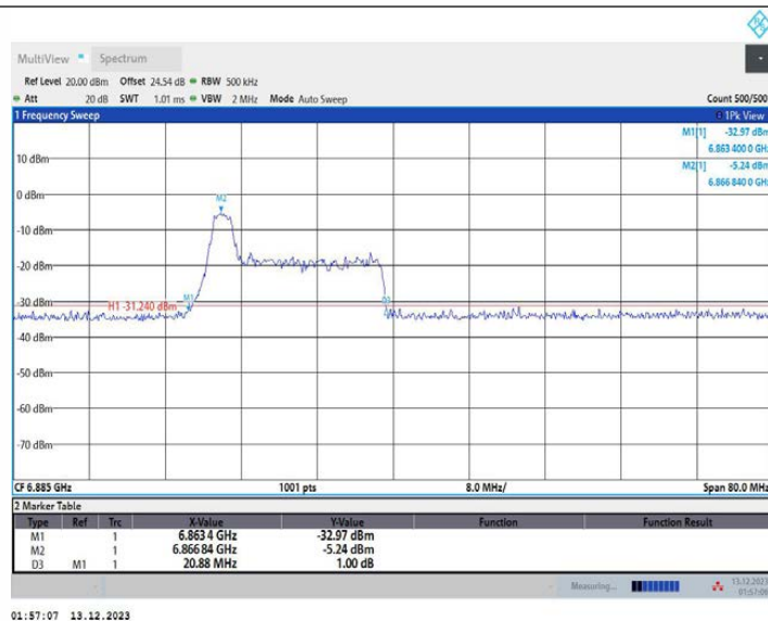
11AX40MIMO_Ant1_6885_52Tone_RU37
