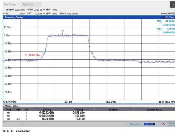
11AX80MIMO_Ant1_6465_26Tone_RU0
