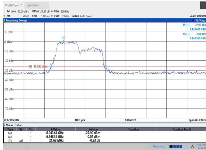
11AX40MIMO_Ant2_6965_242Tone_RU61
