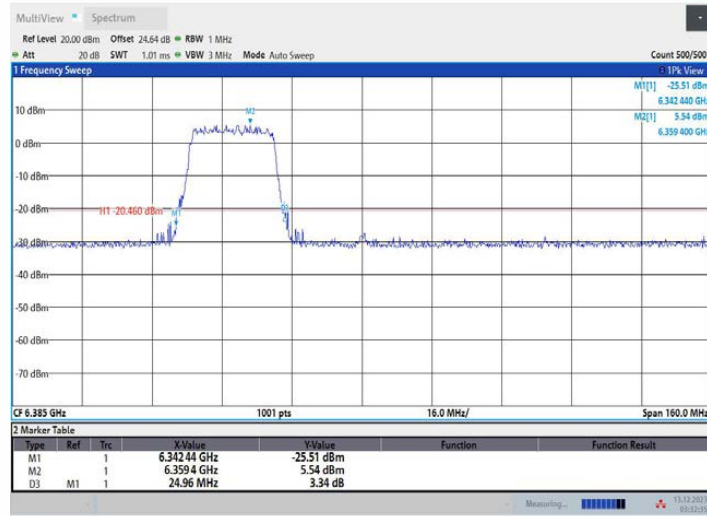
11AX80MIMO_Ant1_6385_484Tone_RU65
