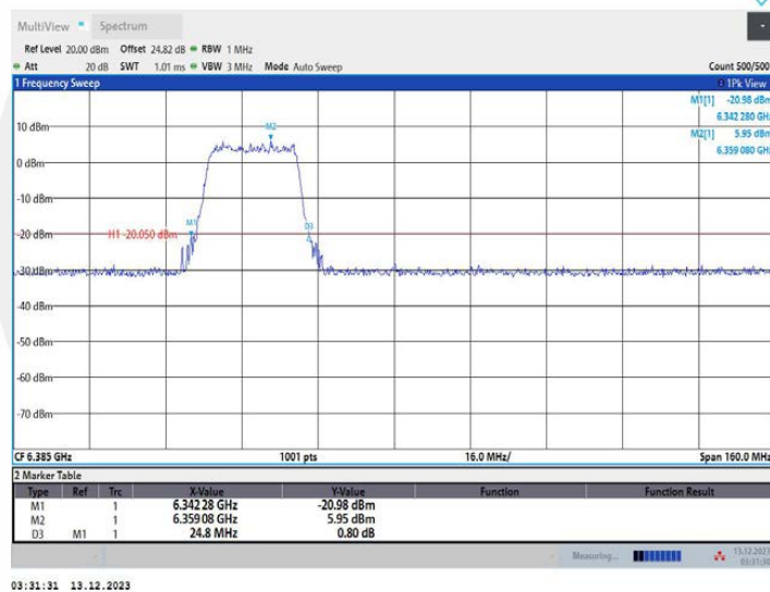
11AX80MIMO_Ant2_6385_484Tone_RU65
