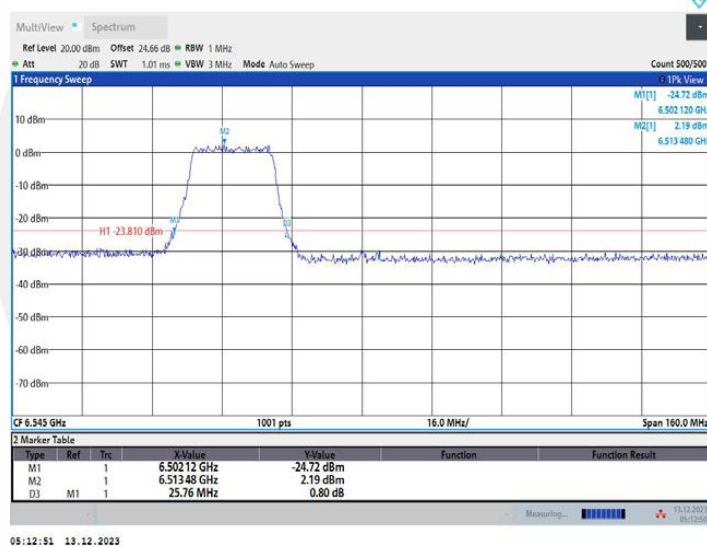
11AX80MIMO_Ant2_6545_484Tone_RU65
