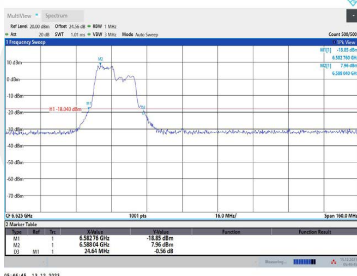
11AX80MIMO_Ant1_6625_242Tone_RU61
