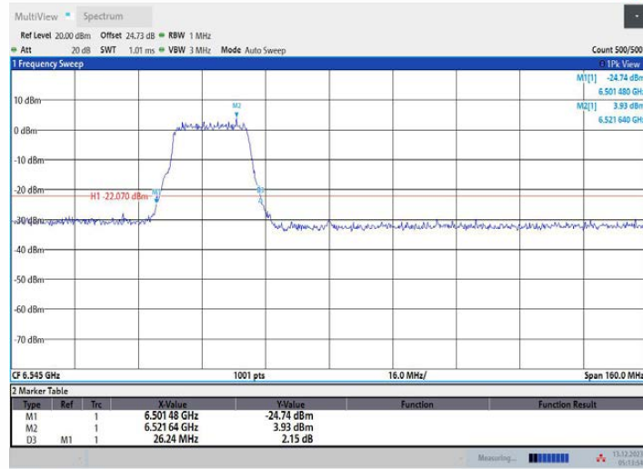
11AX80MIMO_Ant1_6545_484Tone_RU65
