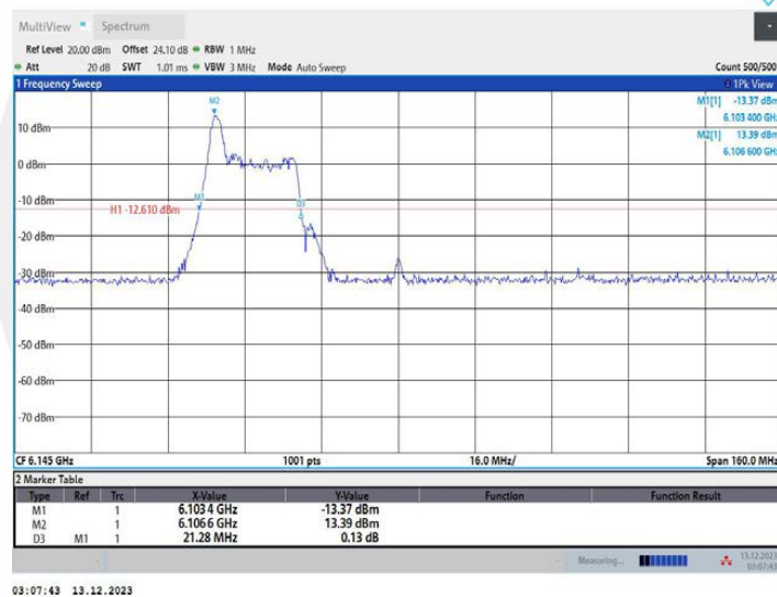
11AX80MIMO_Ant1_6145_52Tone_RU37
