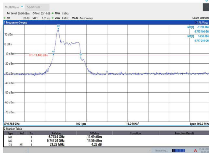
11AX80MIMO_Ant1_6785_52Tone_RU37
