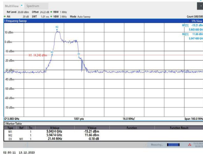
11AX80MIMO_Ant1_5985_106Tone_RU53
