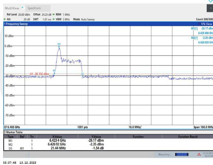
11AX80MIMO_Ant1_6465_52Tone_RU37
