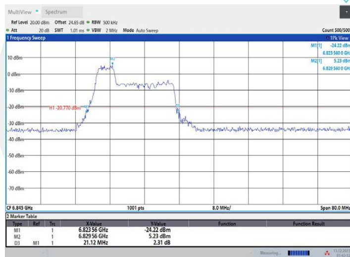
11AX40MIMO_Ant1_6845_106Tone_RU53
