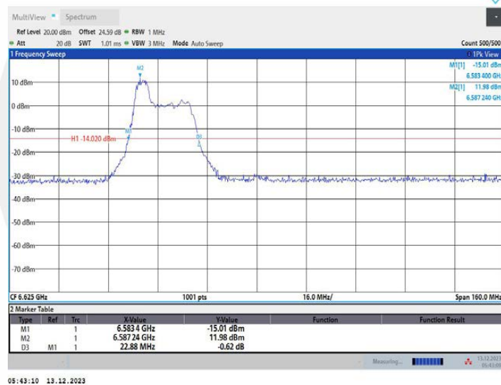
11AX80MIMO_Ant2_6625_106Tone_RU53
