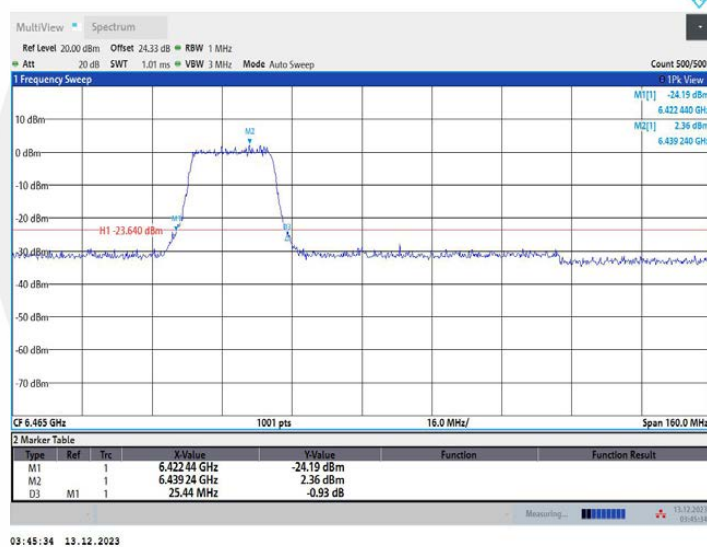
11AX80MIMO_Ant2_6465_484Tone_RU65
