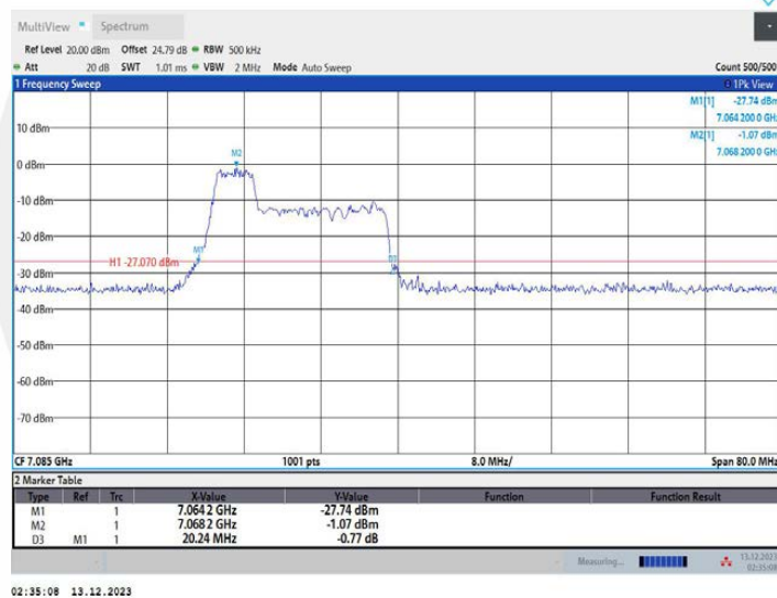
11AX40MIMO_Ant1_7085_106Tone_RU53
