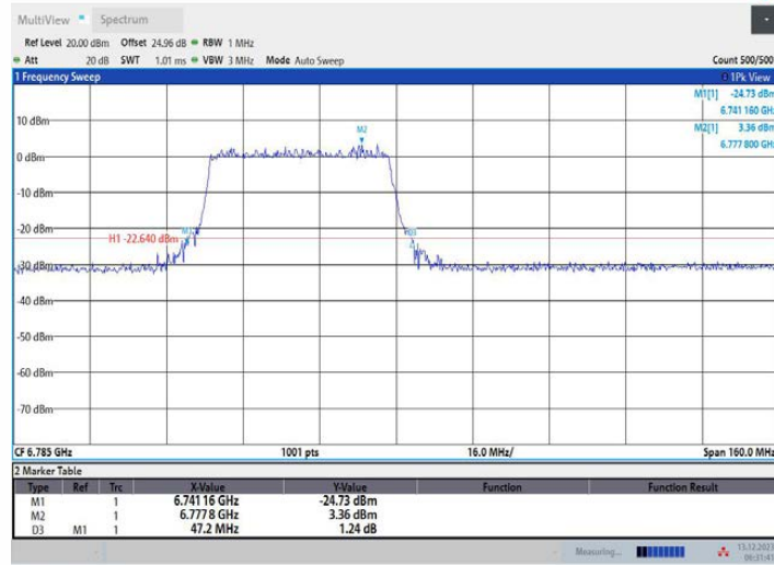
11AX80MIMO_Ant1_6785_26Tone_RU0
