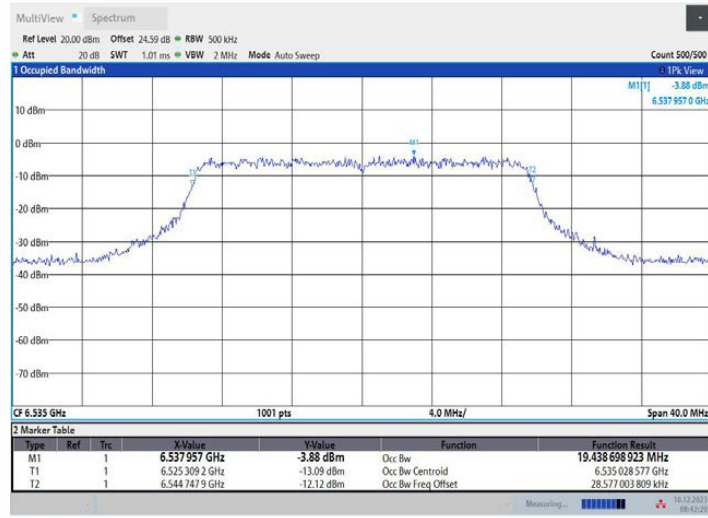
11AX20MIMO_Ant1_6535
