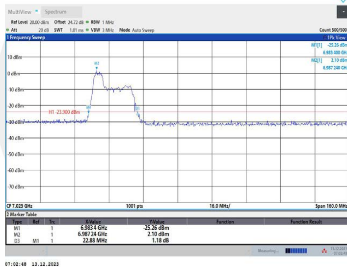
11AX80MIMO_Ant2_7025_106Tone_RU53
