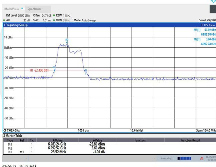
11AX80MIMO_Ant1_7025_242Tone_RU61
