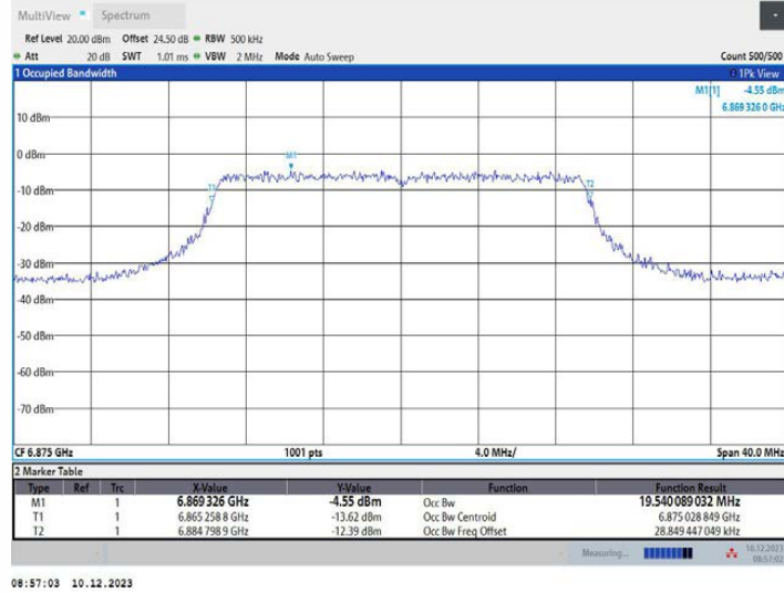
11AX20MIMO_Ant1_6875
