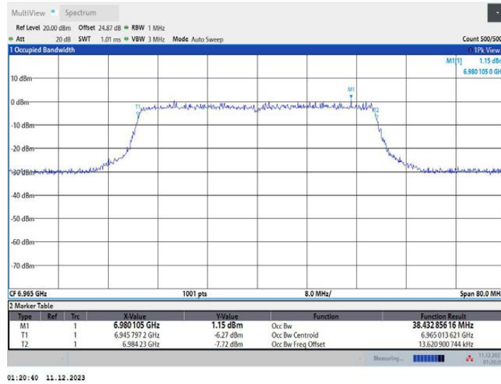
11AX40MIMO_Ant1_6965
