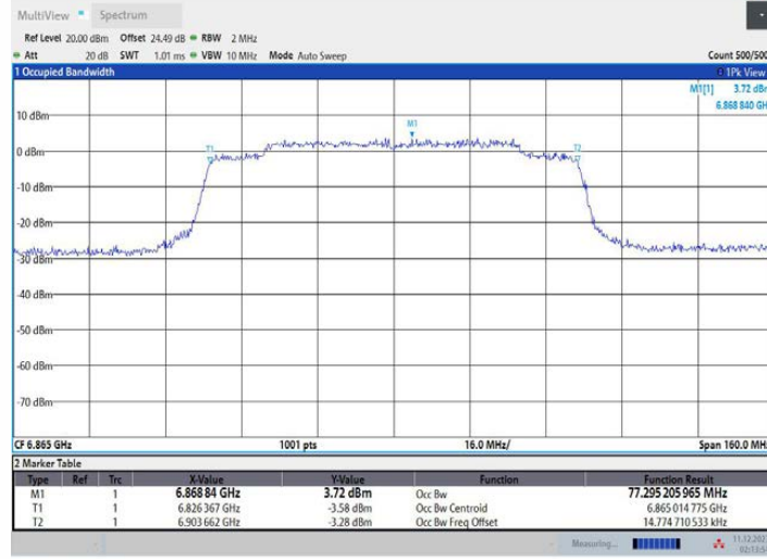
11AX80MIMO_Ant1_6865
