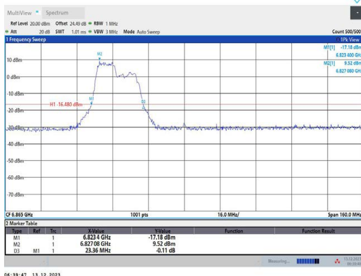
11AX80MIMO_Ant2_6865_242Tone_RU61
