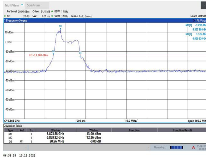
11AX80MIMO_Ant1_6865_106Tone_RU53
