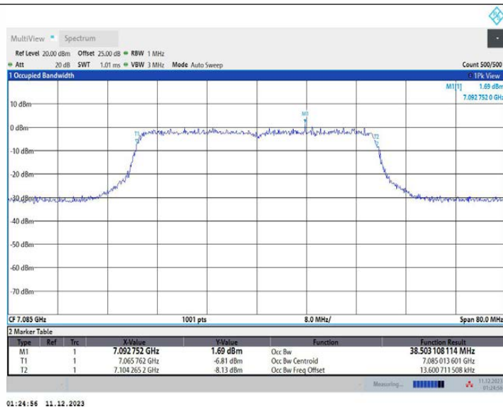
11AX40MIMO_Ant1_7085
