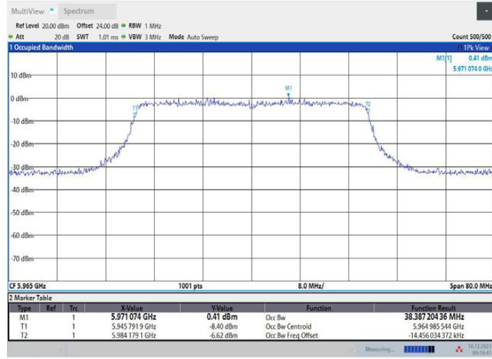
11AX40MIMO_Ant1_5965
