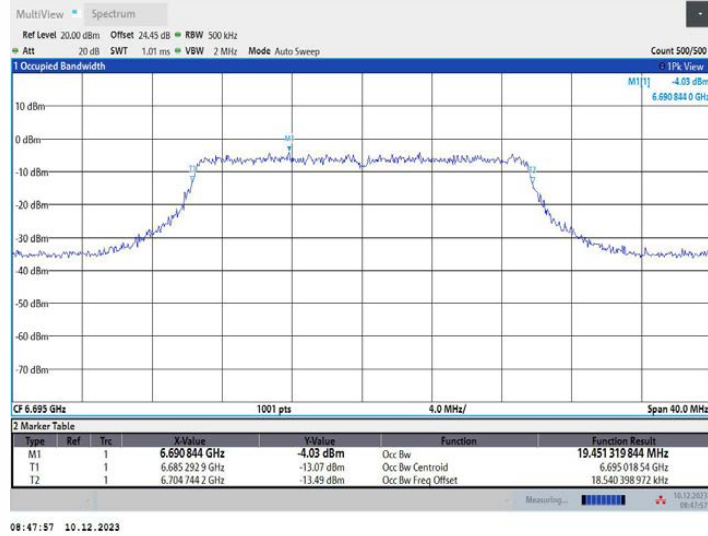
11AX20MIMO_Ant1_6695
