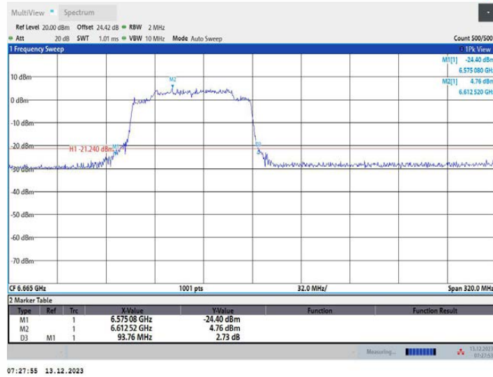
11AX160MIMO_Ant1_6665_996Tone_RU67
