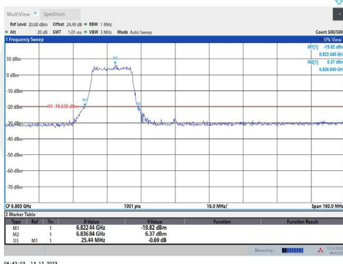
11AX80MIMO_Ant2_6865_484Tone_RU65
