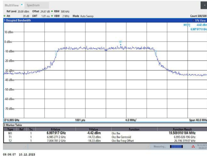
11AX20MIMO_Ant1_6995
