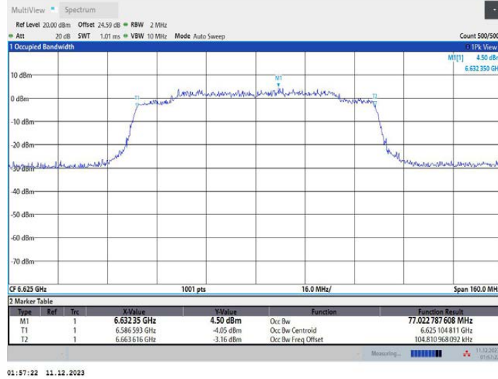
11AX80MIMO_Ant1_6625
