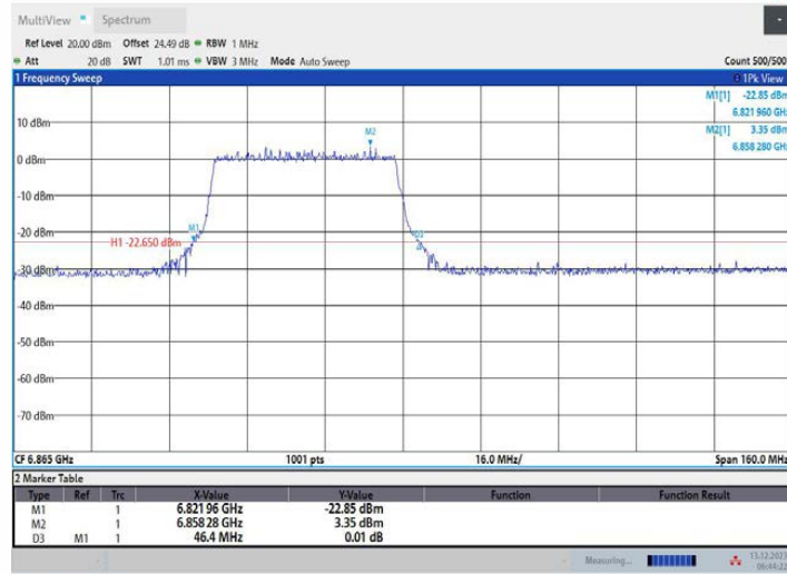
11AX80MIMO_Ant1_6865_26Tone_RU0
