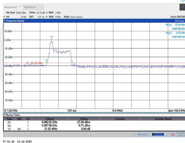
11AX80MIMO_Ant1_7025_52Tone_RU37
