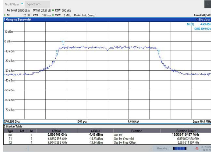
11AX20MIMO_Ant1_6895
