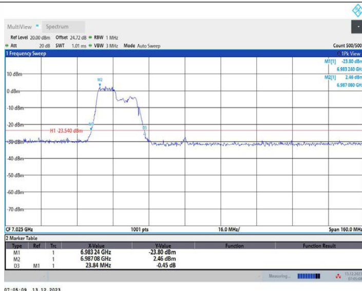
11AX80MIMO_Ant2_7025_242Tone_RU61
