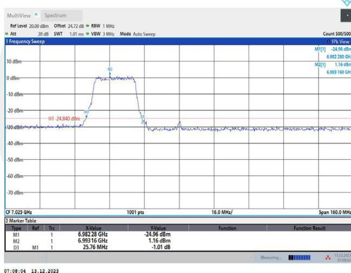
11AX80MIMO_Ant2_7025_484Tone_RU65
