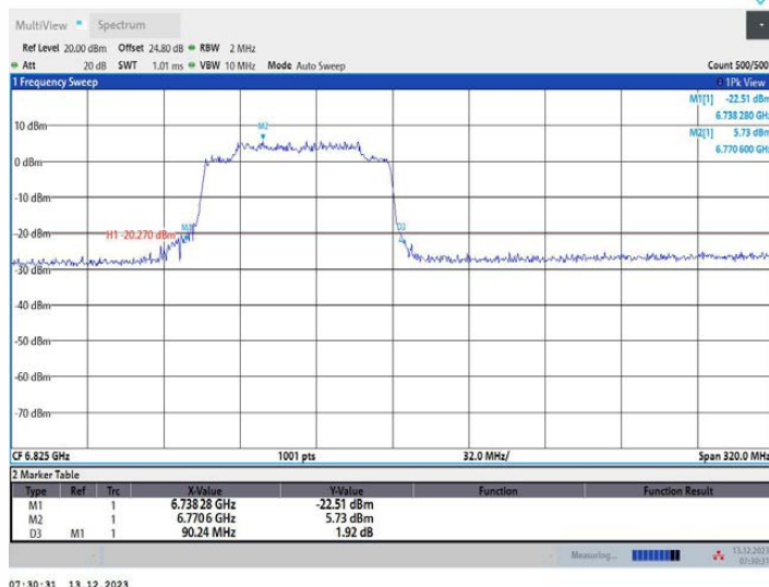
11AX160MIMO_Ant1_6825_996Tone_RU67
