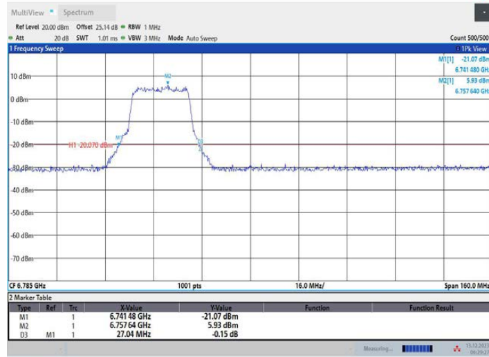
11AX80MIMO_Ant1_6785_484Tone_RU65
