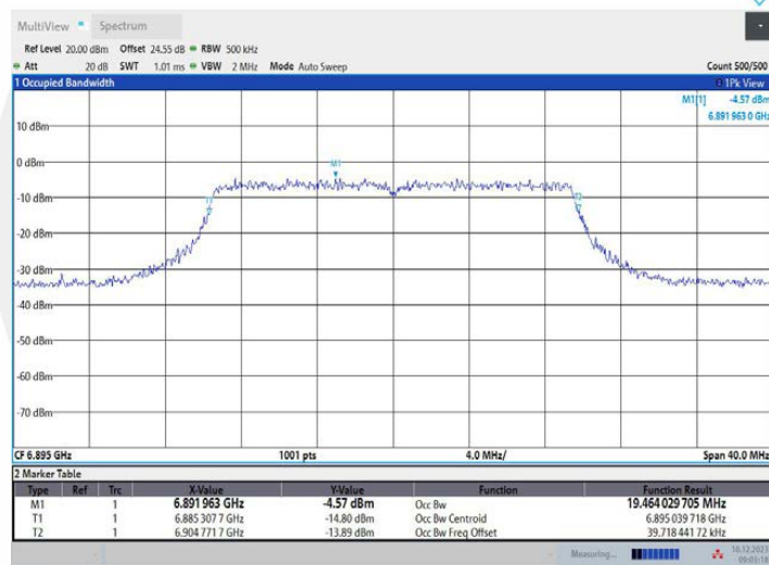
11AX20MIMO_Ant2_6895
