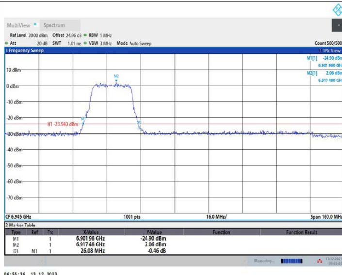
11AX80MIMO_Ant1_6945_484Tone_RU65
