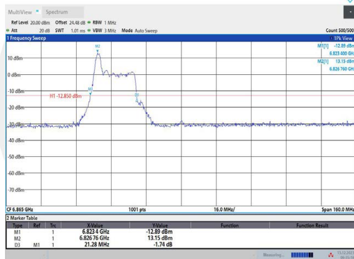
11AX80MIMO_Ant1_6865_52Tone_RU37
