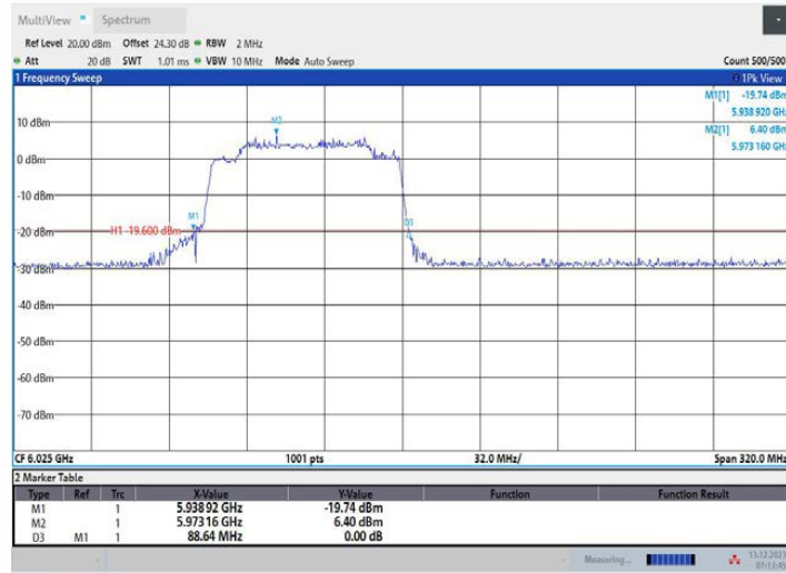
11AX160MIMO_Ant1_6025_996Tone_RU67
