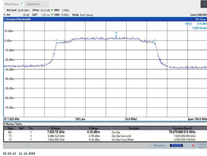
11AX80MIMO_Ant1_7025
