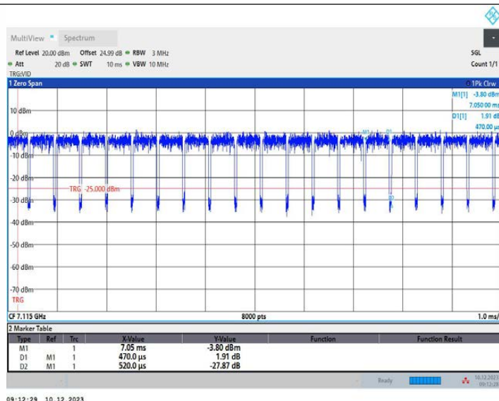
11AX20MIMO_Ant1_7115
