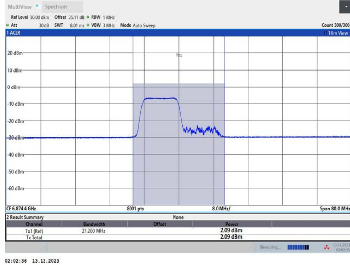
11AX40MIMO_Ant2_6885_242Tone_RU61
