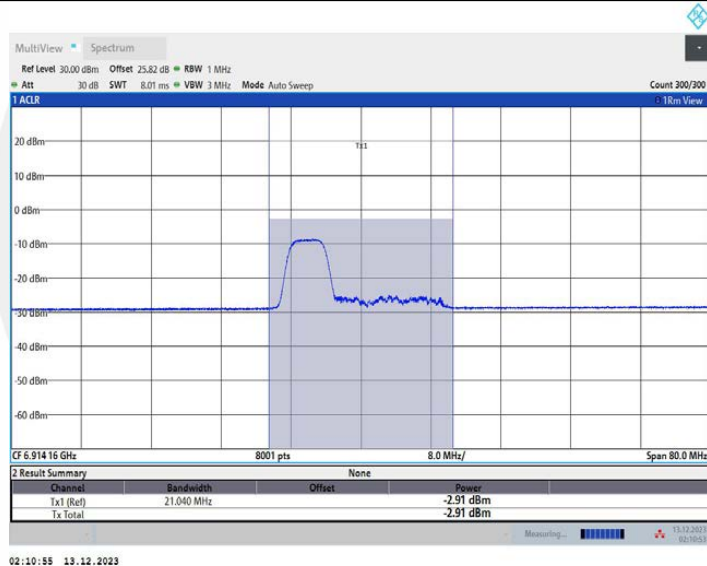
11AX40MIMO_Ant2_6925_106Tone_RU53
