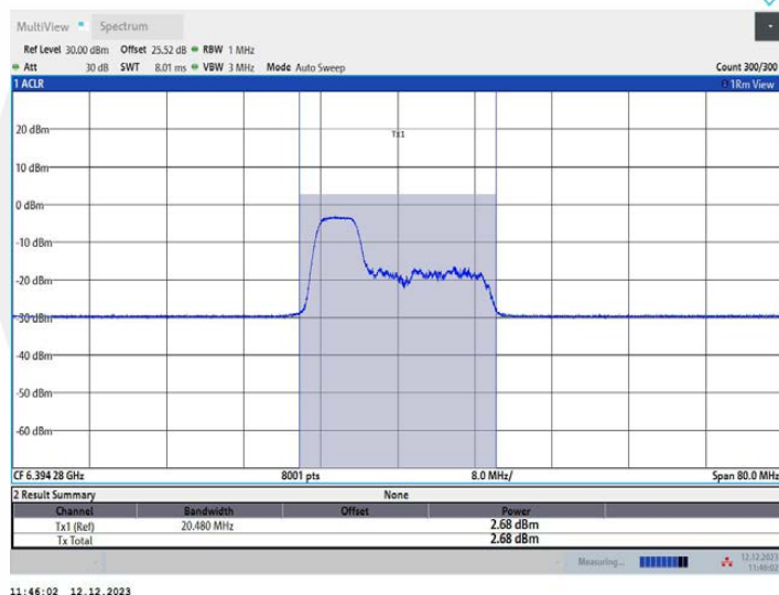
11AX40MIMO_Ant1_6405_106Tone_RU53
