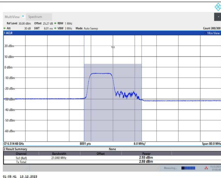
11AX40MIMO_Ant1_6525_242Tone_RU61
