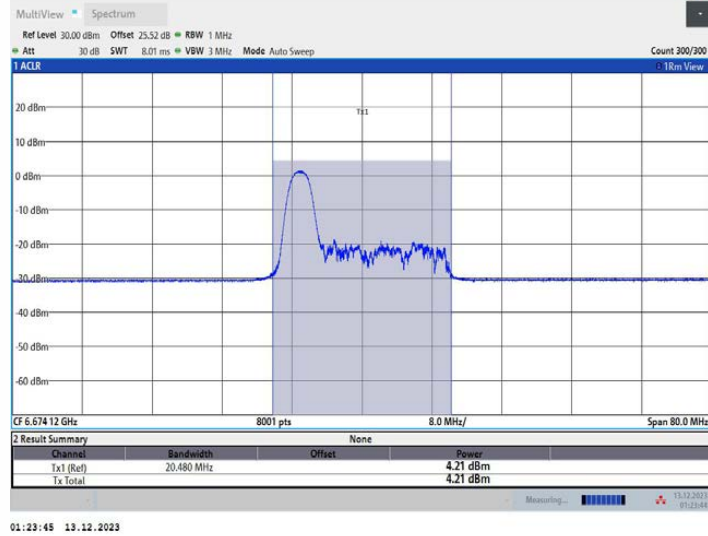
11AX40MIMO_Ant2_6685_52Tone_RU37
