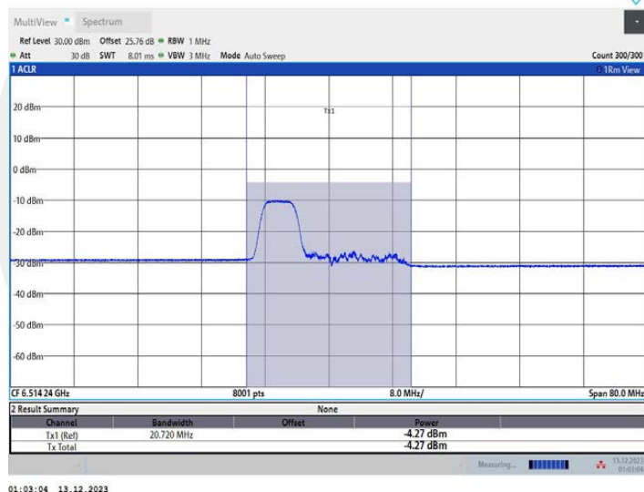
11AX40MIMO_Ant1_6525_106Tone_RU53
