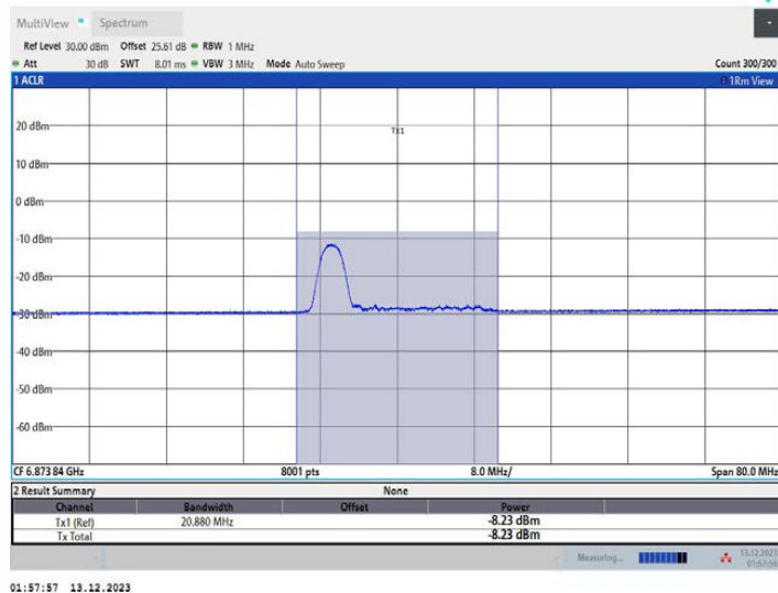
11AX40MIMO_Ant1_6885_52Tone_RU37
