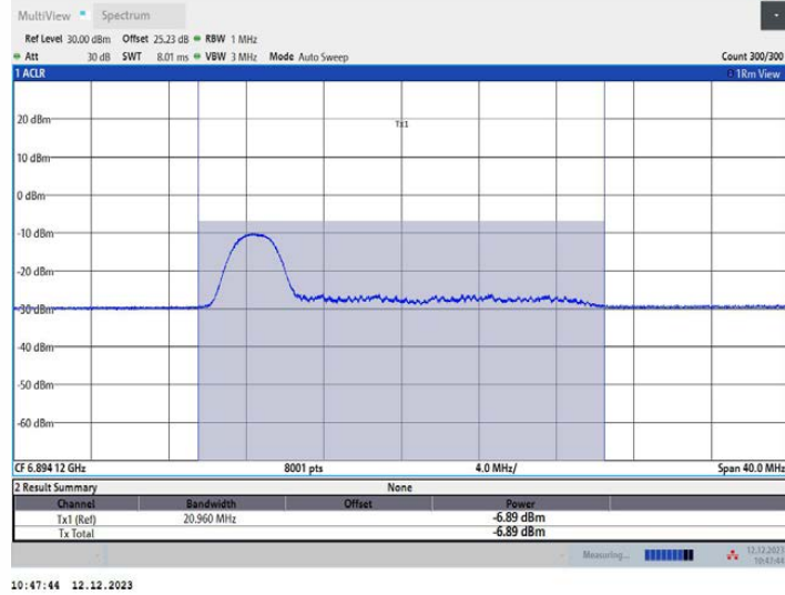
11AX20MIMO_Ant2_6895_52Tone_RU37
