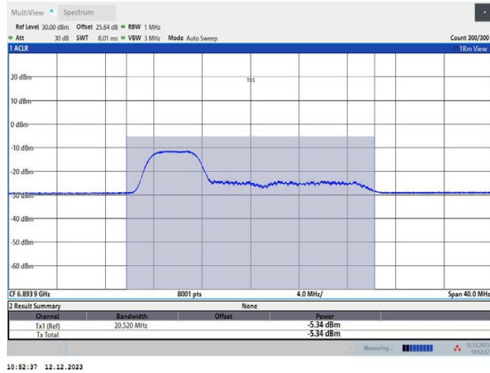
11AX20MIMO_Ant1_6895_106Tone_RU53
