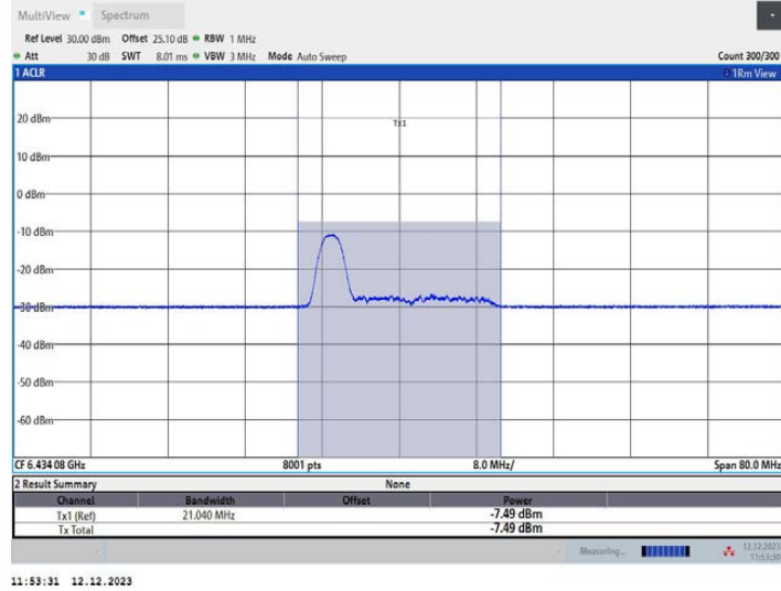
11AX40MIMO_Ant2_6445_52Tone_RU37
