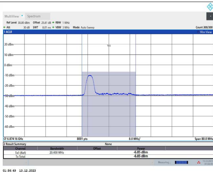
11AX40MIMO_Ant2_6885_52Tone_RU37
