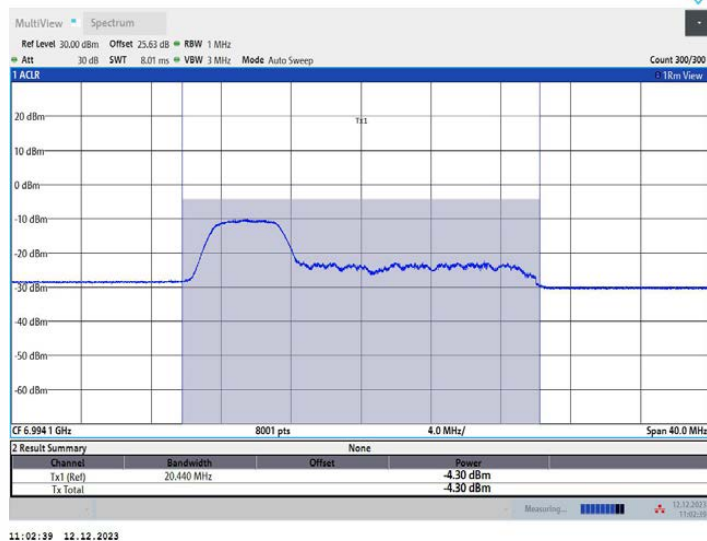
11AX20MIMO_Ant1_6995_106Tone_RU53
