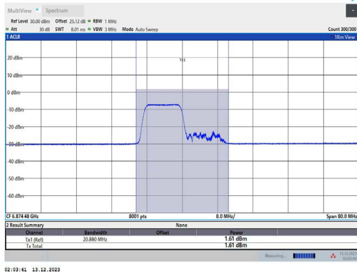
11AX40MIMO_Ant1_6885_242Tone_RU61
