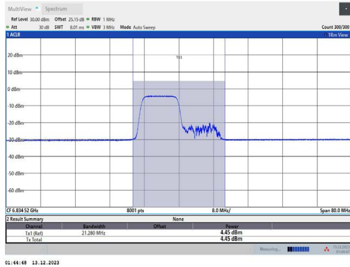
11AX40MIMO_Ant2_6845_242Tone_RU61
