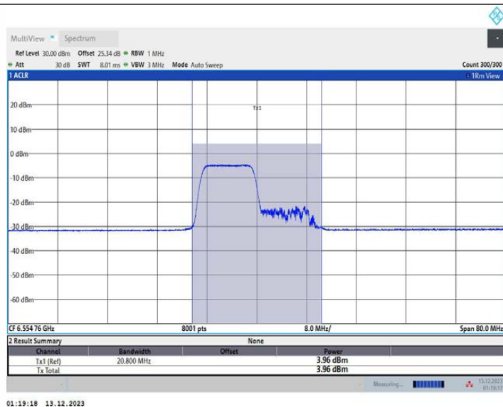
11AX40MIMO_Ant1_6565_242Tone_RU61
