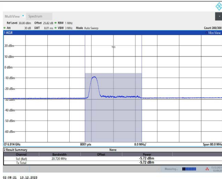
11AX40MIMO_Ant2_6925_52Tone_RU37
