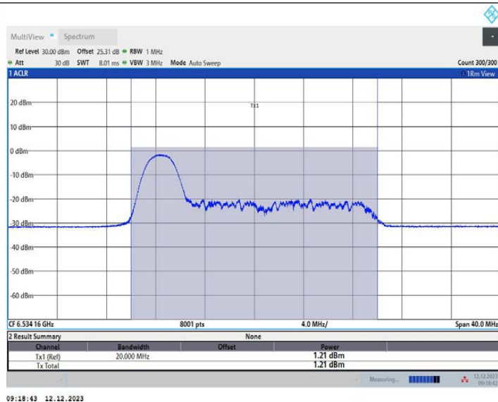
11AX20MIMO_Ant2_6535_52Tone_RU37
