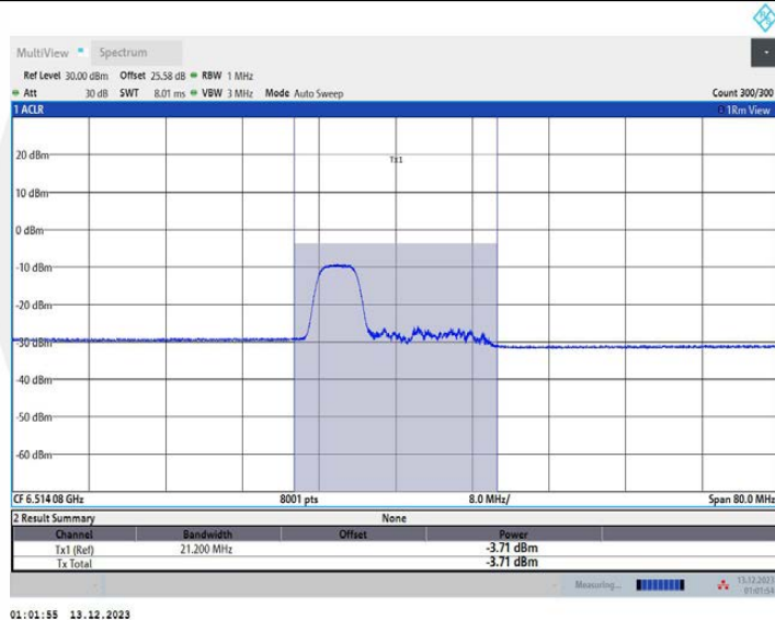
11AX40MIMO_Ant2_6525_106Tone_RU53
