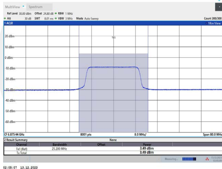
11AX40MIMO_Ant1_6885_26Tone_RU0
