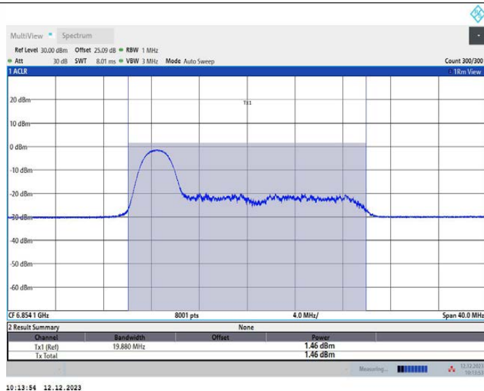
11AX20MIMO_Ant2_6855_52Tone_RU37
