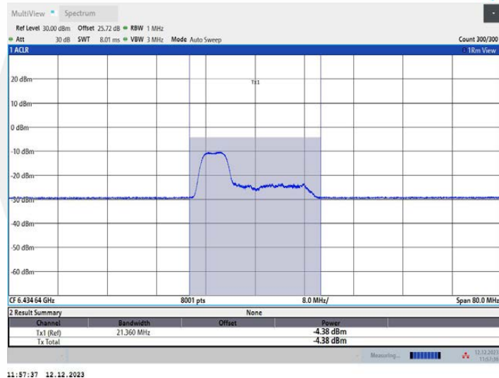
11AX40MIMO_Ant2_6445_106Tone_RU53
