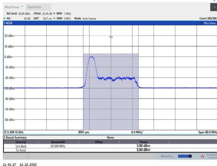
11AX40MIMO_Ant2_6405_52Tone_RU37
