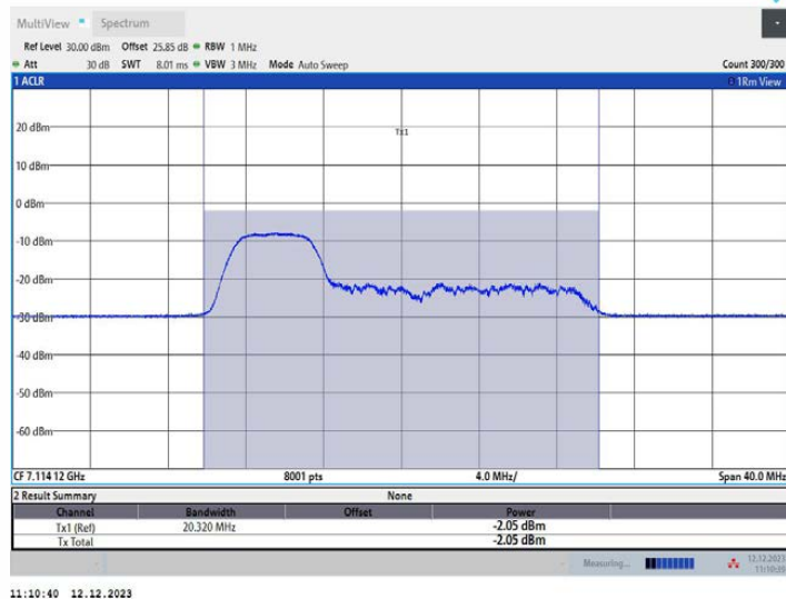
11AX20MIMO_Ant1_7115_106Tone_RU53
