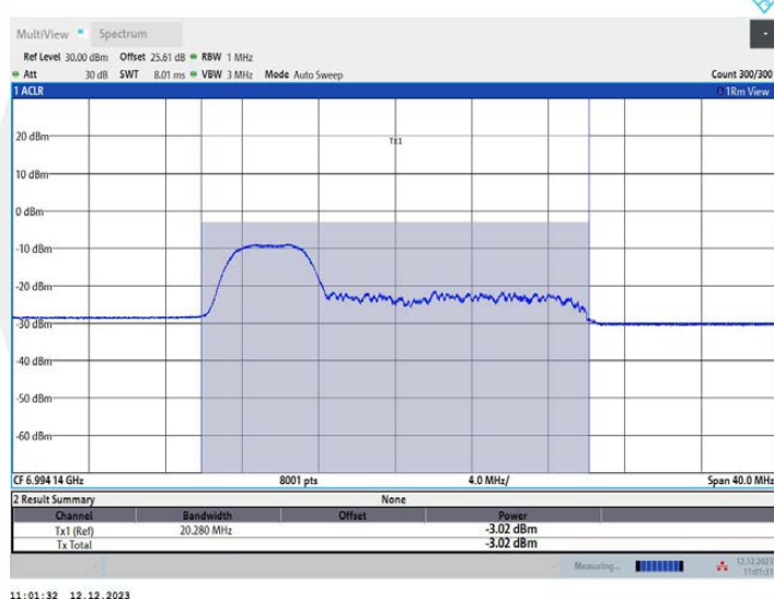
11AX20MIMO_Ant2_6995_106Tone_RU53
