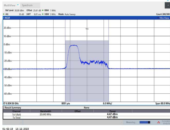
11AX40MIMO_Ant2_6845_106Tone_RU53
