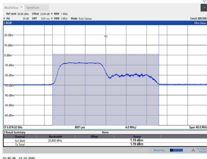
11AX20MIMO_Ant2_6895_26Tone_RU0
