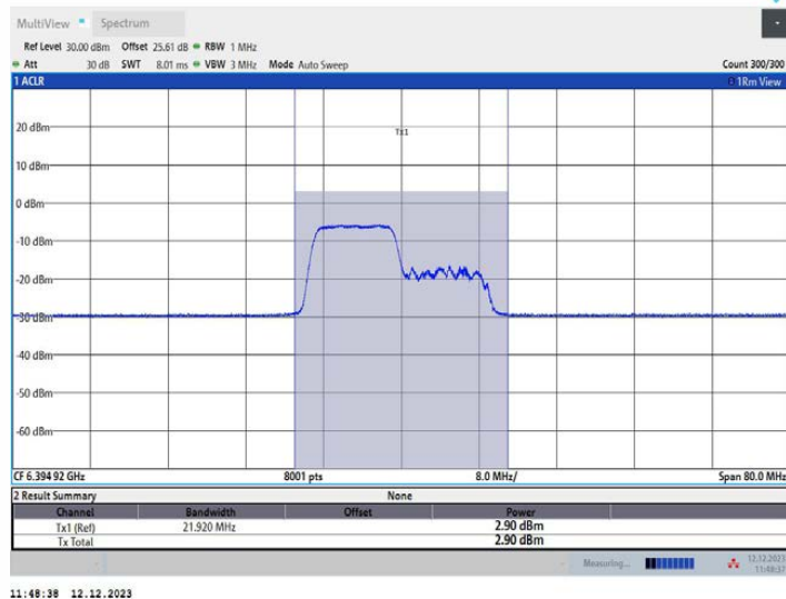
11AX40MIMO_Ant1_6405_242Tone_RU61
