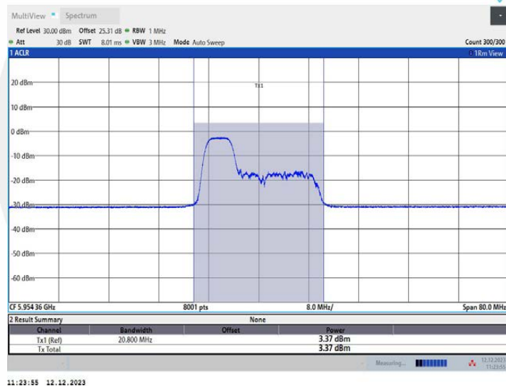
11AX40MIMO_Ant1_5965_106Tone_RU53
