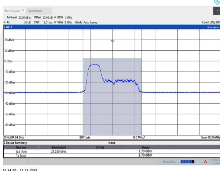
11AX40MIMO_Ant2_6405_106Tone_RU53
