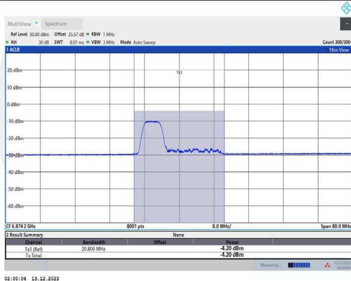
11AX40MIMO_Ant2_6885_106Tone_RU53
