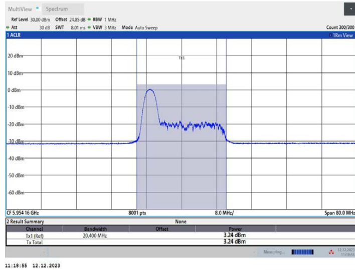
11AX40MIMO_Ant1_5965_52Tone_RU37
