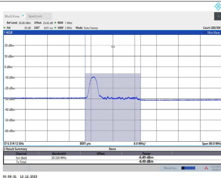
11AX40MIMO_Ant2_6525_52Tone_RU37
