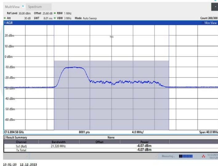
11AX20MIMO_Ant2_6895_106Tone_RU53
