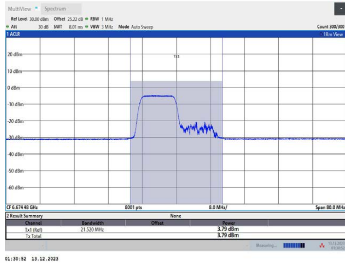
11AX40MIMO_Ant1_6685_242Tone_RU61
