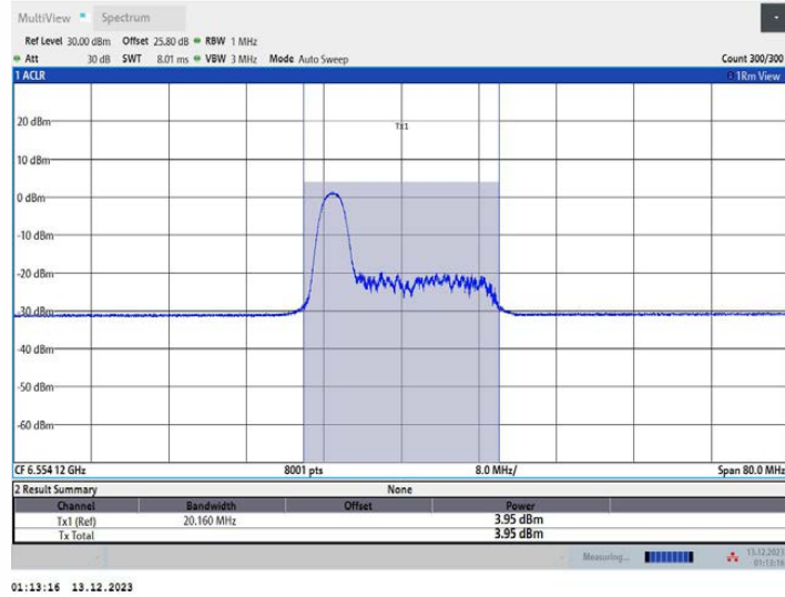
11AX40MIMO_Ant1_6565_52Tone_RU37
