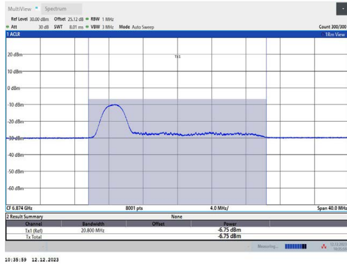
11AX20MIMO_Ant2_6875_52Tone_RU37
