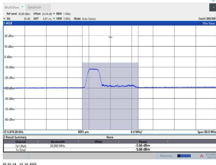
11AX40MIMO_Ant1_6885_106Tone_RU53
