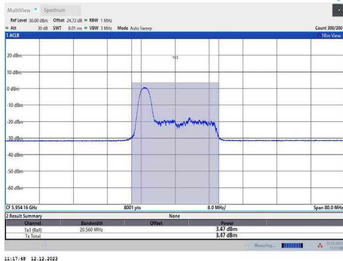
11AX40MIMO_Ant2_5965_52Tone_RU37
