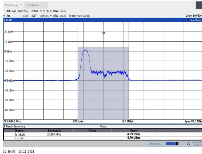
11AX40MIMO_Ant2_6845_52Tone_RU37
