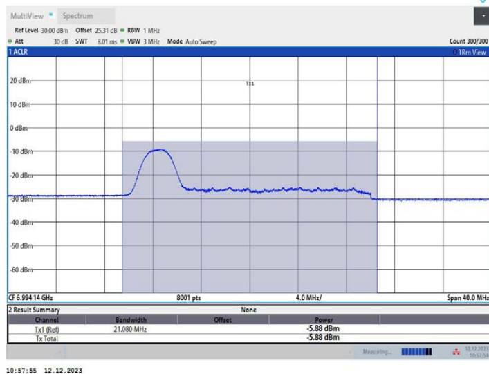
11AX20MIMO_Ant2_6995_52Tone_RU37
