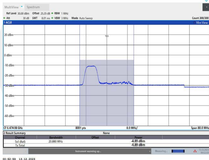
11AX40MIMO_Ant1_6485_106Tone_RU53
