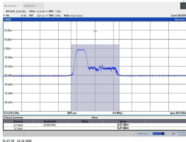
11AX40MIMO_Ant2_6685_106Tone_RU53
