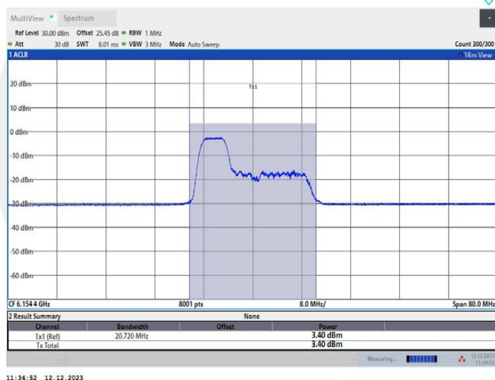
11AX40MIMO_Ant1_6165_106Tone_RU53
