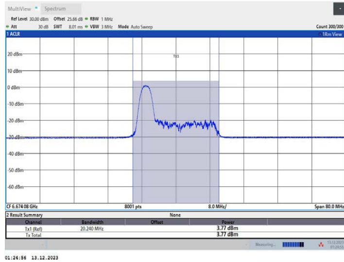
11AX40MIMO_Ant1_6685_52Tone_RU37
