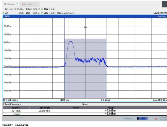
11AX40MIMO_Ant2_6565_52Tone_RU37
