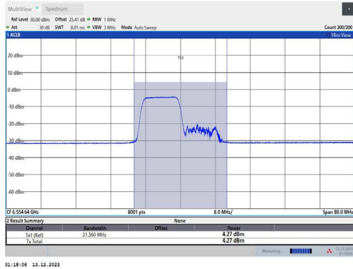
11AX40MIMO_Ant2_6565_242Tone_RU61
