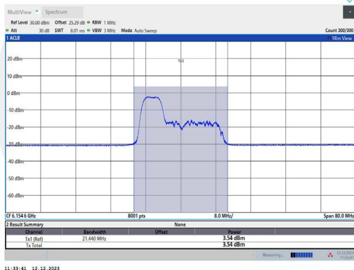
11AX40MIMO_Ant2_6165_106Tone_RU53
