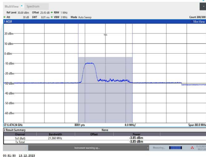
11AX40MIMO_Ant2_6485_106Tone_RU53
