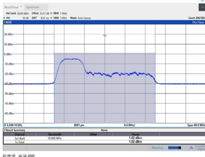
11AX20MIMO_Ant1_6695_106Tone_RU53
