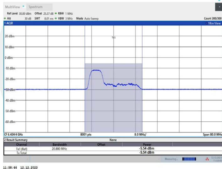
11AX40MIMO_Ant1_6445_106Tone_RU53
