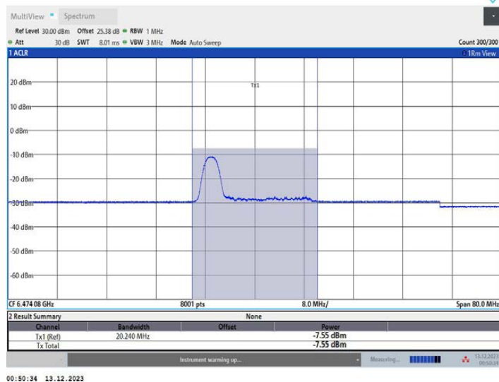
11AX40MIMO_Ant1_6485_52Tone_RU37
