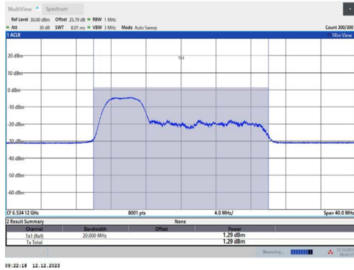
11AX20MIMO_Ant1_6535_106Tone_RU53
