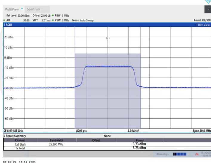
11AX40MIMO_Ant1_6925_26Tone_RU0
