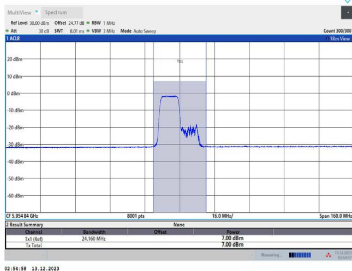
11AX80MIMO_Ant2_5985_242Tone_RU61
