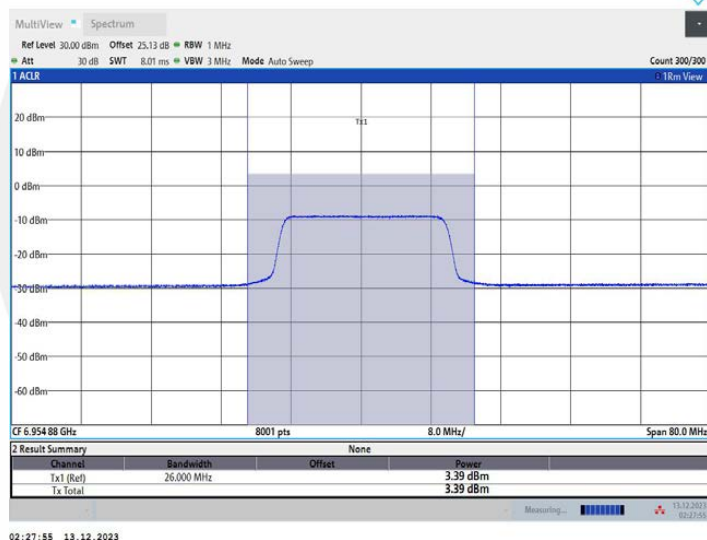
11AX40MIMO_Ant1_6965_26Tone_RU0
