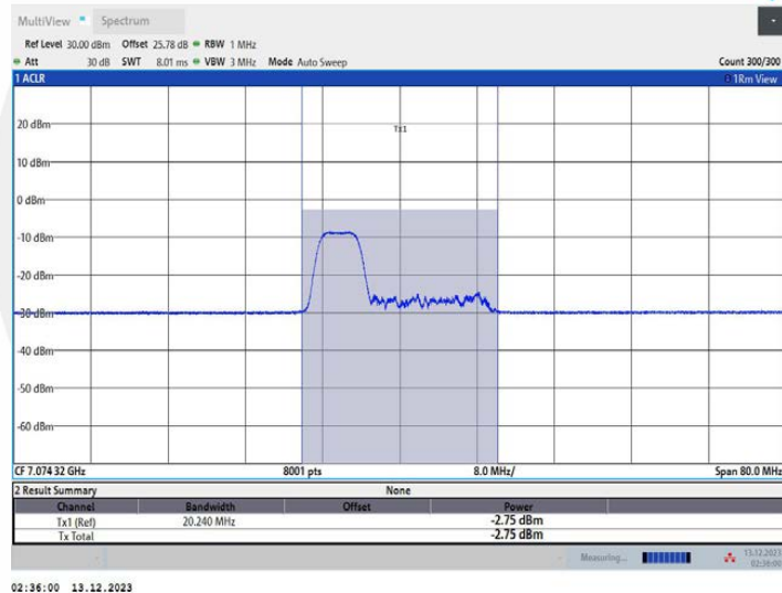
11AX40MIMO_Ant1_7085_106Tone_RU53
