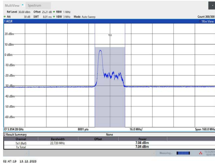
11AX80MIMO_Ant2_5985_52Tone_RU37
