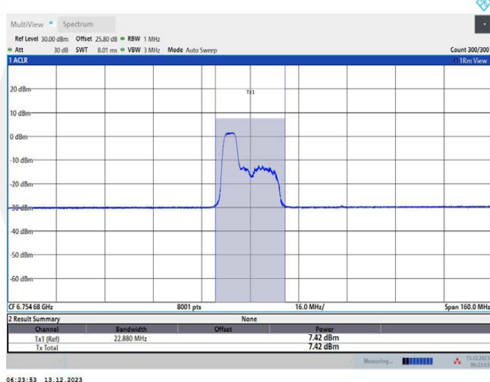
11AX80MIMO_Ant2_6785_106Tone_RU53
