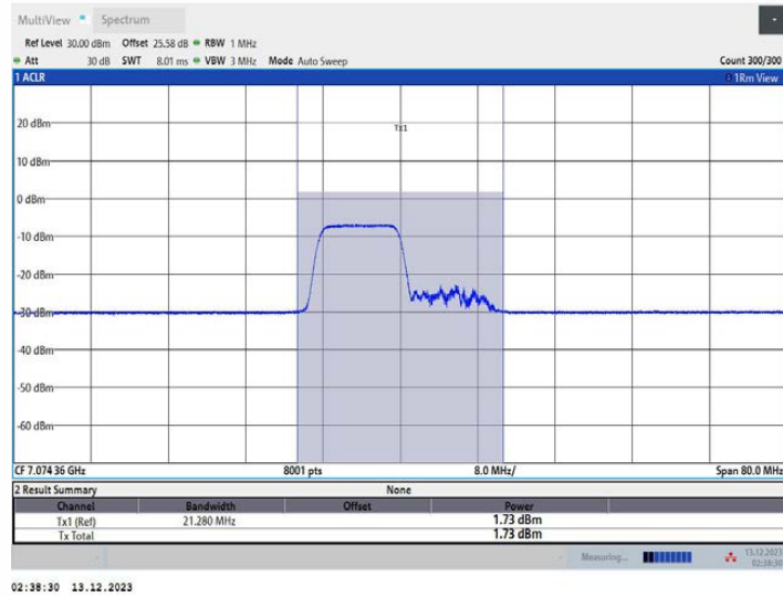
11AX40MIMO_Ant2_7085_242Tone_RU61
