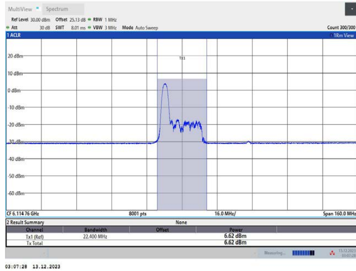
11AX80MIMO_Ant2_6145_52Tone_RU37
