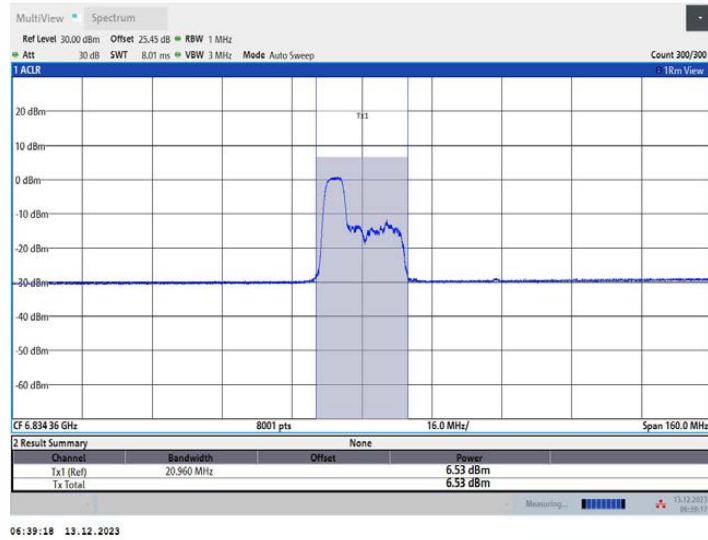
11AX80MIMO_Ant1_6865_106Tone_RU53
