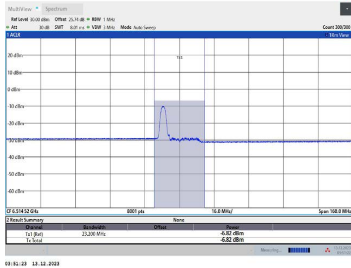
11AX80MIMO_Ant2_6545_52Tone_RU37
