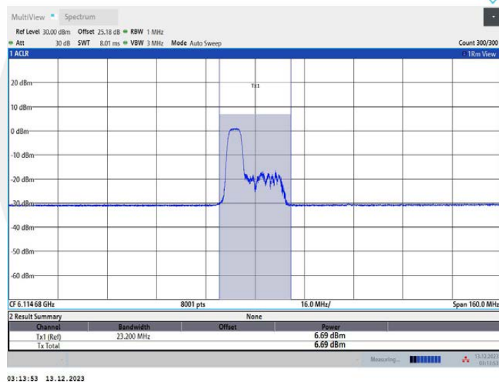
11AX80MIMO_Ant2_6145_106Tone_RU53
