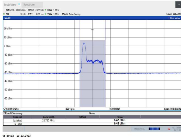
11AX80MIMO_Ant2_6625_52Tone_RU37
