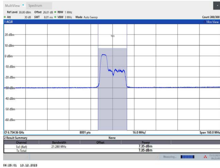
11AX80MIMO_Ant1_6785_106Tone_RU53
