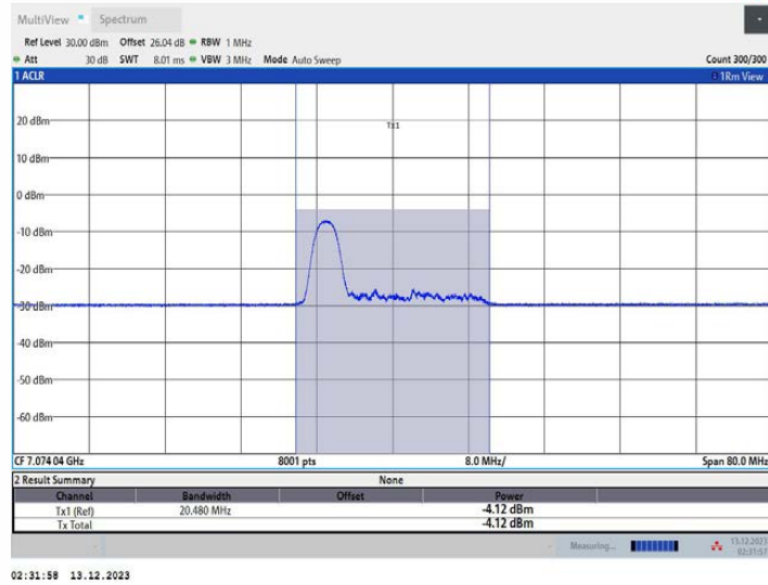
11AX40MIMO_Ant2_7085_52Tone_RU37
