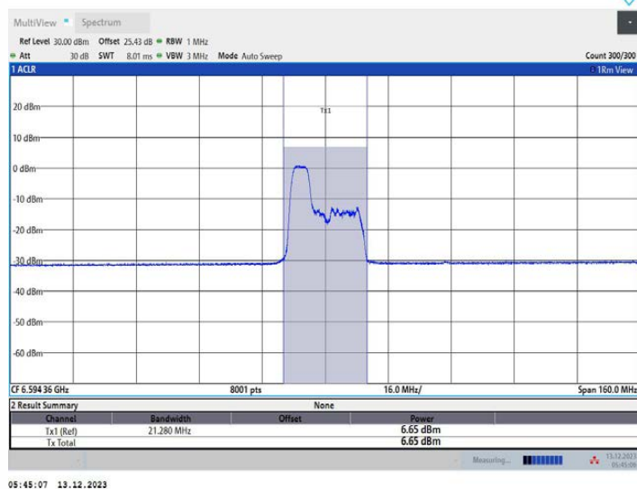
11AX80MIMO_Ant1_6625_106Tone_RU53
