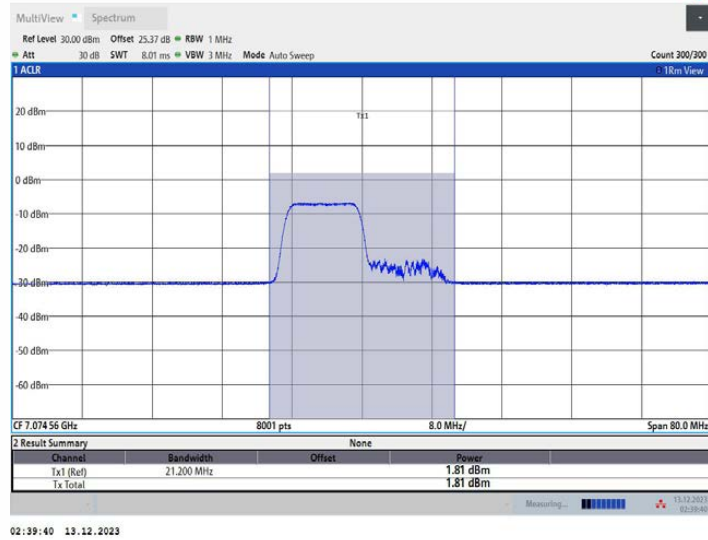
11AX40MIMO_Ant1_7085_242Tone_RU61
