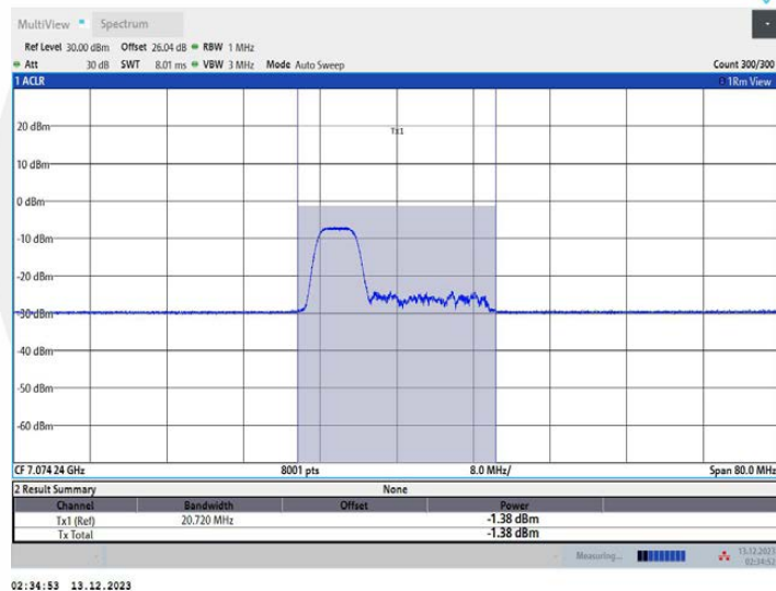
11AX40MIMO_Ant2_7085_106Tone_RU53
