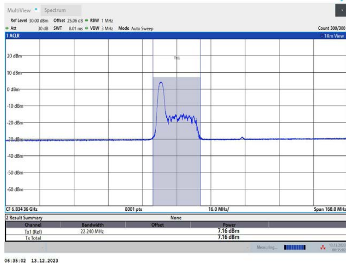
11AX80MIMO_Ant2_6865_52Tone_RU37
