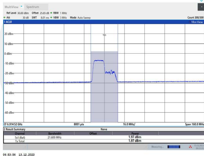
11AX80MIMO_Ant1_6945_242Tone_RU61
