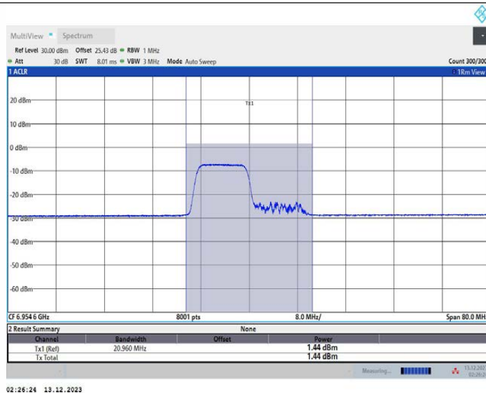
11AX40MIMO_Ant1_6965_242Tone_RU61
