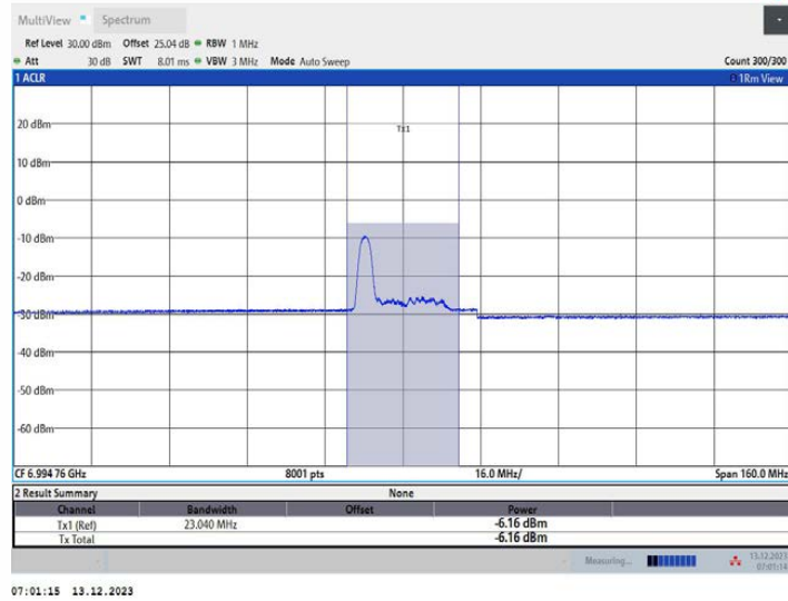
11AX80MIMO_Ant2_7025_52Tone_RU37
