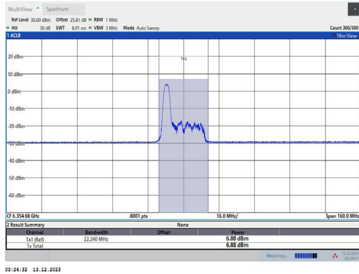
11AX80MIMO_Ant2_6385_52Tone_RU37
