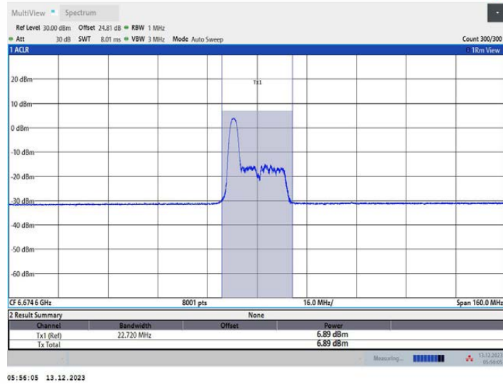
11AX80MIMO_Ant2_6705_52Tone_RU37
