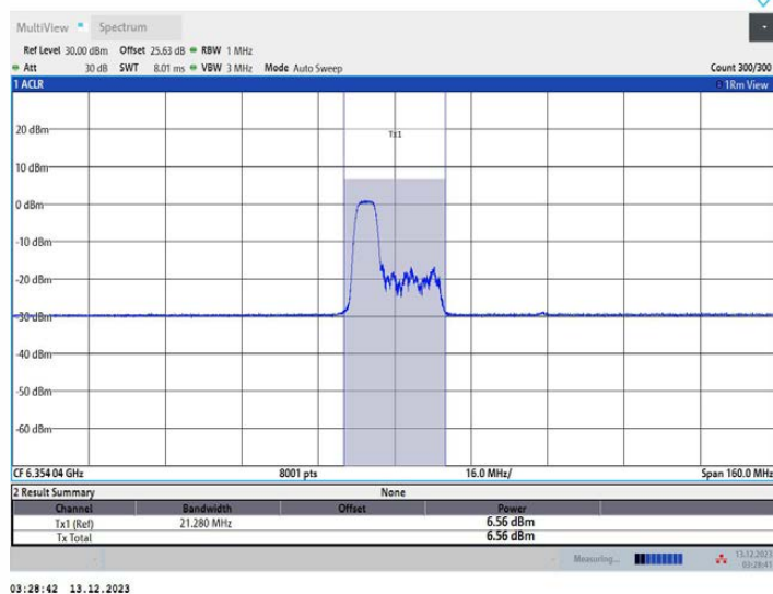
11AX80MIMO_Ant1_6385_106Tone_RU53
