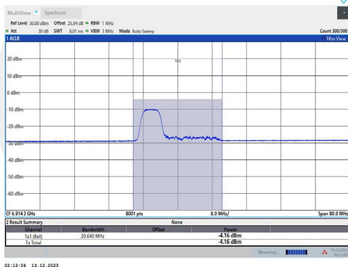
11AX40MIMO_Ant1_6925_106Tone_RU53
