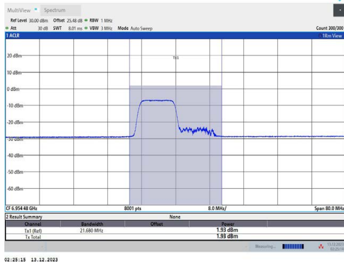
11AX40MIMO_Ant2_6965_242Tone_RU61
