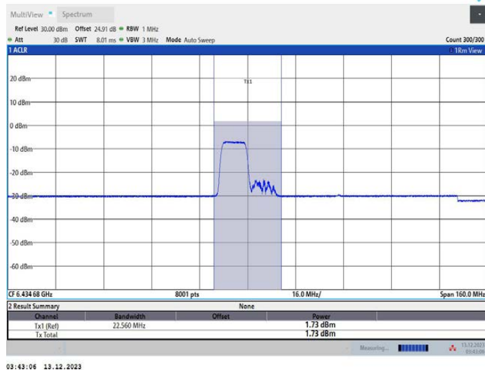
11AX80MIMO_Ant2_6465_242Tone_RU61
