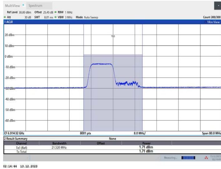
11AX40MIMO_Ant1_6925_242Tone_RU61
