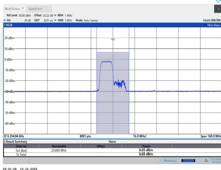
11AX80MIMO_Ant1_6385_242Tone_RU61
